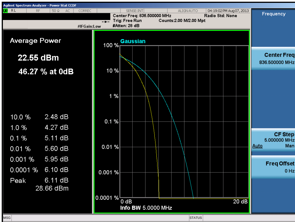
Plot 8-5. PAR Plot (5.0MHz QPSK – RB Size 25)
