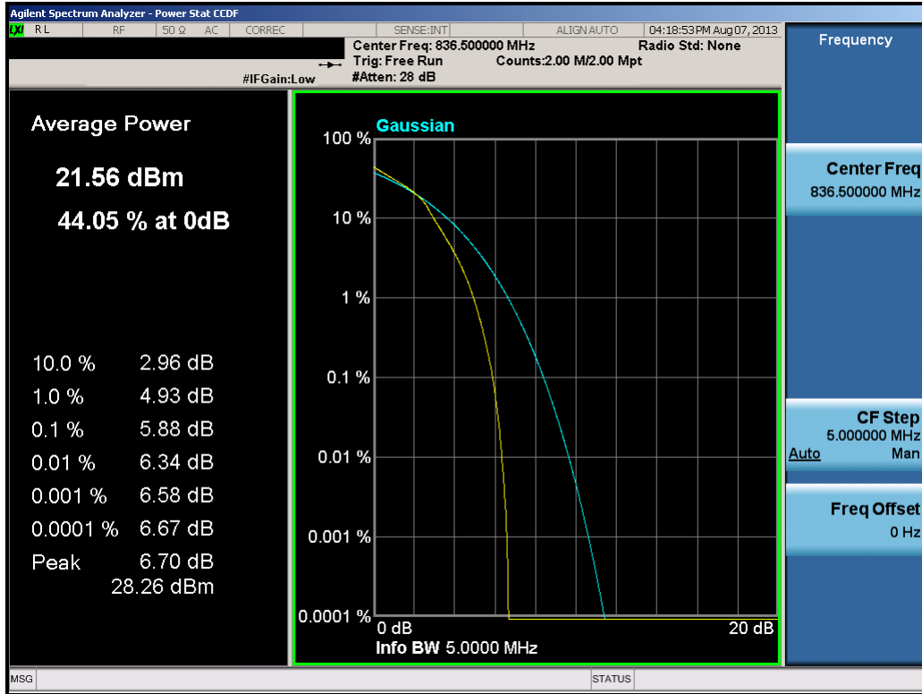
Plot 8-6. PAR Plot (5.0MHz 16-QAM – RB Size 25)
