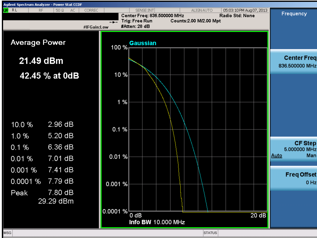
Plot 8-18. PAR Plot (10.0MHz 16-QAM – RB Size 50)
