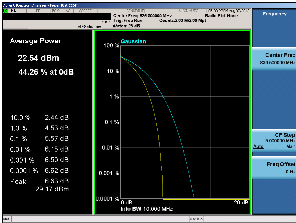
Plot 8-17. PAR Plot (10.0MHz QPSK – RB Size 50)
