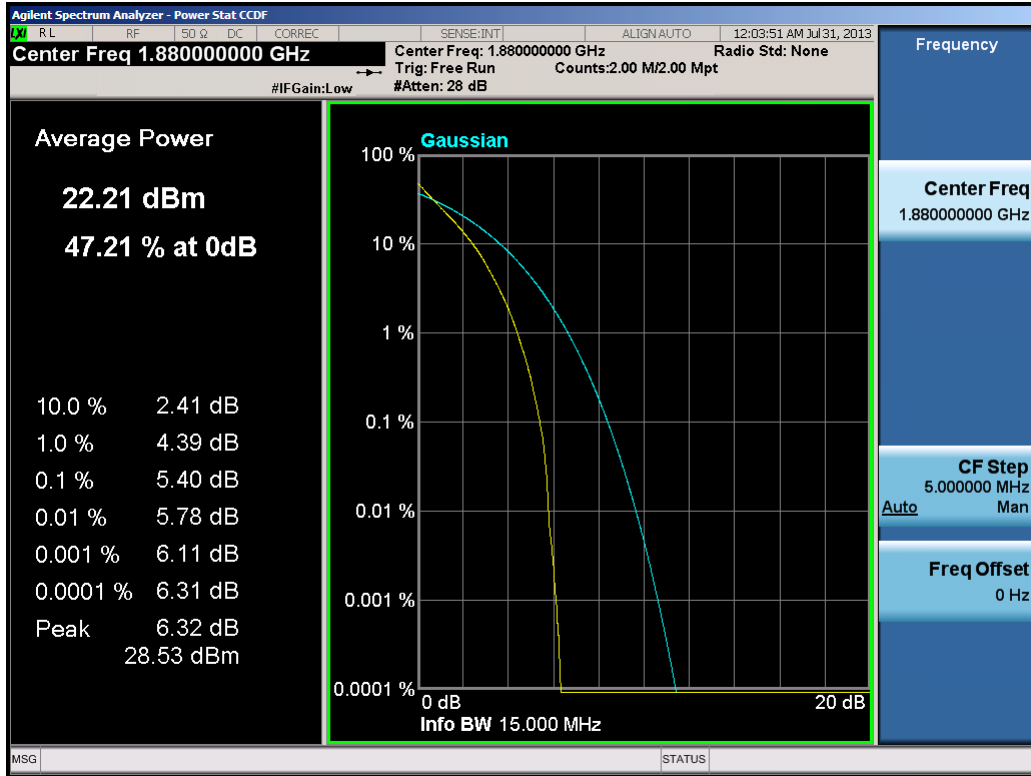
Plot 10-23. PAR Plot (15.0MHz QPSK – RB Size 75)
