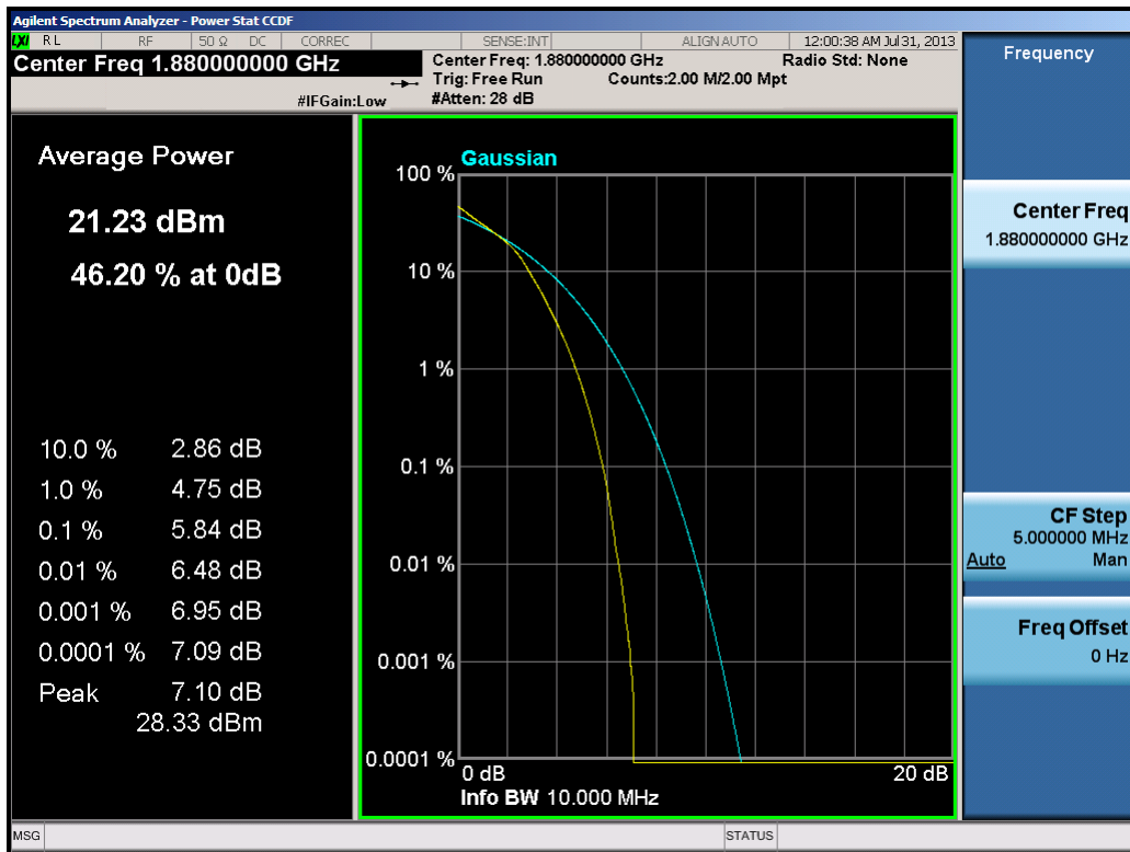
Plot 10-16. PAR Plot (10.0MHz 16-QAM – RB Size 50)
