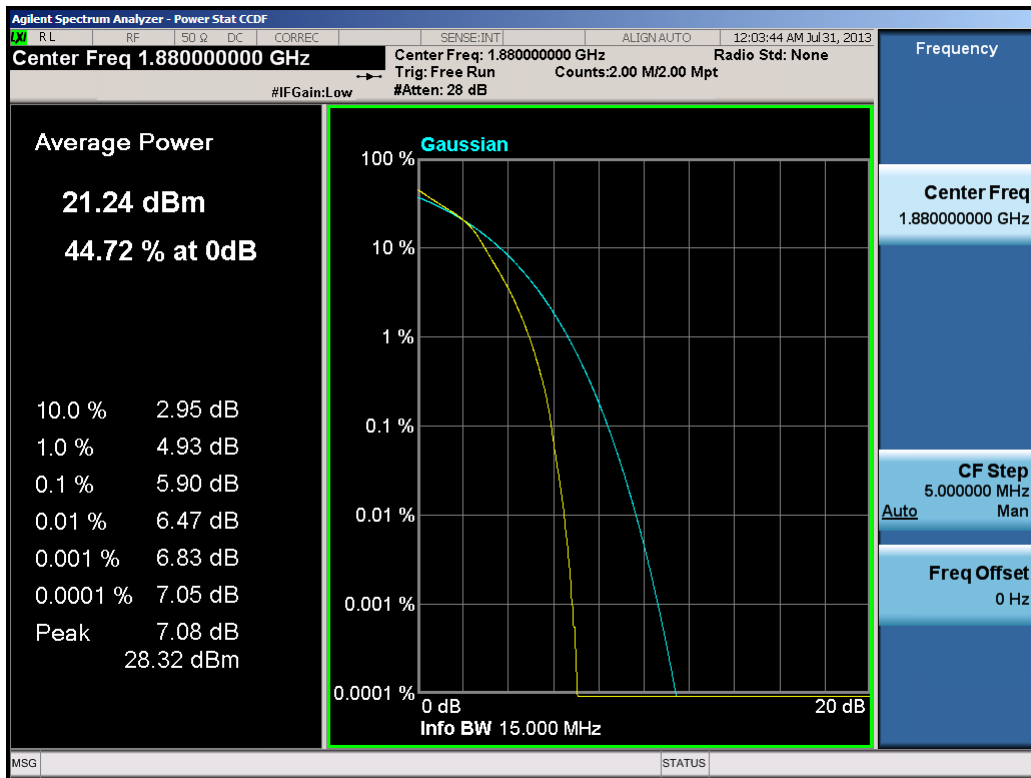
Plot 10-24. PAR Plot (15.0MHz 16-QAM – RB Size 75)
