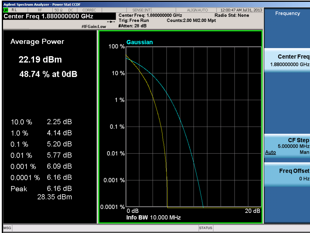
Plot 10-15. PAR Plot (10.0MHz QPSK – RB Size 50)
