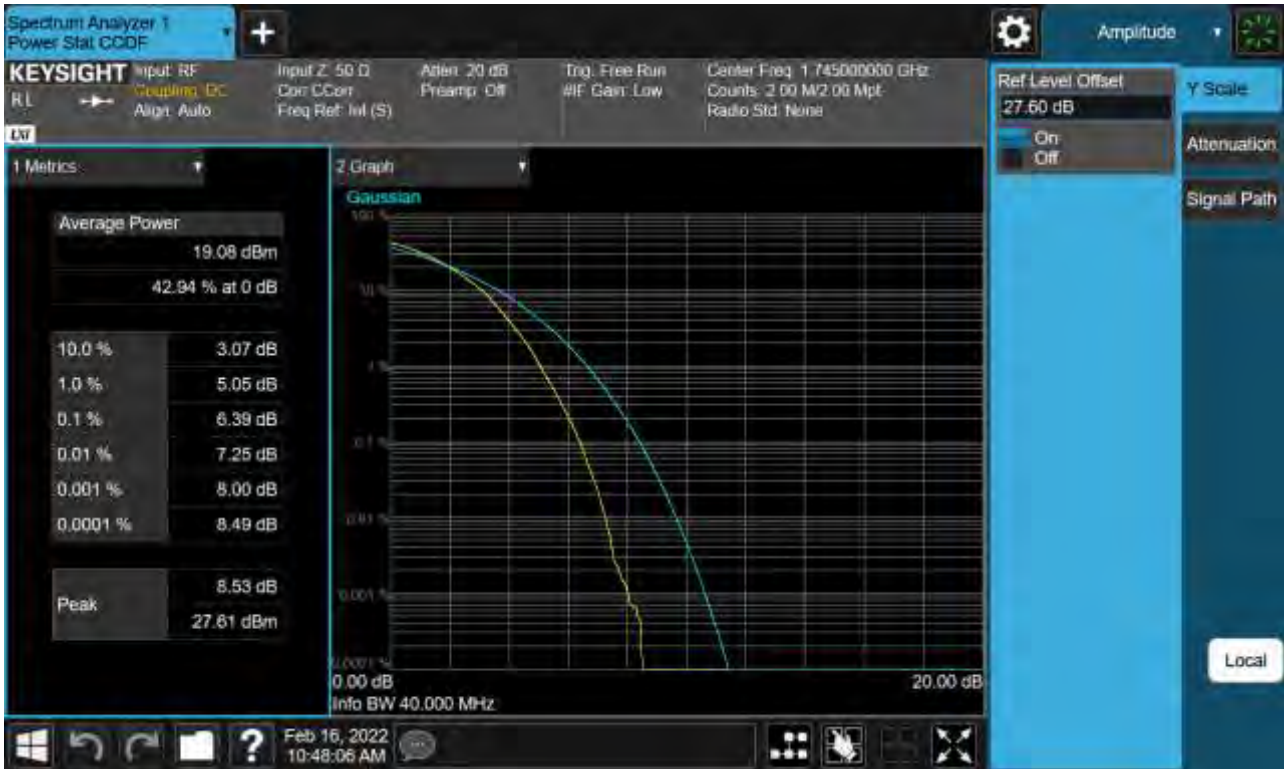
Sub6 n66. PAR Plot (40 M BW_Ch.349000_256QAM_Full RB)
