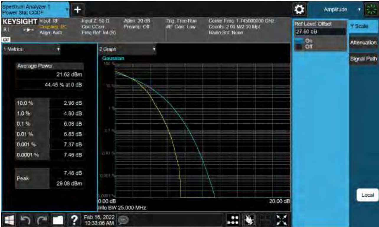
Sub6 n66. PAR Plot (25 M BW_Ch.349000_16QAM_Full RB)
