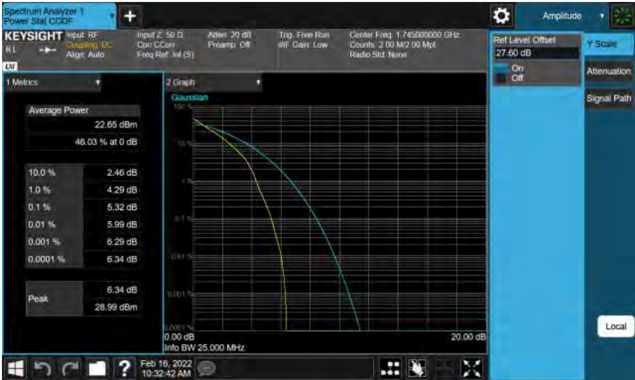
Sub6 n66. PAR Plot (25 M BW_Ch.349000_QPSK_Full RB)
