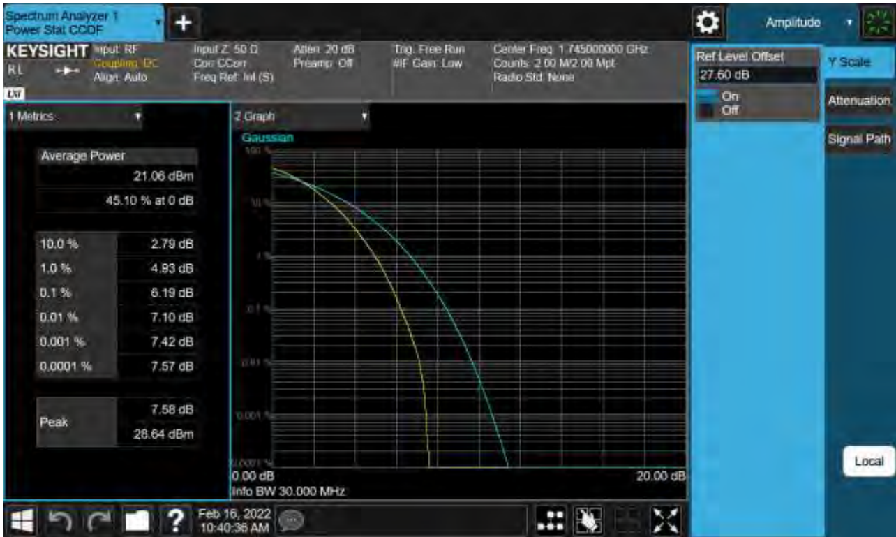
Sub6 n66. PAR Plot (30 M BW_Ch.349000_64QAM_Full RB)
