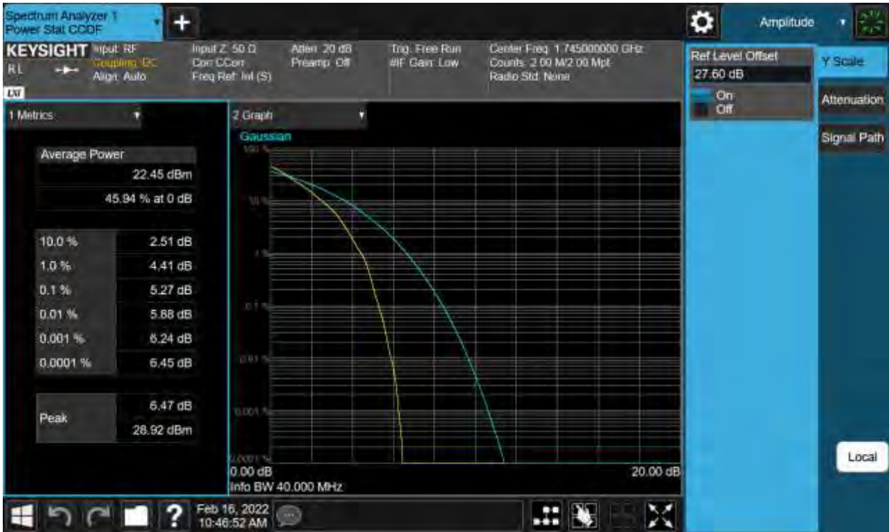
Sub6 n66. PAR Plot (40 M BW_Ch.349000_QPSK_Full RB)
