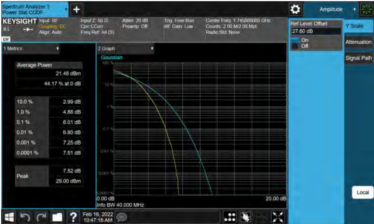
Sub6 n66. PAR Plot (40 M BW_Ch.349000_16QAM_Full RB)
