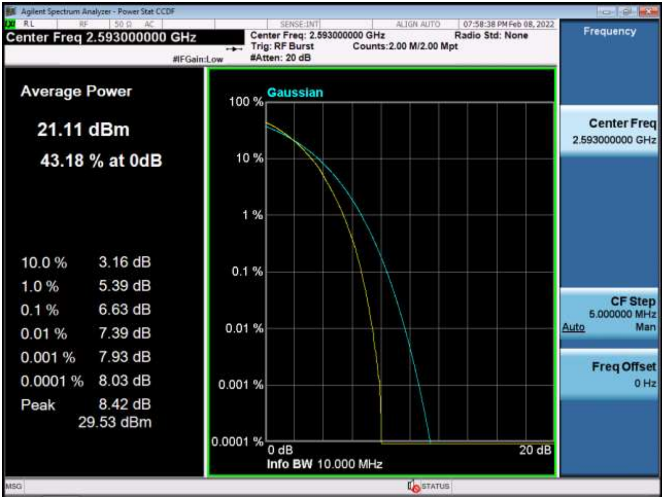
PAR Plot (10 M BW_Ch.40620_64QAM_RB50_0)
