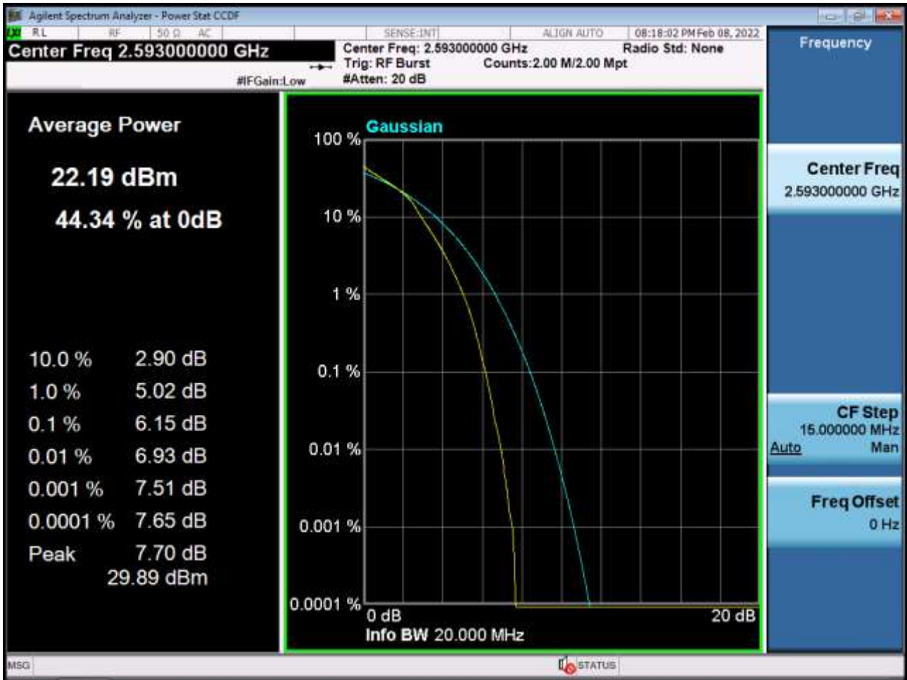
PAR Plot (20 M BW_Ch.40620_16QAM_RB100_0)
