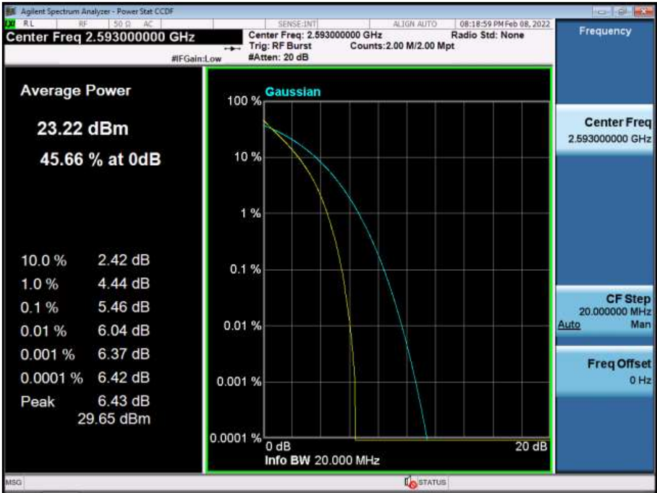
PAR Plot (20 M BW_Ch.40620_QPSK_RB100_0)
