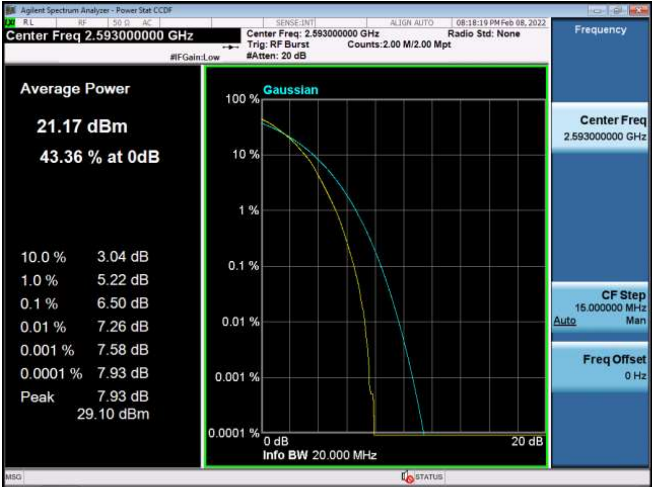
PAR Plot (20 M BW_Ch.40620_64QAM_RB100_0)
