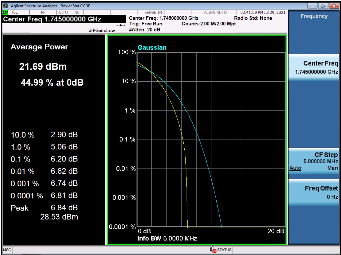
Sub6 n66. PAR Plot (5 M BW_Ch.349000_64QAM_RB25_0)
