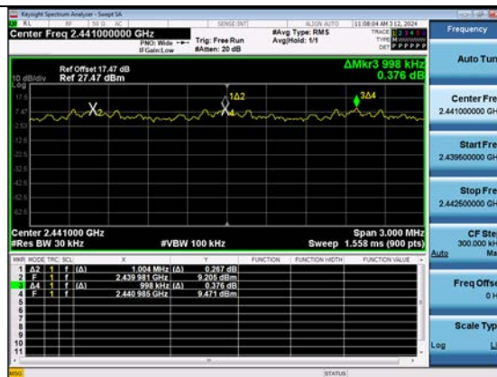
Test Plot ( \pi/4 DQPSK)
