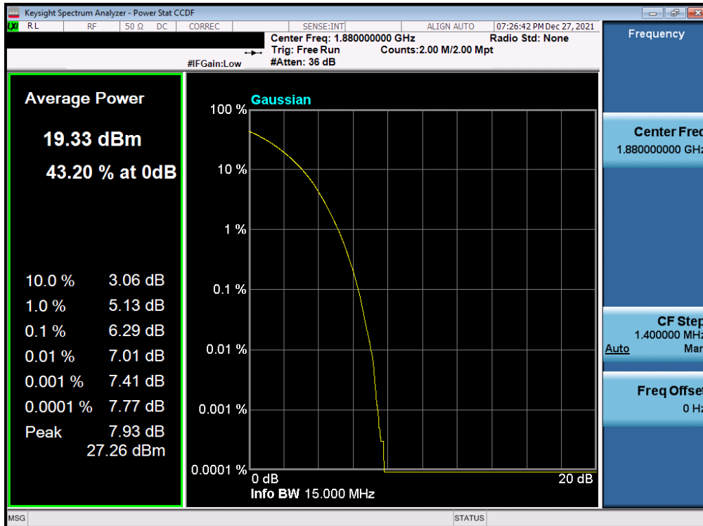
Plot 7-76. PAR Plot (LTE Band 2 - 15MHz 256-QAM - Full RB)
