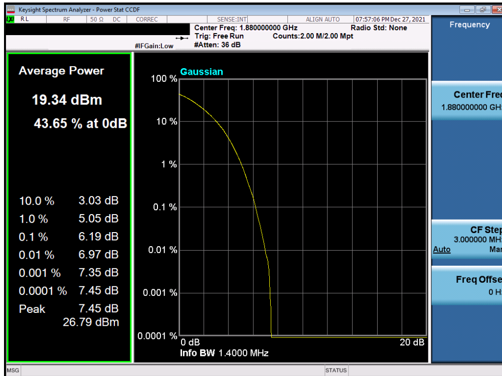
Plot 7-84. PAR Plot (LTE Band 2 - 1.4MHz 256-QAM - Full RB)
