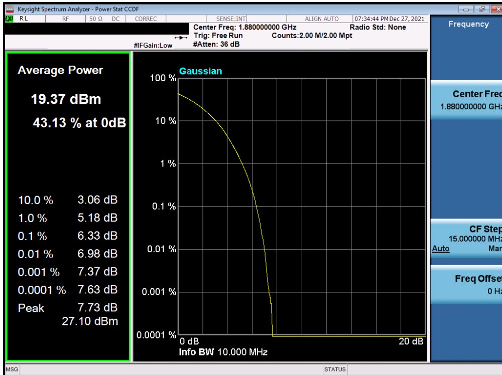
Plot 7-78. PAR Plot (LTE Band 2 - 10MHz 256-QAM - Full RB)
