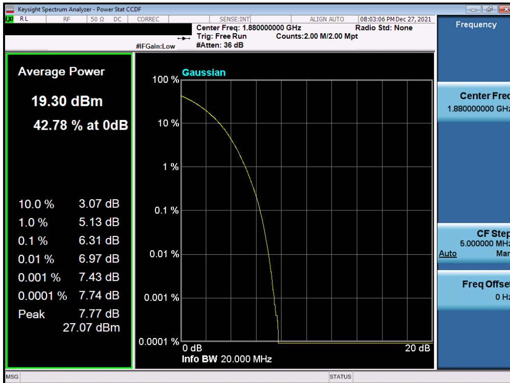
Plot 7-74. PAR Plot (LTE Band 2 - 20MHz 256-QAM - Full RB)
