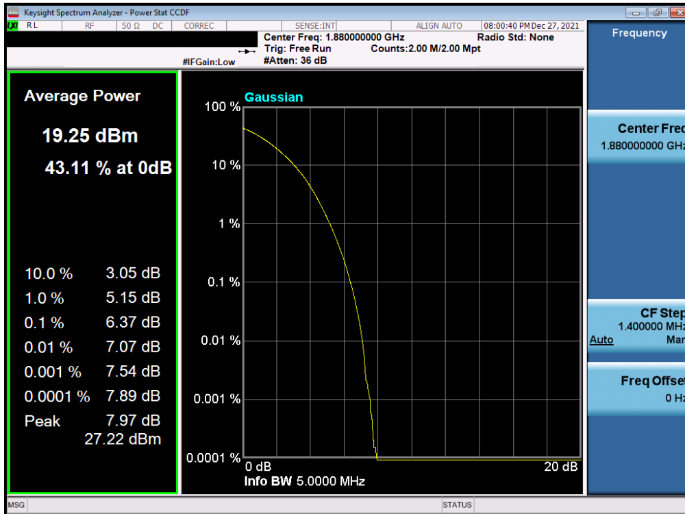
Plot 7-80. PAR Plot (LTE Band 2 - 5MHz 256-QAM - Full RB)
