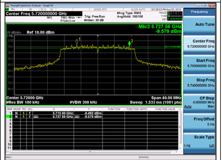
802.11n_HT20 CH.144
