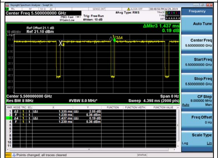
802.11ac(VHT20)
