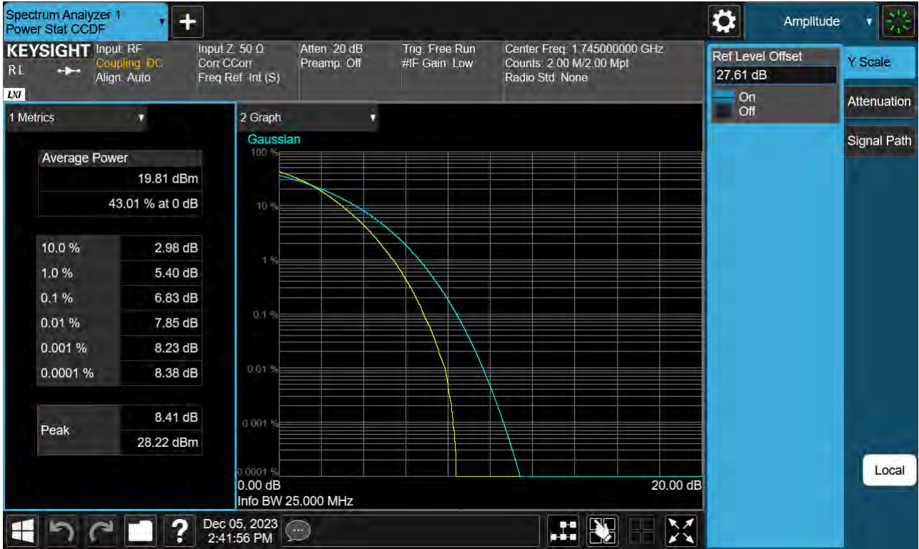
Sub6 n66. PAR Plot (25 M BW_Ch.349000_256QAM_Full RB)
