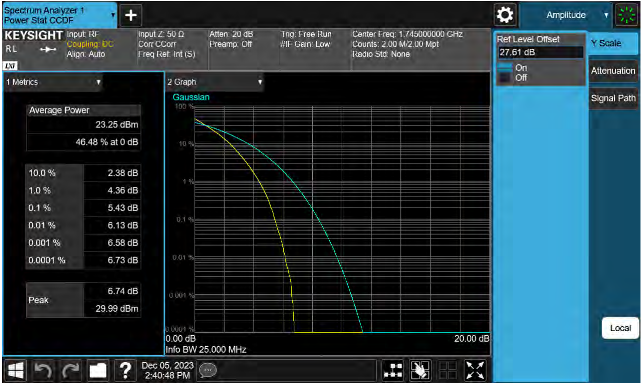
Sub6 n66. PAR Plot (25 M BW_Ch.349000_QPSK_Full RB)
