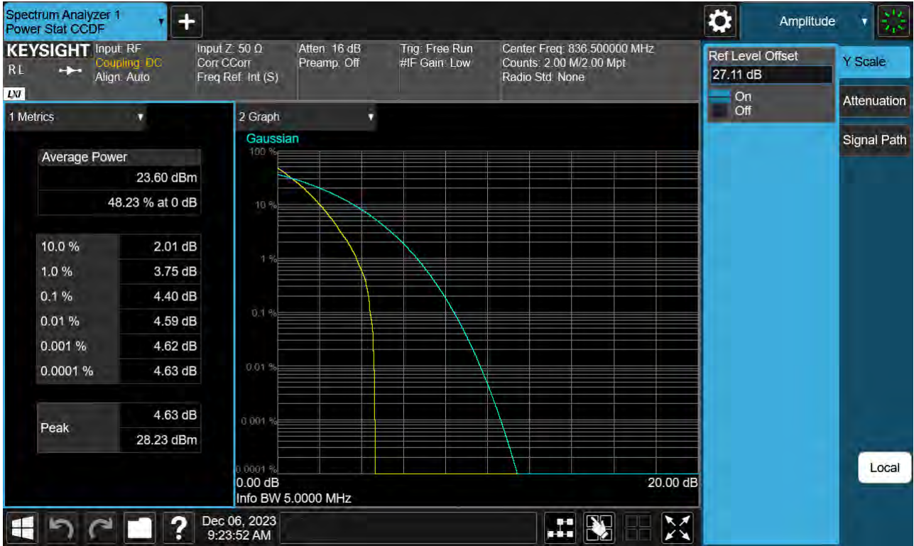
Sub6 n5. PAR Plot (5 M BW_Ch.167300_BPSK_Full RB_0)
