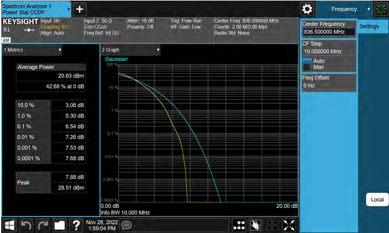
Sub6 n5. PAR Plot (10 M BW_Ch. 167300_256QAM_Full RB _0)
