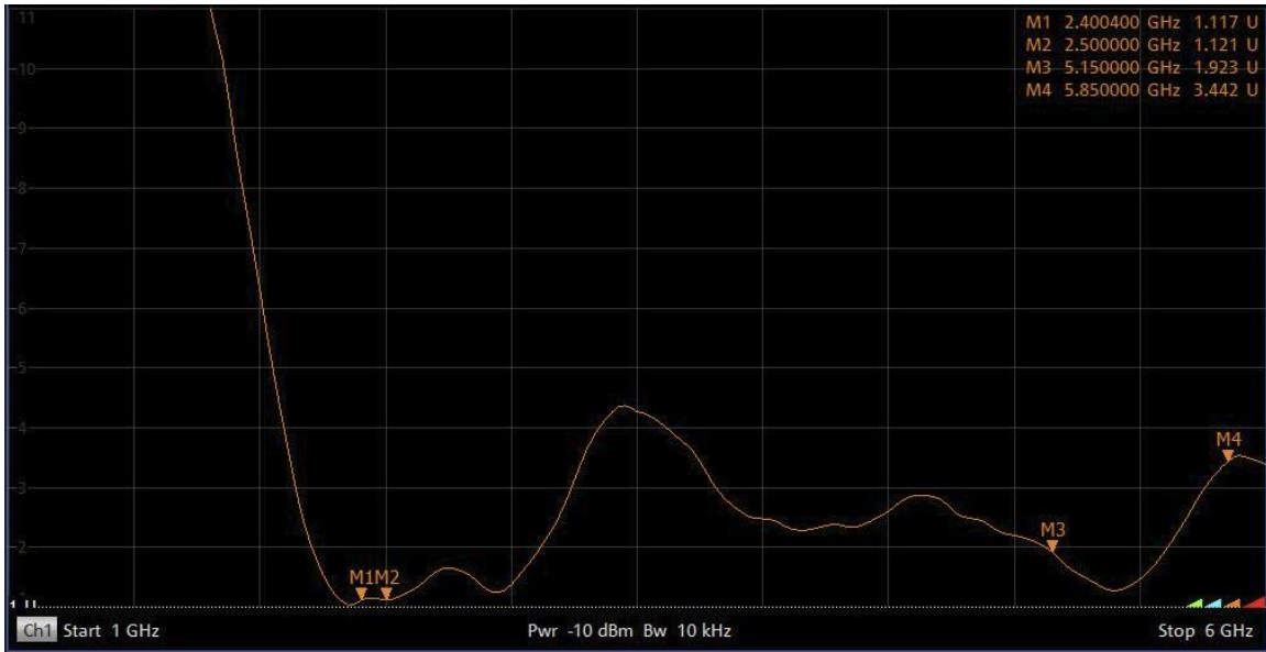
BT/WiFi Antenna
