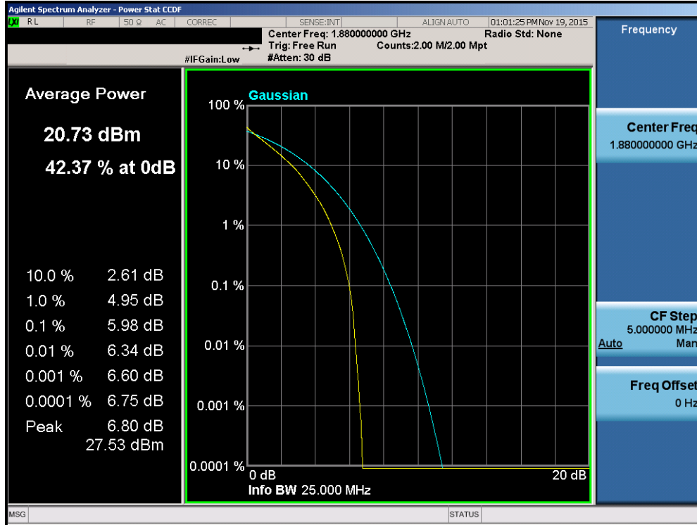
Plot 7-155. PAR Plot (Band 2 – 15.0MHz QPSK – RB Size 75)
