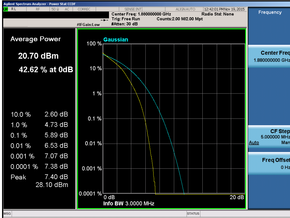
Plot 7-149. PAR Plot (Band 2 – 3.0MHz QPSK – RB Size 15)
