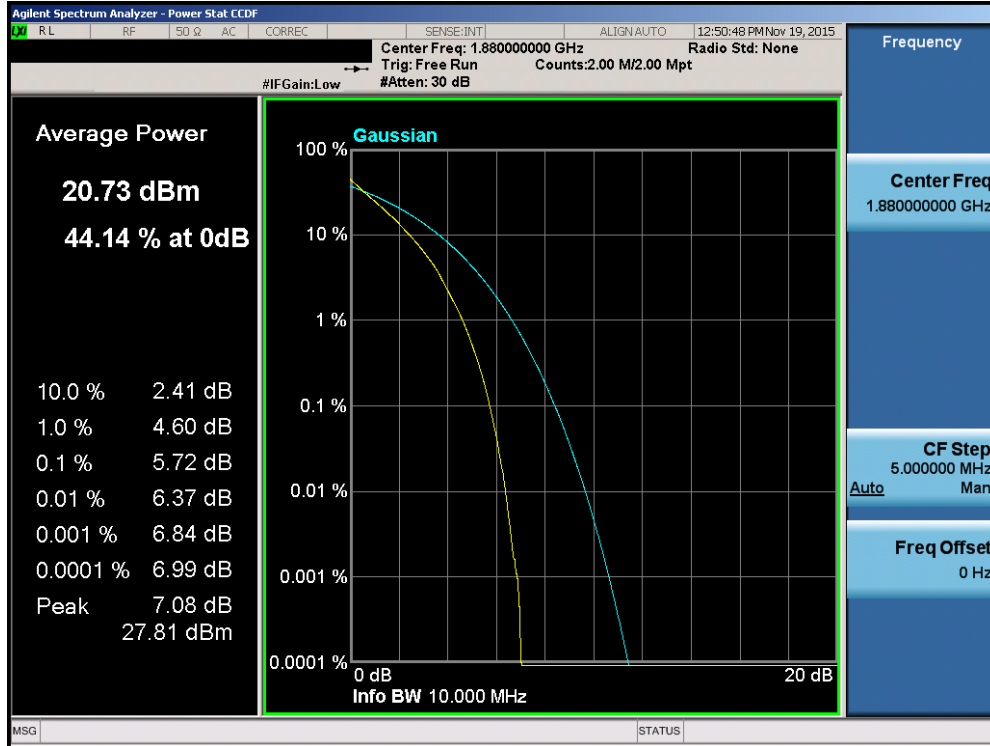
Plot 7-153. PAR Plot (Band 2 – 10.0MHz QPSK – RB Size 50)
