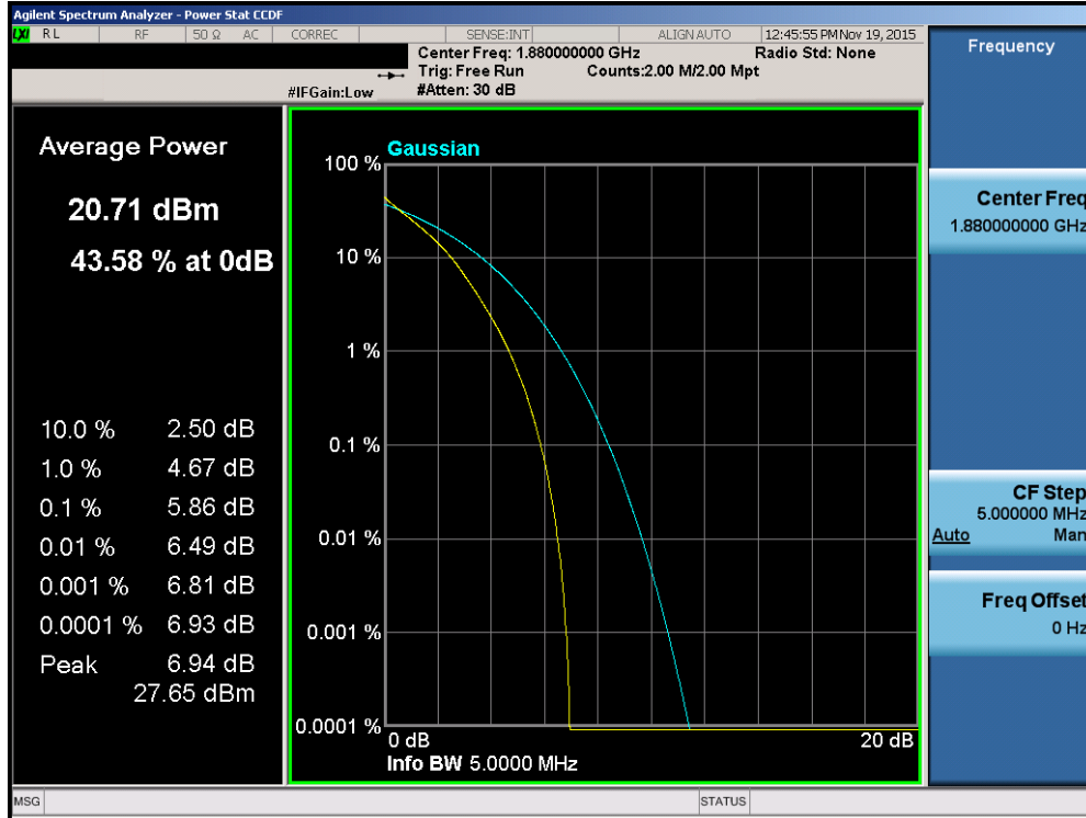
Plot 7-151. PAR Plot (Band 2 – 5.0MHz QPSK – RB Size 25)
