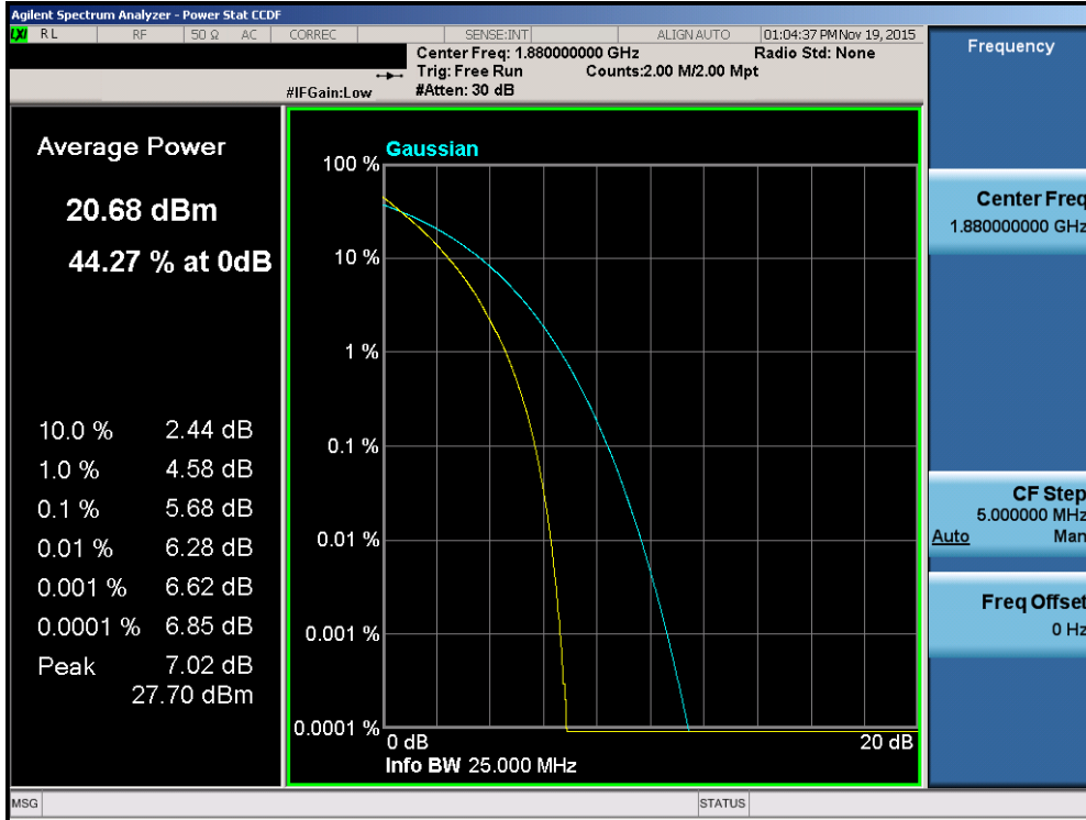
Plot 7-157. PAR Plot (Band 2 – 20.0MHz QPSK – RB Size 100)
