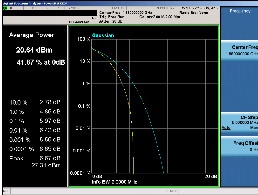
Plot 7-147. PAR Plot (Band 2 – 1.4MHz QPSK – RB Size 6)
