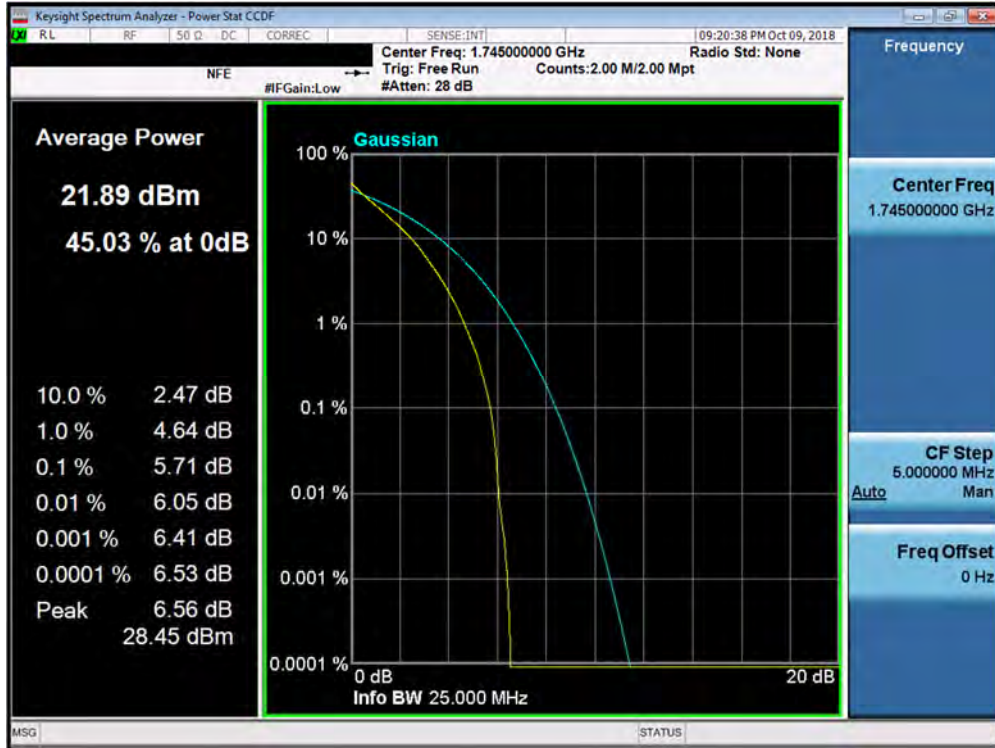
Plot 7-211. PAR Plot (Band 66/4 - 15.0MHz QPSK - Full RB Configuration)
