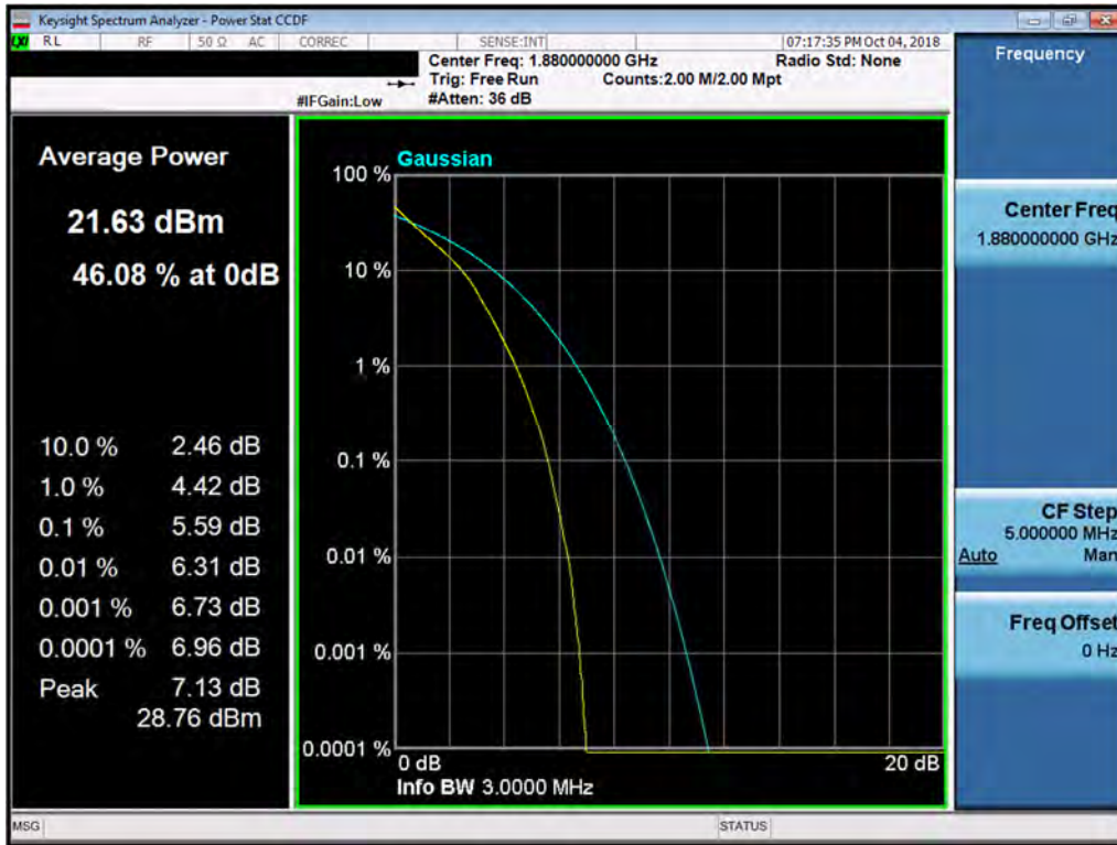
Plot 7-217. PAR Plot (Band 2 - 3.0MHz QPSK - Full RB Configuration)
