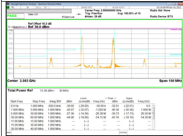
LTE B41 10MHz + 20MHz QPSK Mid Ch RB1-0 + RB1-99
