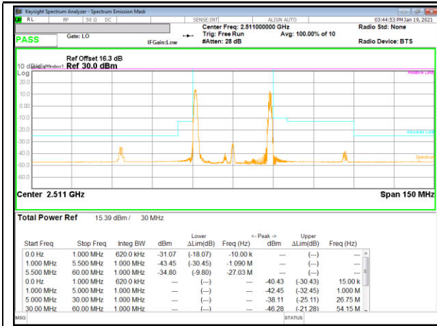
LTE B41 20MHz + 10MHz QPSK Low Ch RB1-0 + RB1-49
