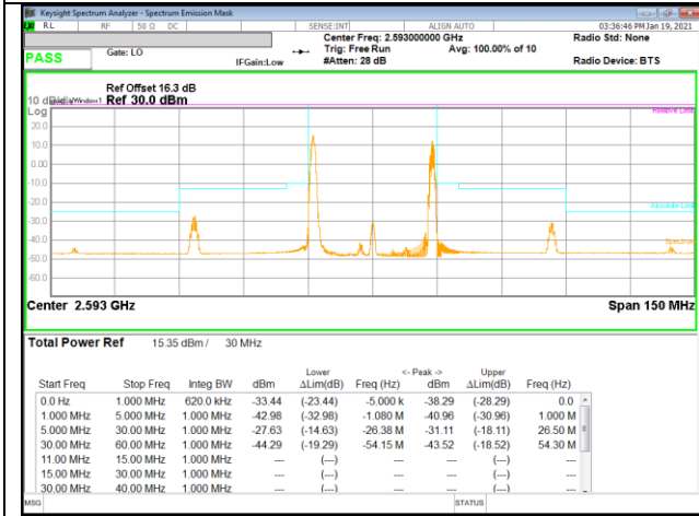
LTE B41 20MHz + 10MHz QPSK Mid Ch RB1-0 + RB1-49
