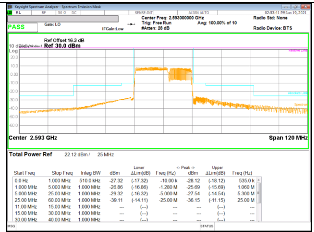
LTE B41 15MHz + 10MHz QPSK Mid Ch RB75-0 + RB50-0
