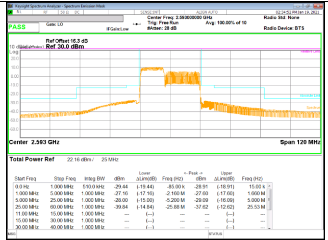
LTE B41 10MHz + 15MHz QPSK Mid Ch RB50-0 + RB75-0
