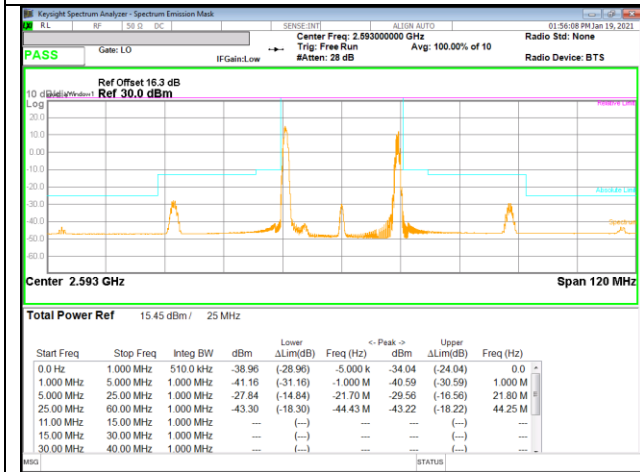
LTE B41 5MHz + 20MHz QPSK Mid Ch RB1-0 + RB1-99
