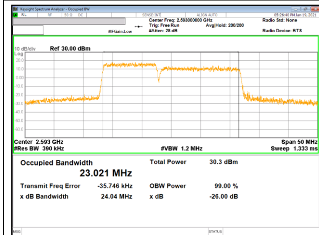
LTE B41 10MHz + 15MHz QPSK RB50-0 + RB75-0
