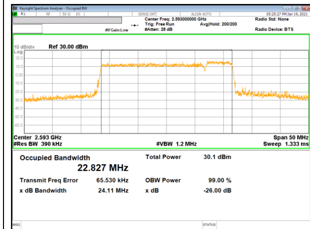
LTE B41 20MHz + 5MHz QPSK RB100-0 + RB25-0
