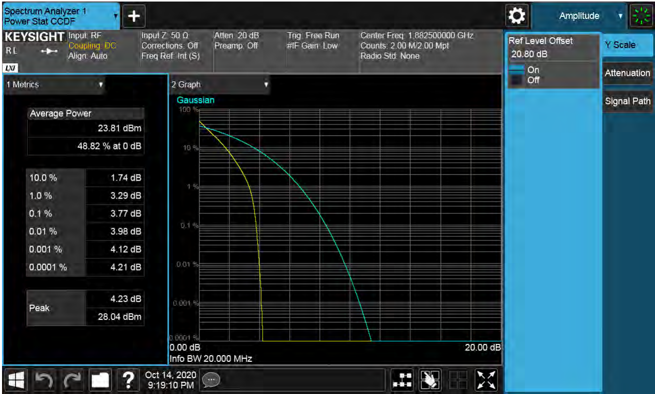
Sub6 n25(2). PAR Plot (20M BW Ch.376500 BPSK RB 100_0)
