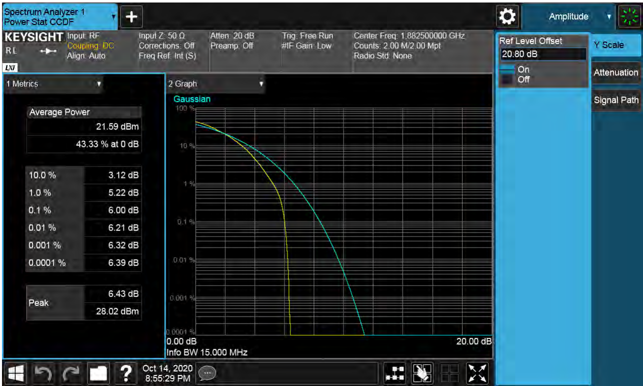
Sub6 n25(2). PAR Plot (15M BW Ch.376500 64QAM RB 75_0)
