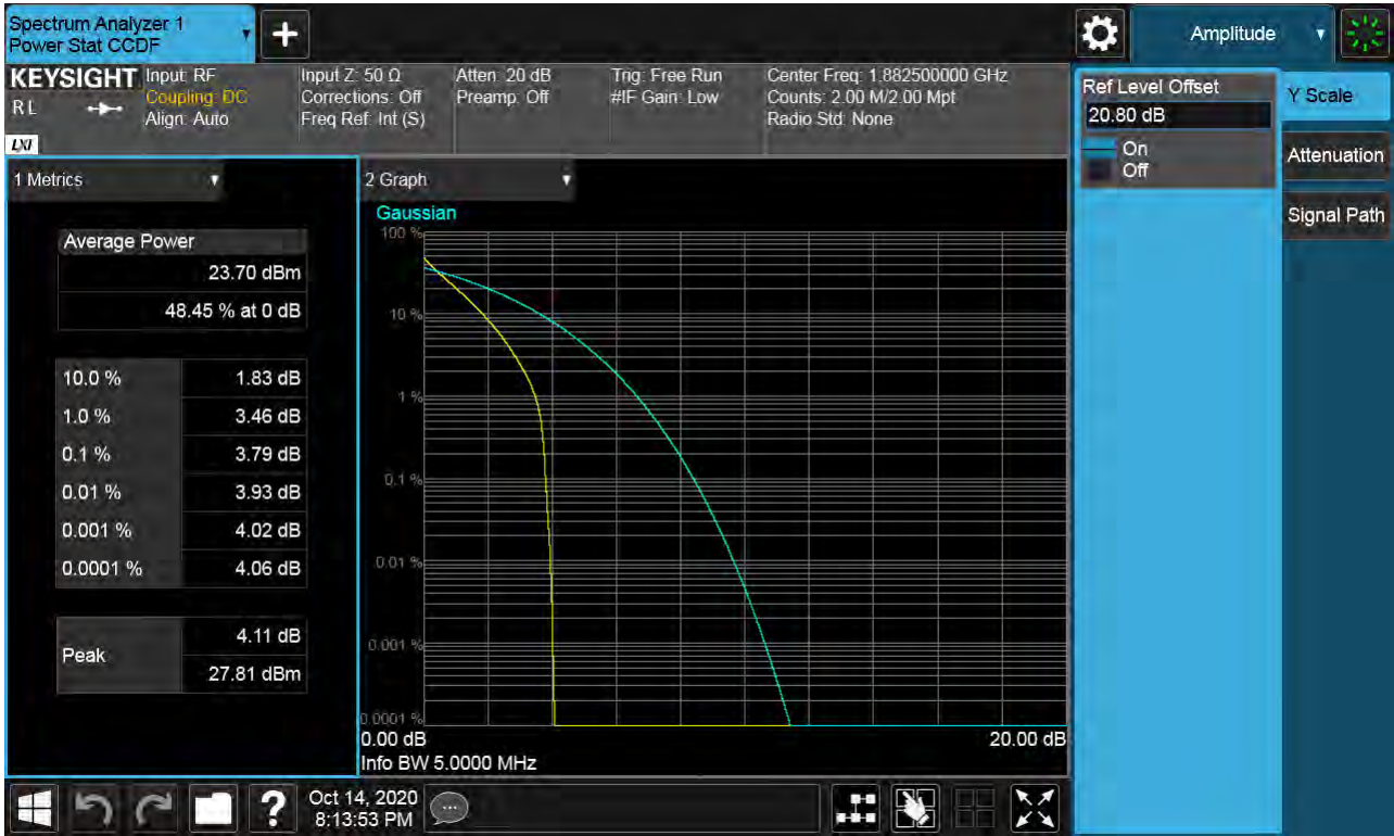
Sub6 n25(2). PAR Plot (5M BW Ch.376500 BPSK )
