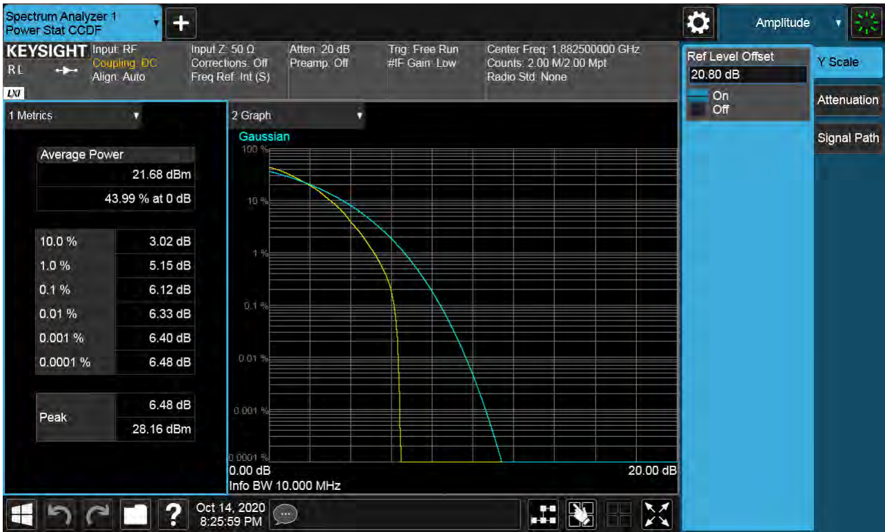
Sub6 n25(2). PAR Plot (10M BW Ch.376500 64QAM RB 50_0)
