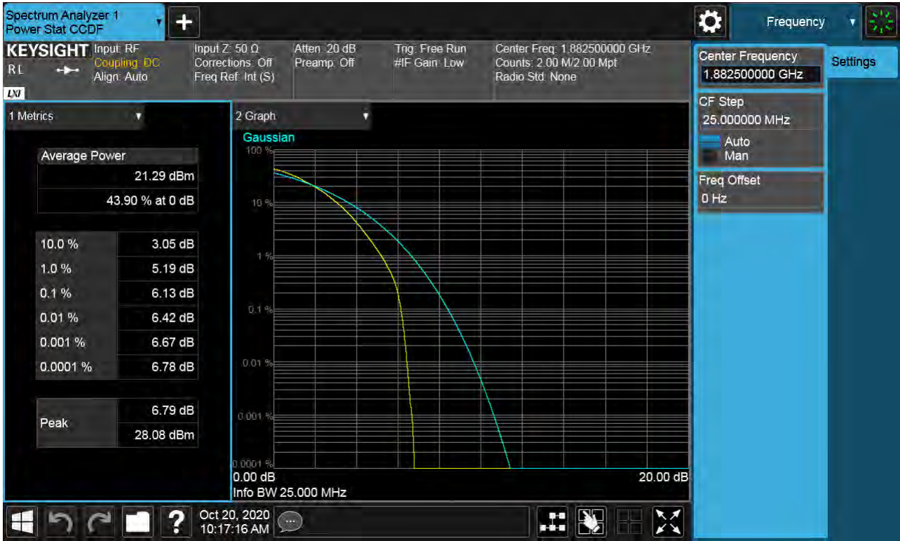
Sub6 n25(2). PAR Plot (25M BW Ch.376500 64QAM )
