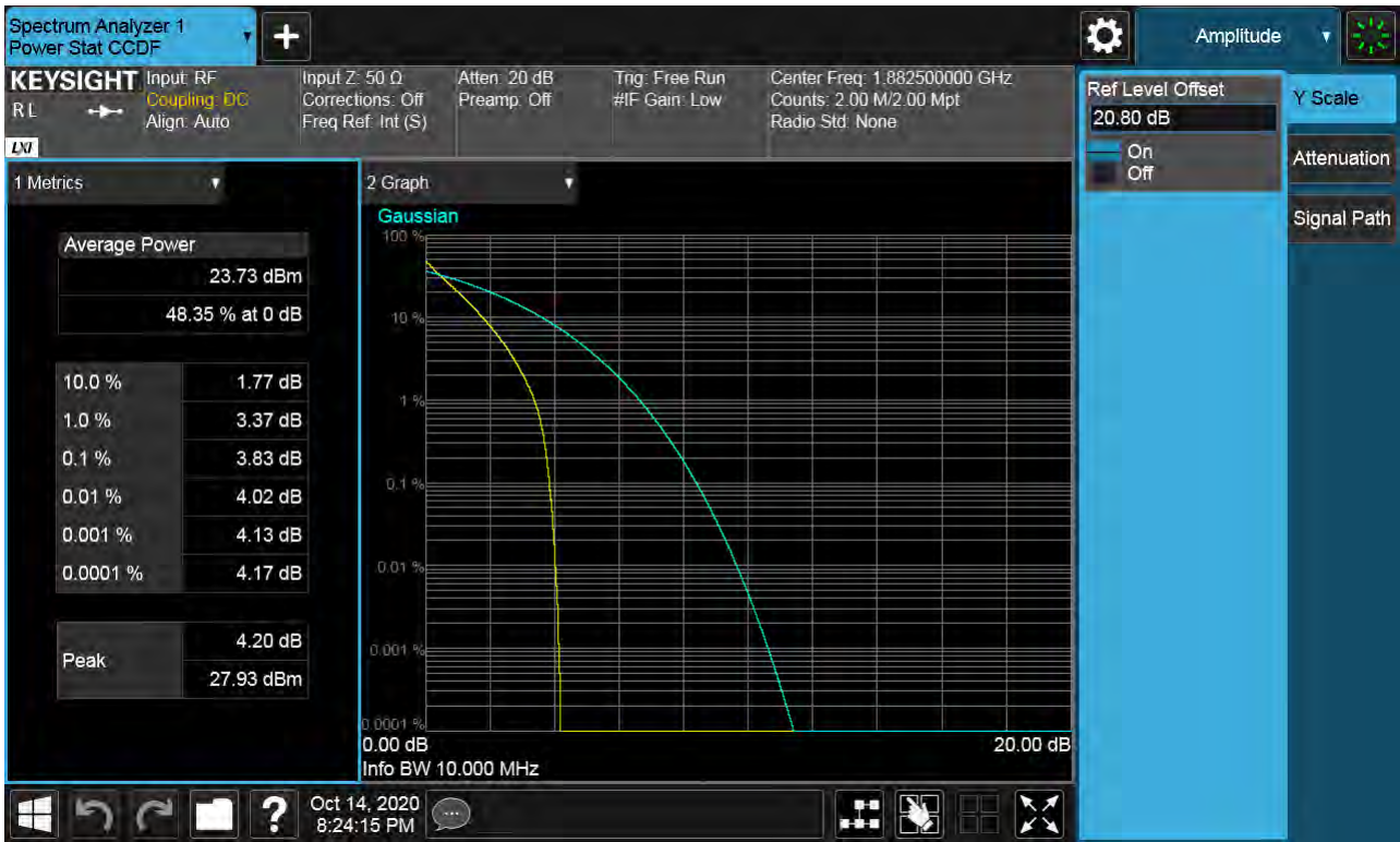
Sub6 n25(2). PAR Plot (10M BW Ch.376500 BPSK RB 50_0)
