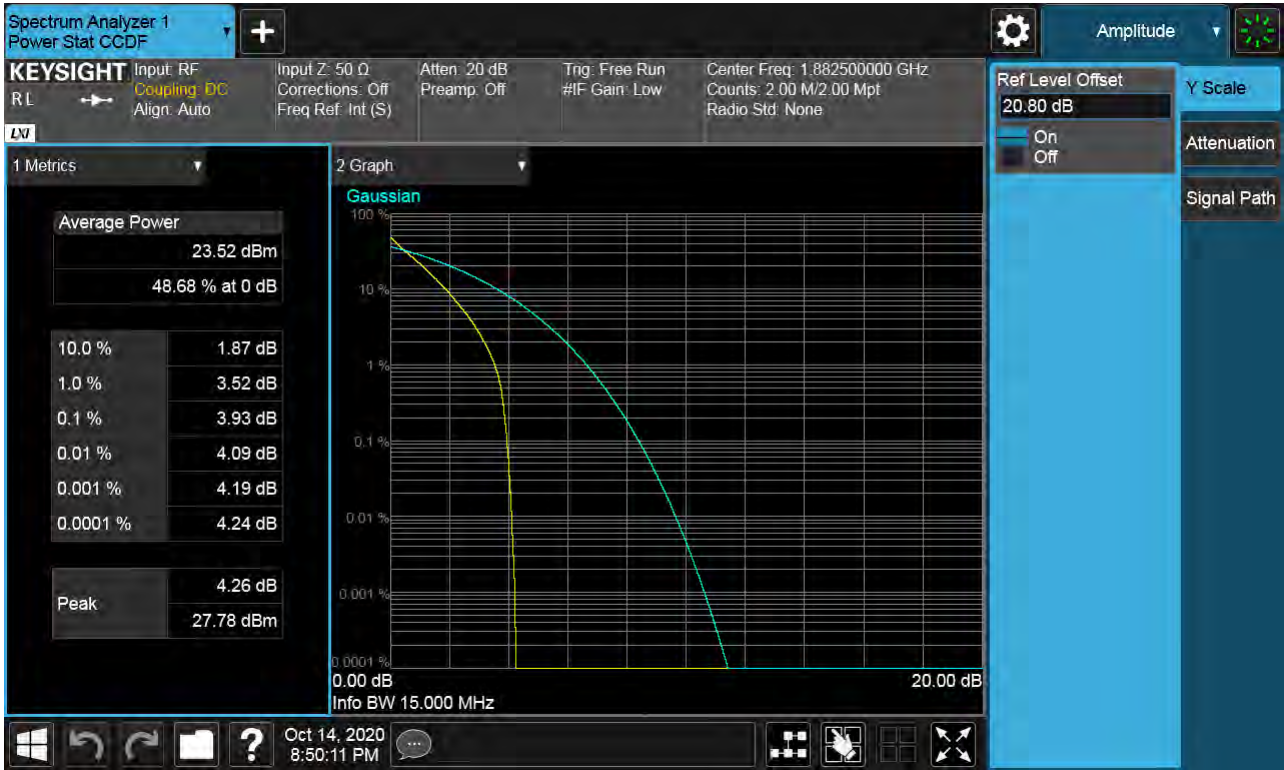
Sub6 n25(2). PAR Plot (15M BW Ch.376500 BPSK RB 75_0)
