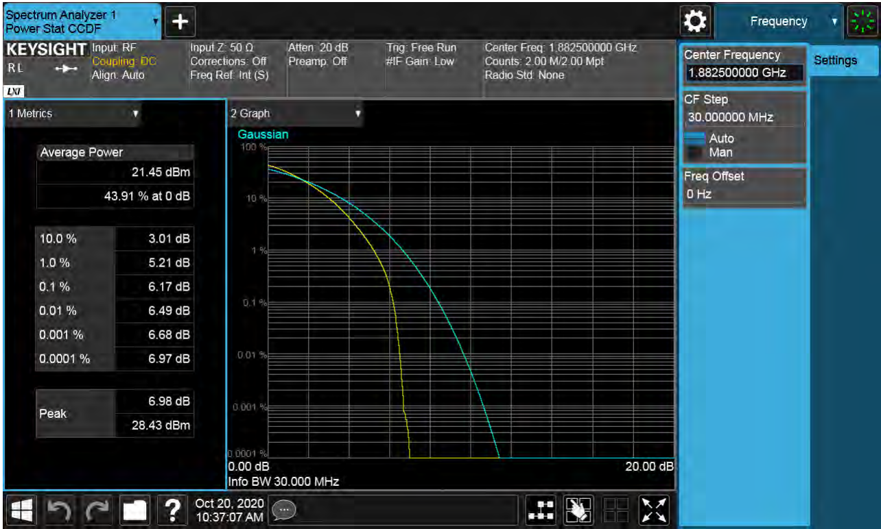
Sub6 n25(2). PAR Plot (30M BW Ch.376500 64QAM )
