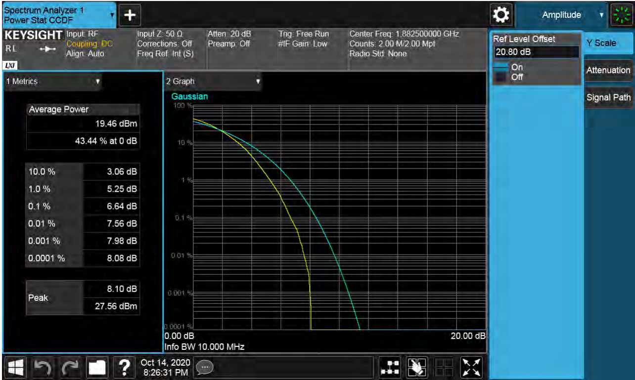
Sub6 n25(2). PAR Plot (10M BW Ch.376500 256QAM RB 50_0)
