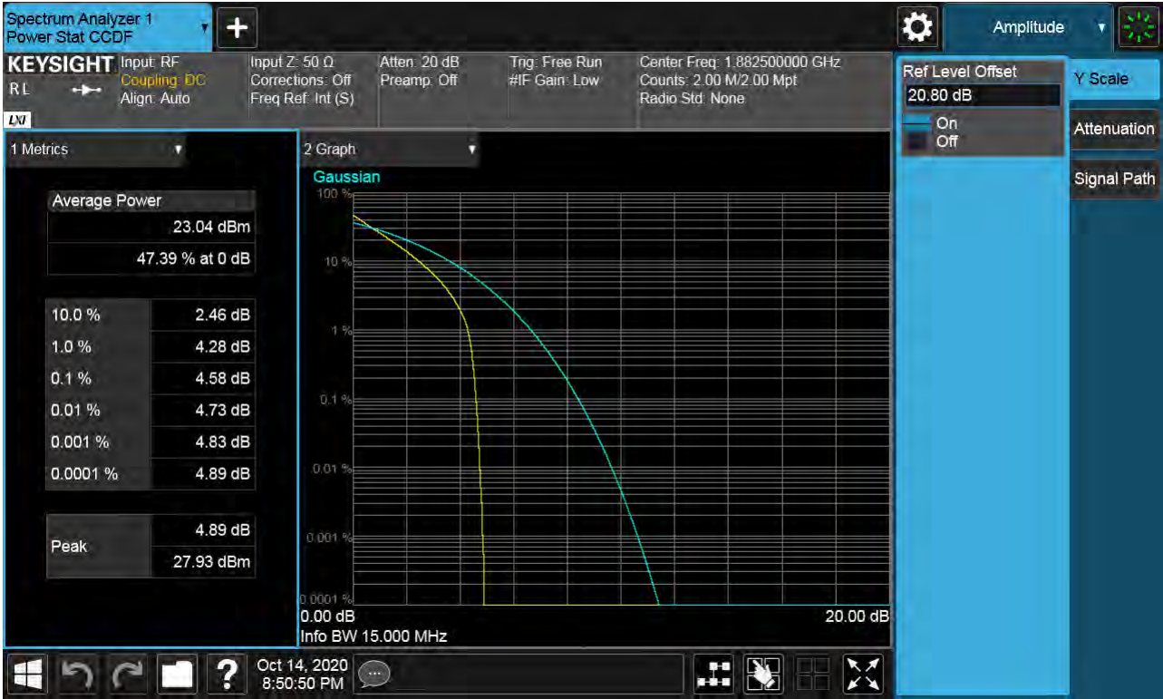
Sub6 n25(2). PAR Plot (15M BW Ch.376500 QPSK RB 75_0)
