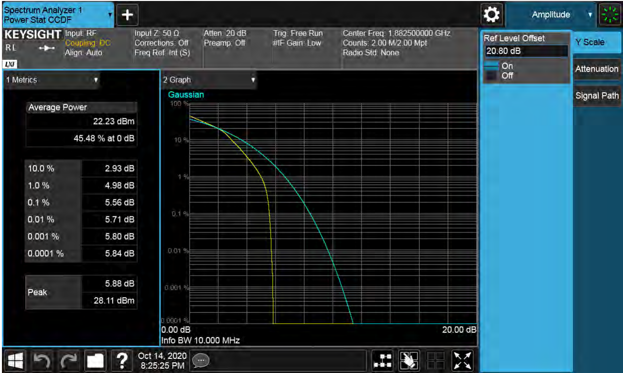
Sub6 n25(2). PAR Plot (10M BW Ch.376500 16QAM RB 50_0)
