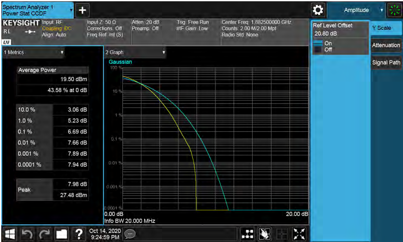
Sub6 n25(2). PAR Plot (20M BW Ch.376500 256QAM RB 100_0)
