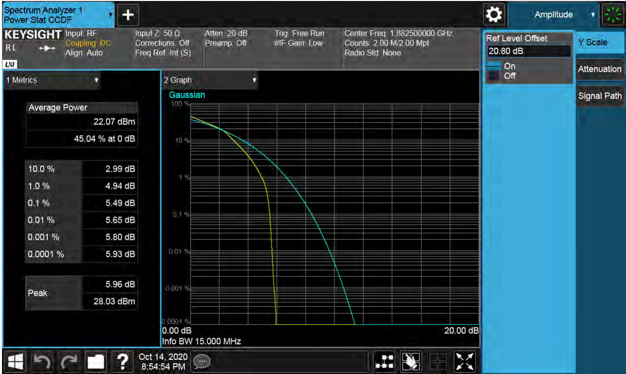
Sub6 n25(2). PAR Plot (15M BW Ch.376500 16QAM RB 75_0)
