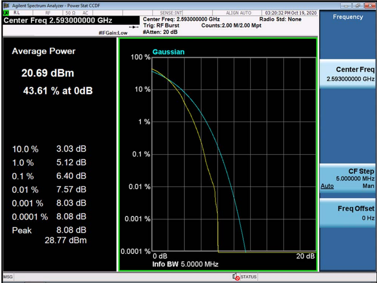
PAR Plot (5M BW_Ch.40620_64QAM_RB25_0) (POWER CLASS 3)
