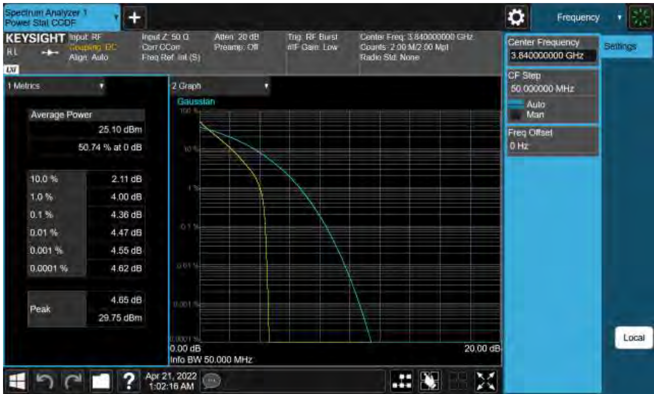
Sub6 n77. PAR Plot (50 M BW_Ch.656000_ BPSK)
