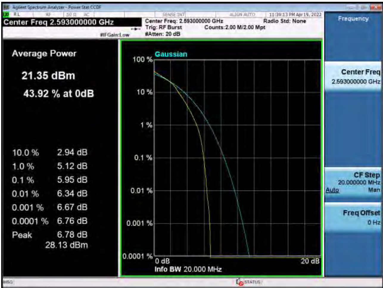
PAR Plot (20M BW_Ch.40620_16QAM_RB100_0) (POWER CLASS 3)
