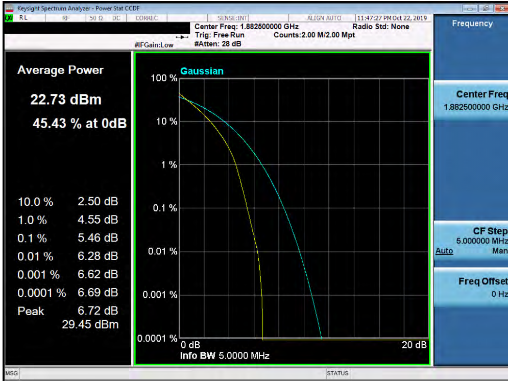
Plot 7-414. PAR Plot (Band 25/2 - 5.0MHz QPSK - Full RB Configuration)
