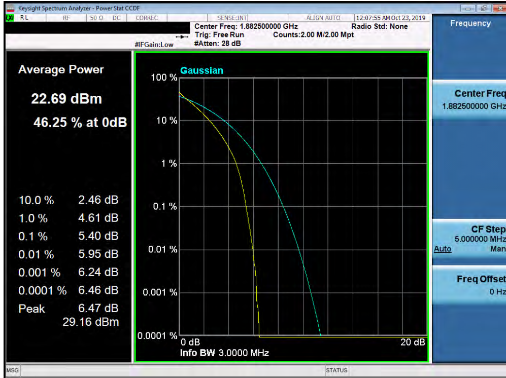
Plot 7-410. PAR Plot (Band 25/2 - 3.0MHz QPSK - Full RB Configuration)
