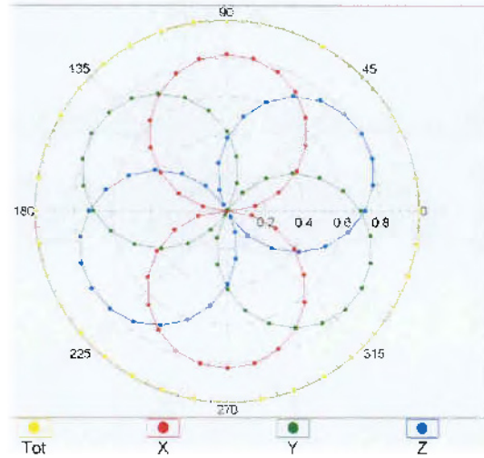
f=1800 MHz,R22
