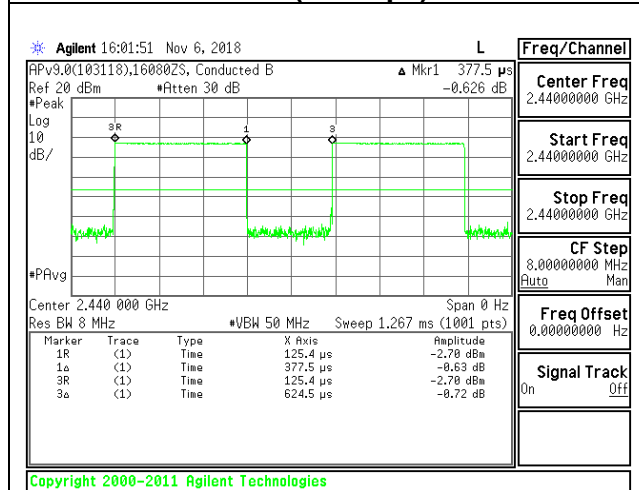
BLE (1Mbps)
