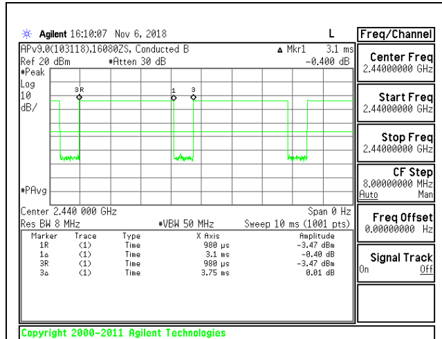
BLE (125kbps)
