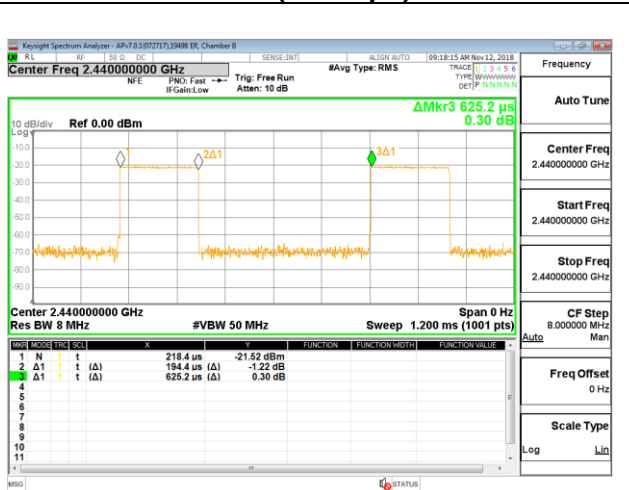
BLE (2Mbps)
