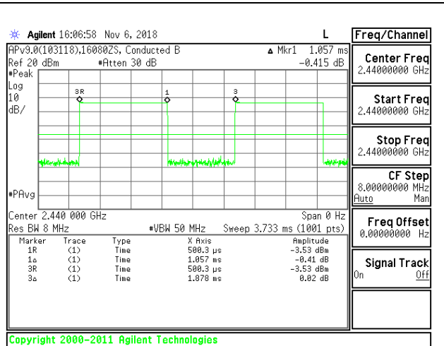
BLE (500kbps)
