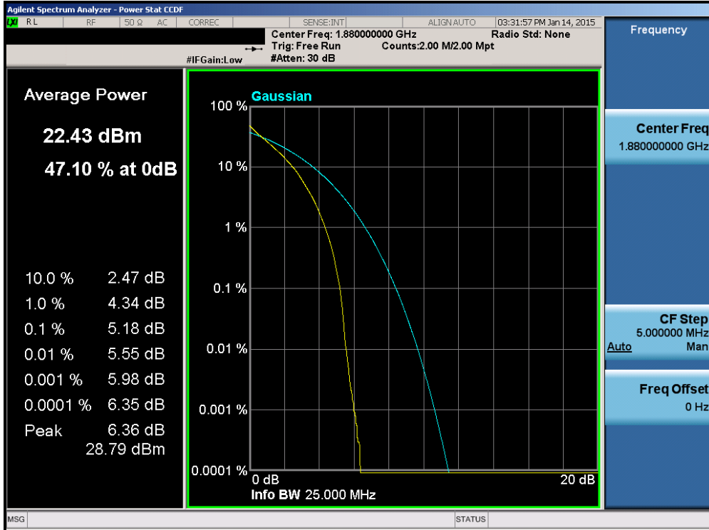
Plot 6-99. PAR Plot (Band 2 – 15.0MHz QPSK – RB Size 75)
