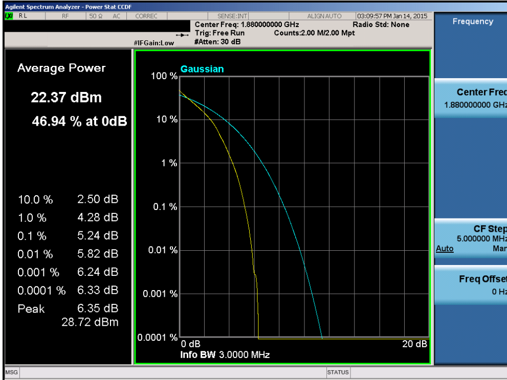
Plot 6-93. PAR Plot (Band 2 – 3.0MHz QPSK – RB Size 15)
