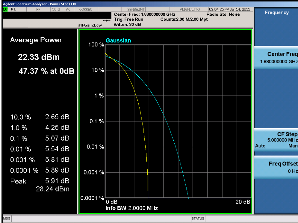
Plot 6-91. PAR Plot (Band 2 – 1.4MHz QPSK – RB Size 6)
