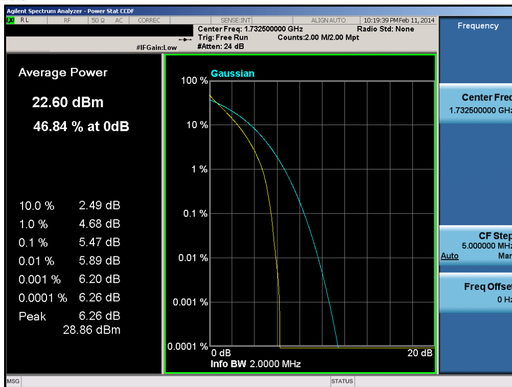
Plot 6-121. PAR Plot (Band 4 – 1.4MHz QPSK – RB Size 6)
