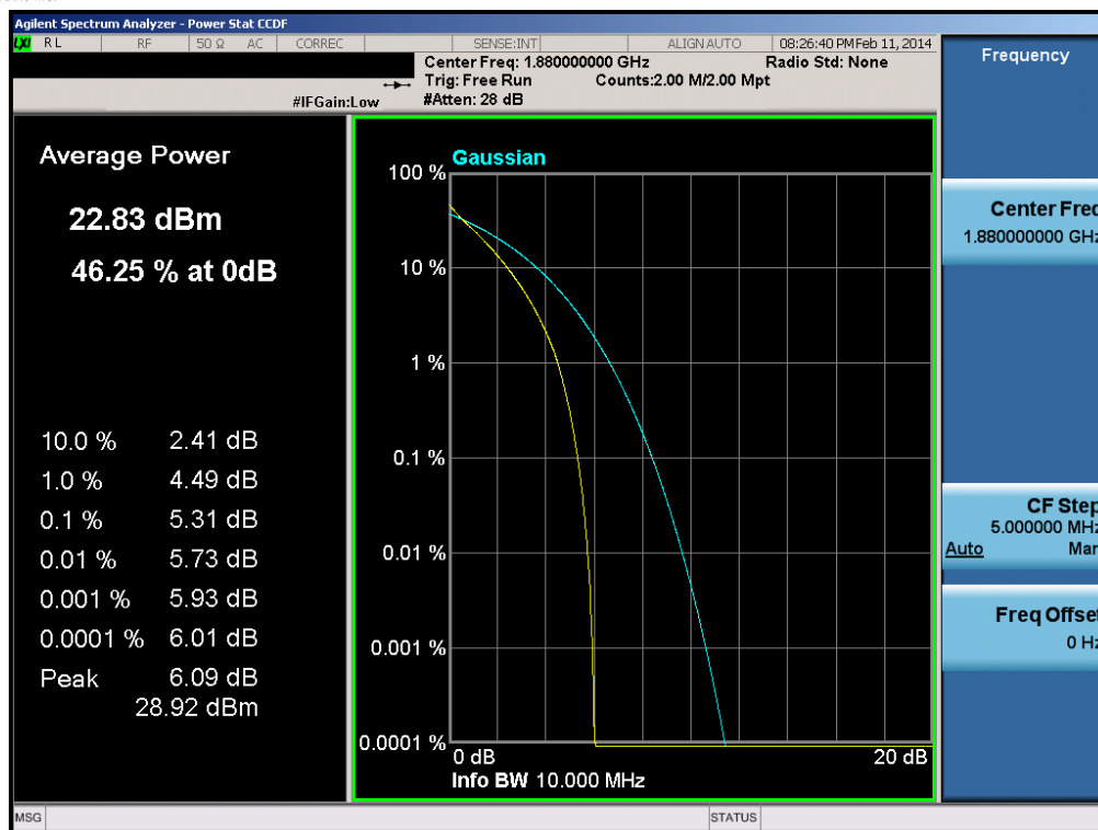
Plot 6-139. PAR Plot (Band 2 – 10.0MHz QPSK – RB Size 50)
