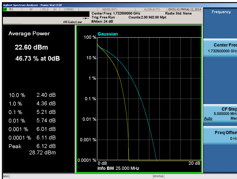
Plot 6-131. PAR Plot (Band 4 – 20.0MHz QPSK – RB Size 100)
