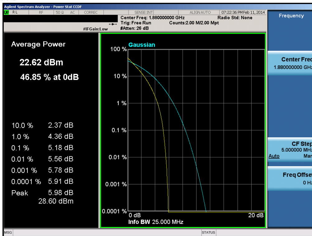
Plot 6-143. PAR Plot (Band 2 – 20.0MHz QPSK – RB Size 100)
