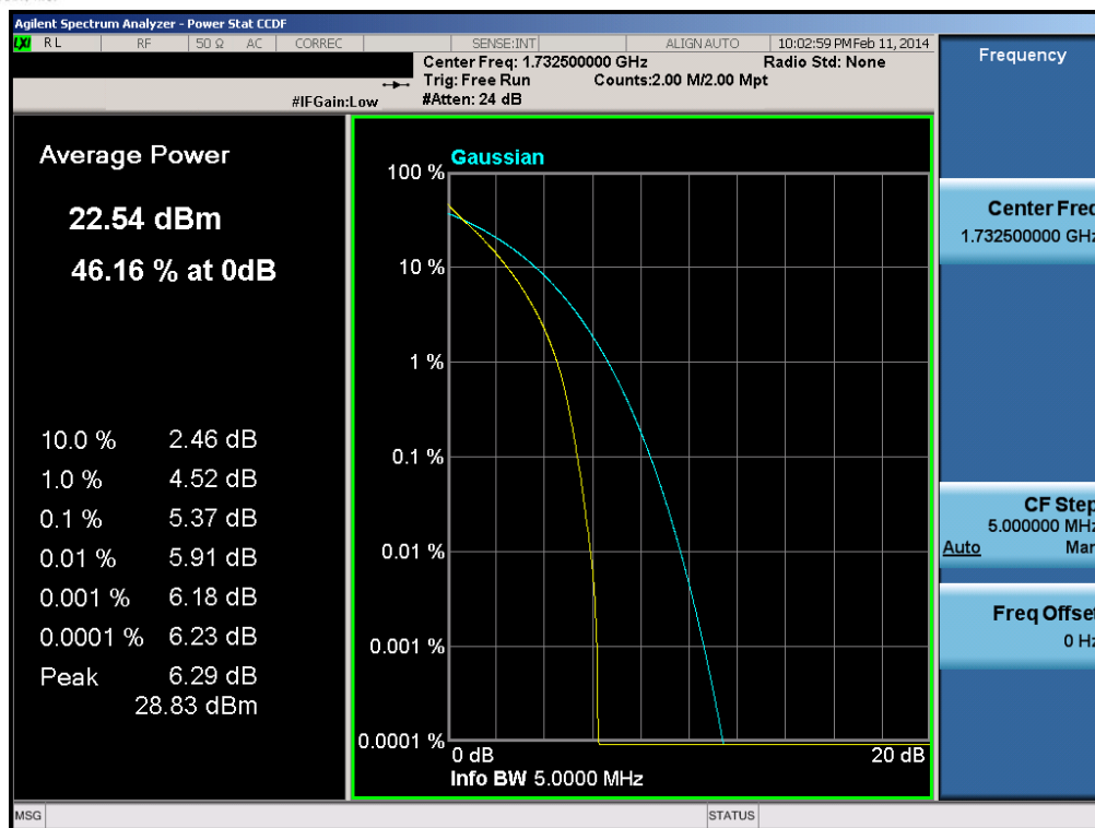
Plot 6-125. PAR Plot (Band 4 – 5.0MHz QPSK – RB Size 25)
