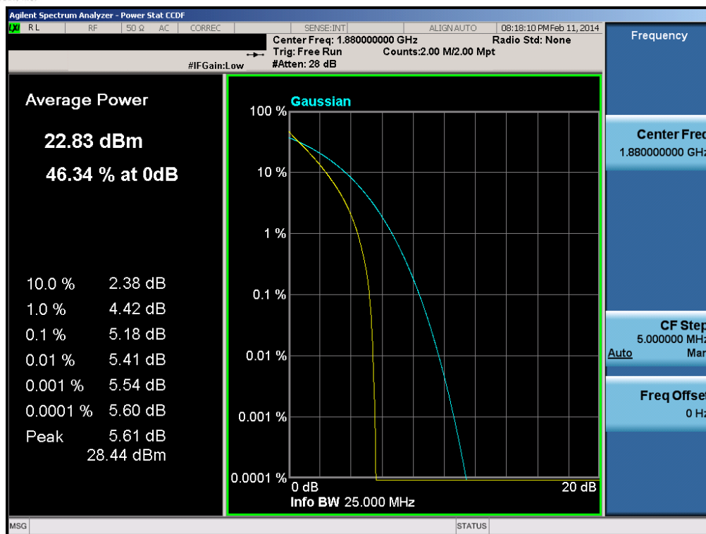
Plot 6-141. PAR Plot (Band 2 – 15.0MHz QPSK – RB Size 75)
