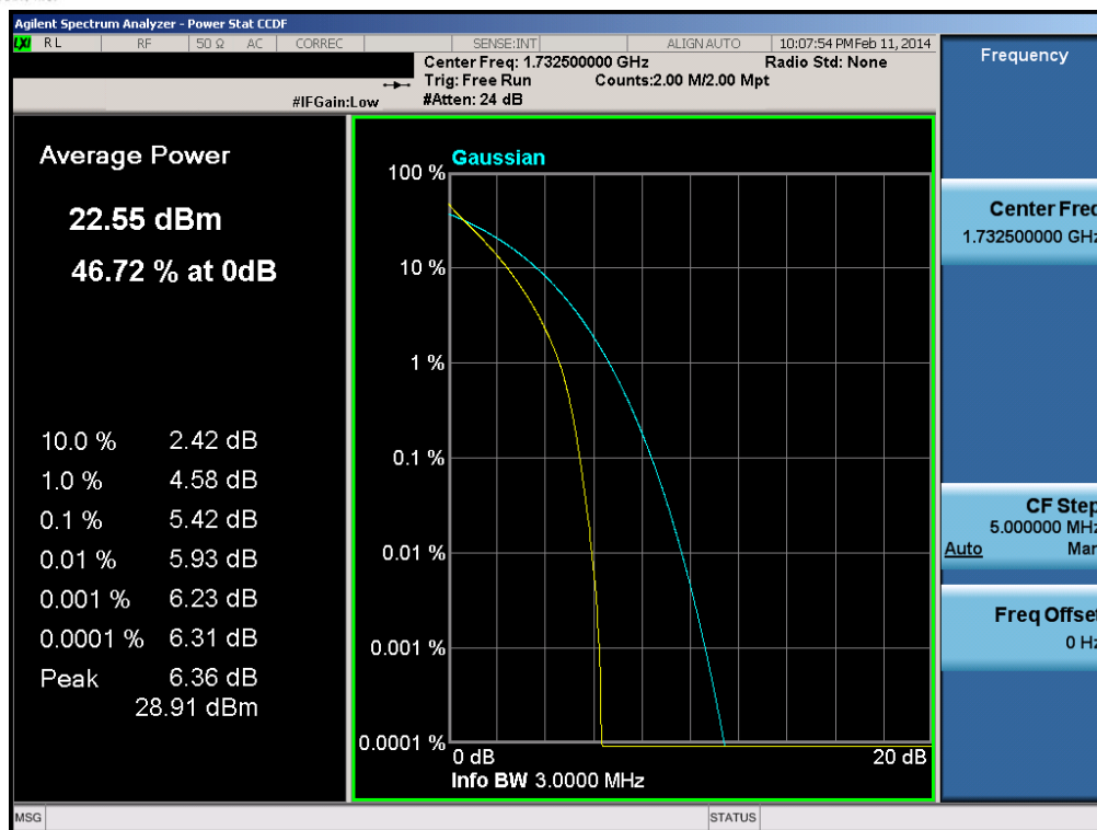
Plot 6-123. PAR Plot (Band 4 – 3.0MHz QPSK – RB Size 15)
