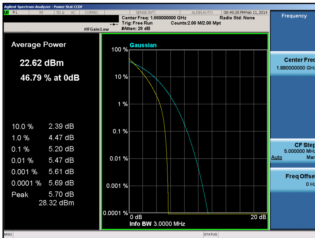
Plot 6-135. PAR Plot (Band 2 – 3.0MHz QPSK – RB Size 15)
