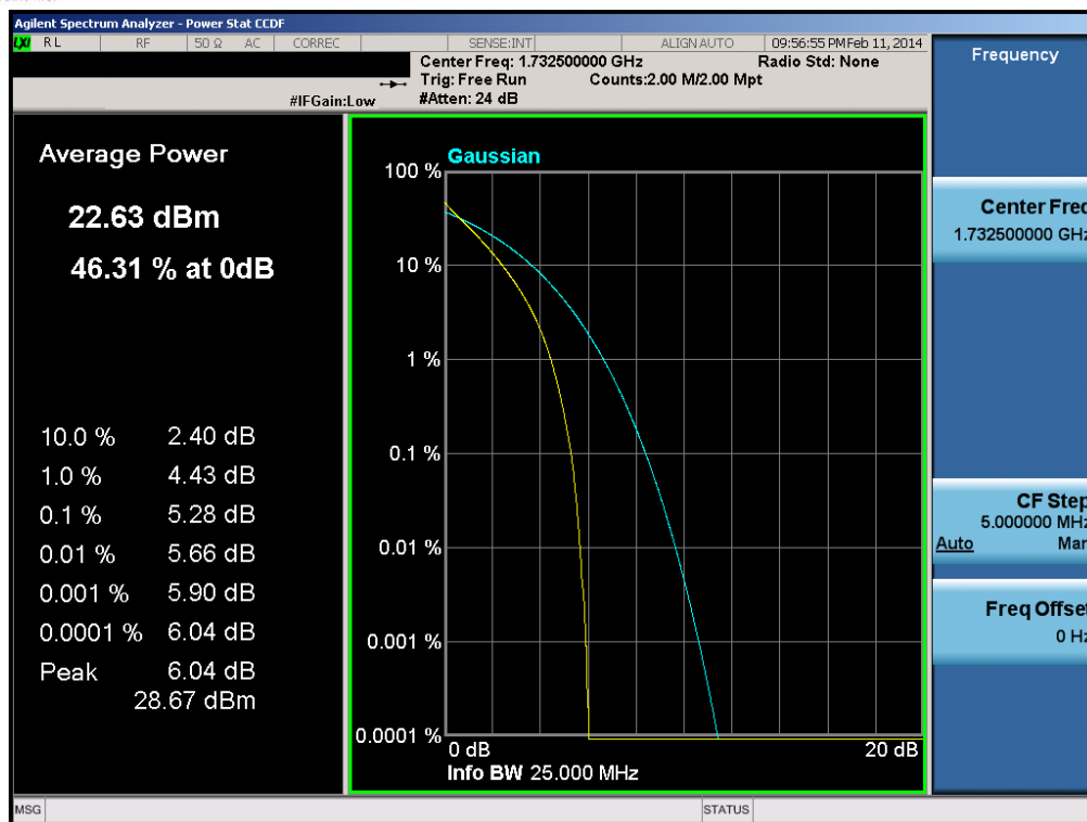
Plot 6-129. PAR Plot (Band 4 – 15.0MHz QPSK – RB Size 75)
