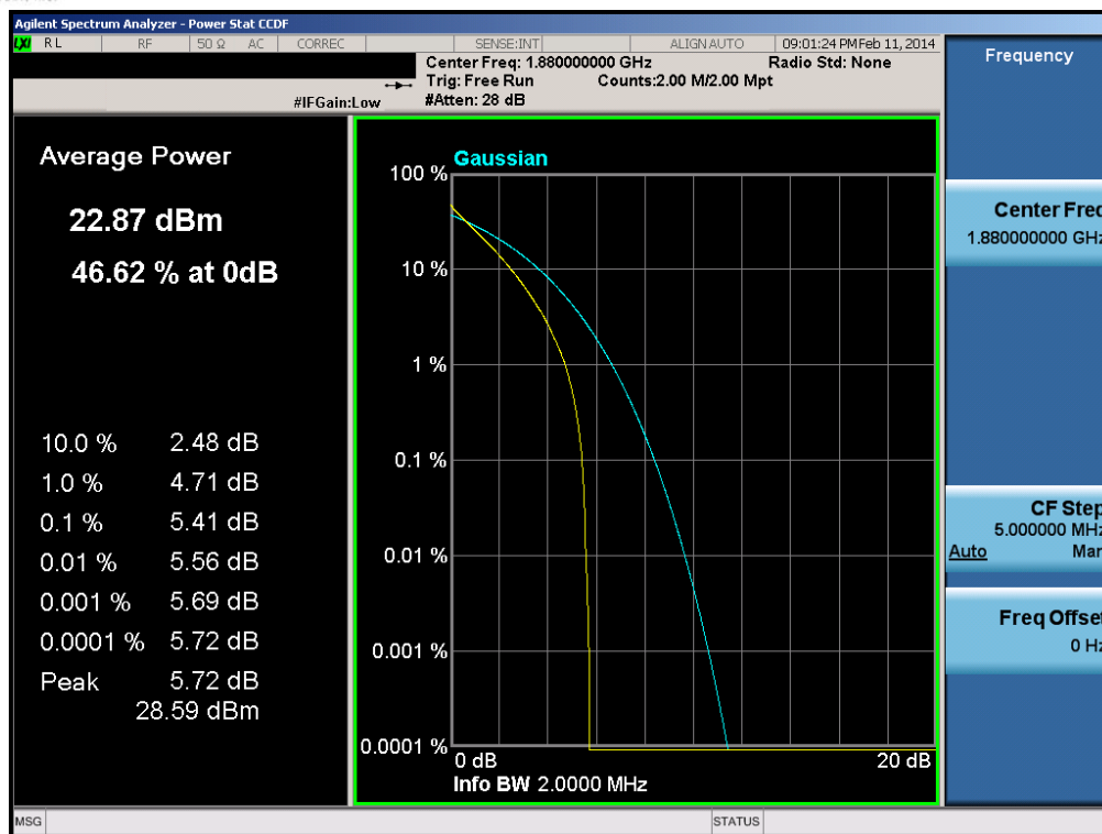
Plot 6-133. PAR Plot (Band 2 – 1.4MHz QPSK – RB Size 6)
