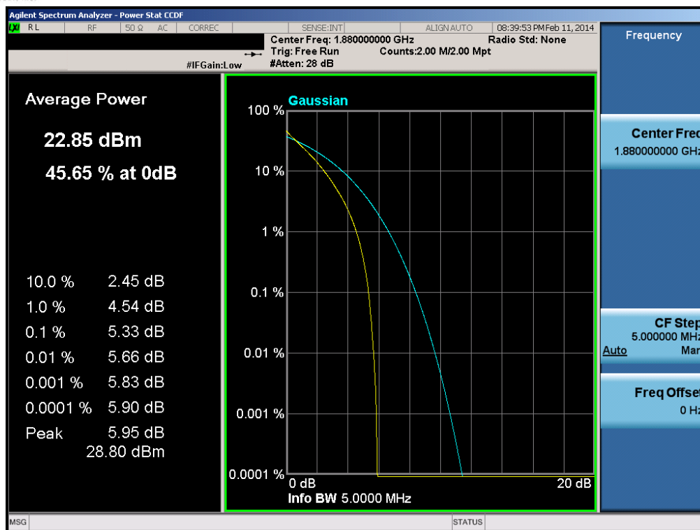
Plot 6-137. PAR Plot (Band 2 – 5.0MHz QPSK – RB Size 25)
