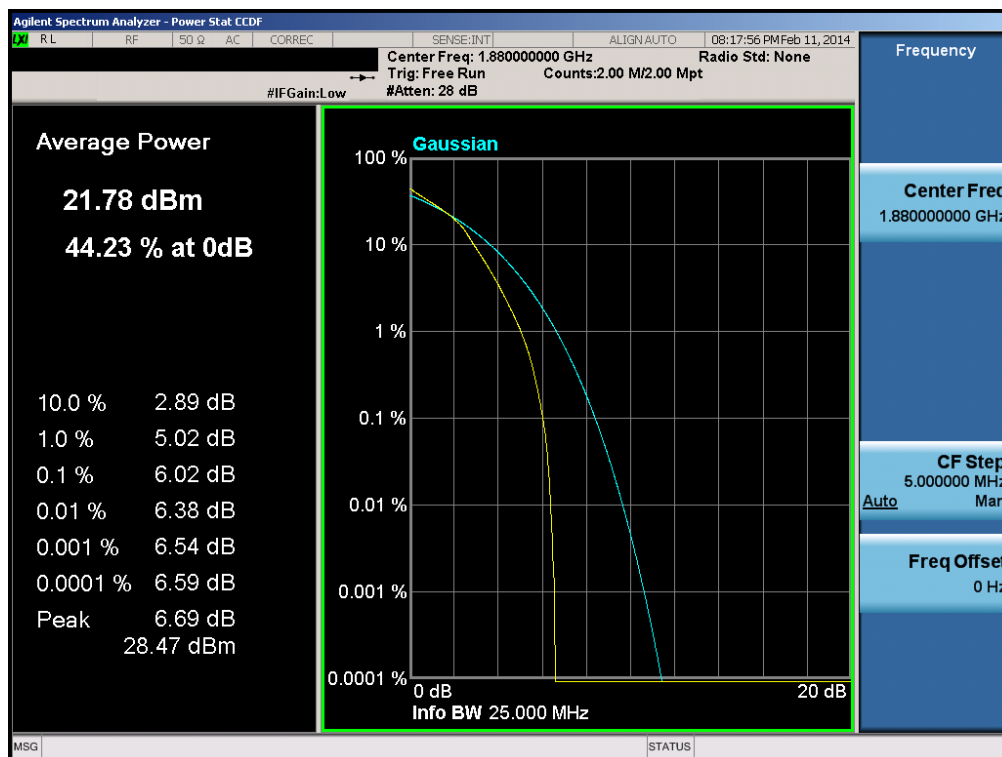
Plot 6-142. PAR Plot (Band 2 – 15.0MHz 16-QAM – RB Size 75)
