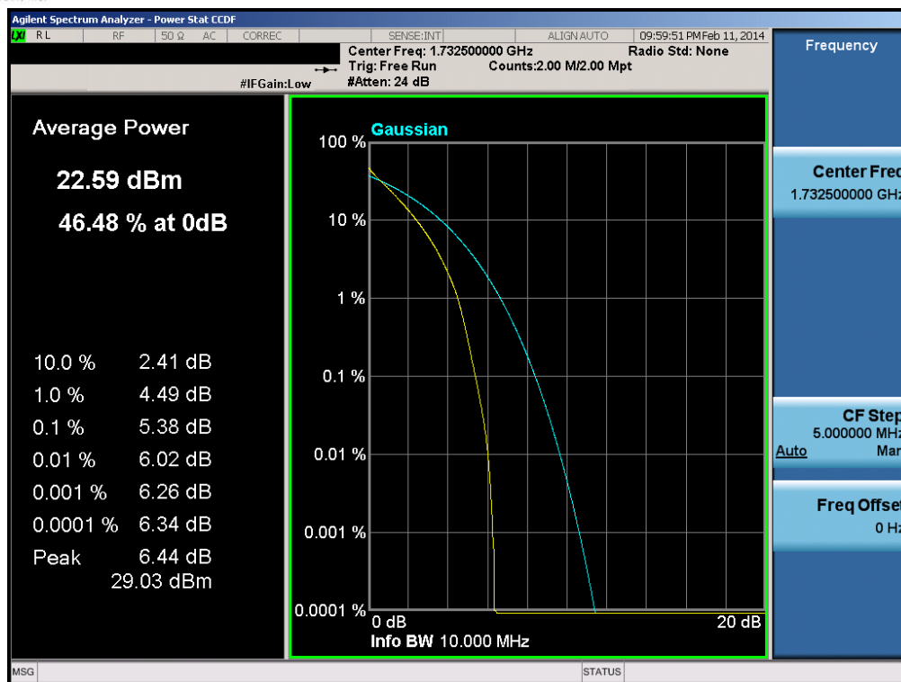
Plot 6-127. PAR Plot (Band 4 – 10.0MHz QPSK – RB Size 50)
