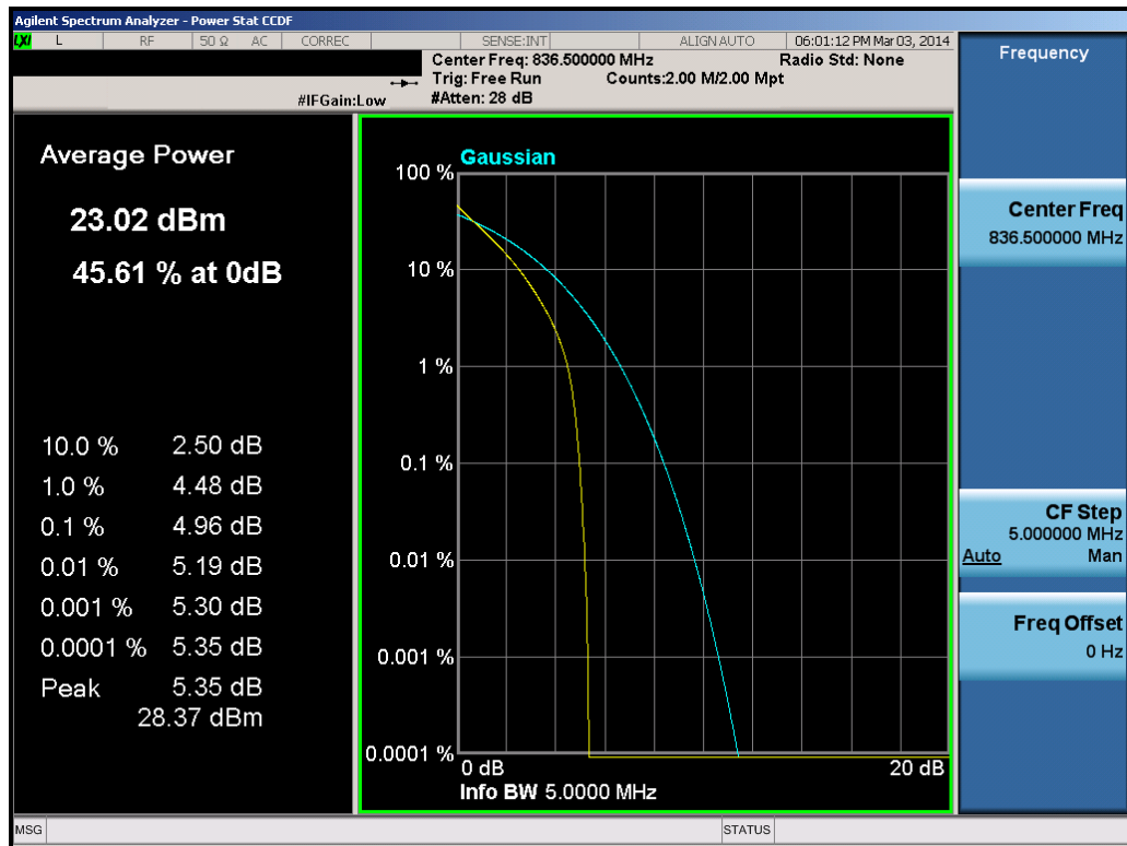
Plot 8-11. PAR Plot (5.0MHz QPSK – RB Size 25)
