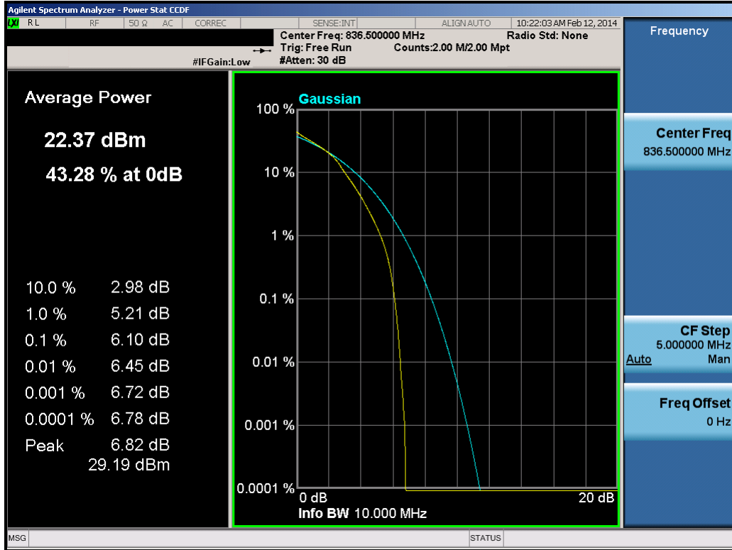
Plot 8-24. PAR Plot (10.0MHz 16-QAM – RB Size 50)
