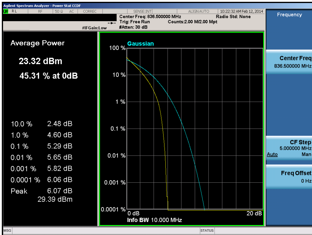
Plot 8-23. PAR Plot (10.0MHz QPSK – RB Size 50)
