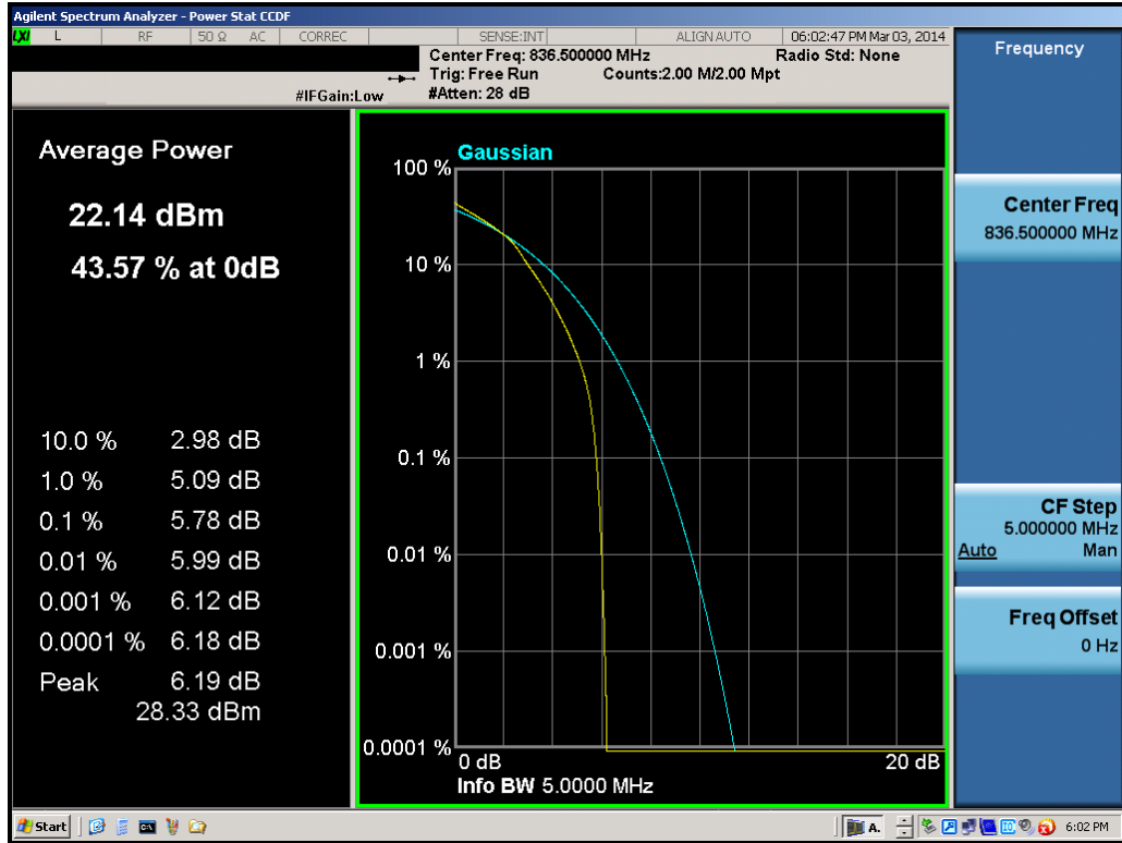
Plot 8-12. PAR Plot (5.0MHz 16-QAM – RB Size 25)
