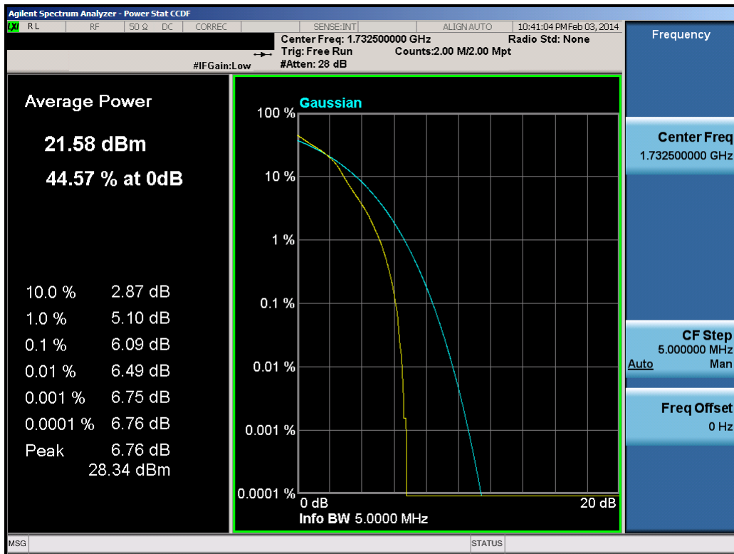
Plot 8-7. PAR Plot (5.0MHz QPSK – RB Size 25)
