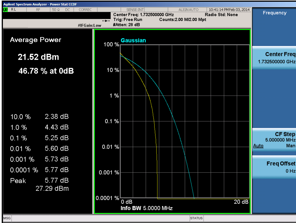
Plot 8-8. PAR Plot (5.0MHz 16-QAM – RB Size 25)
