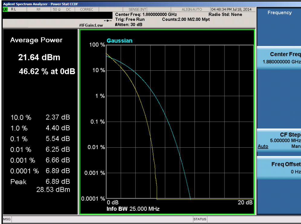
Plot 6-83. PAR Plot (Band 2 – 20.0MHz QPSK – RB Size 100)
