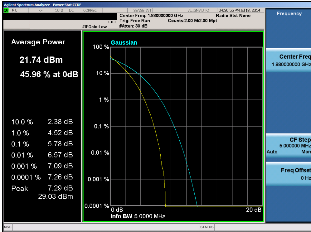
Plot 6-77. PAR Plot (Band 2 – 5.0MHz QPSK – RB Size 25)
