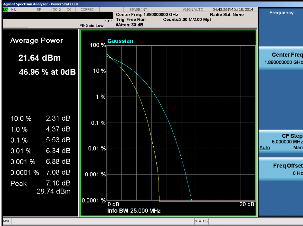
Plot 6-81. PAR Plot (Band 2 – 15.0MHz QPSK – RB Size 75)
