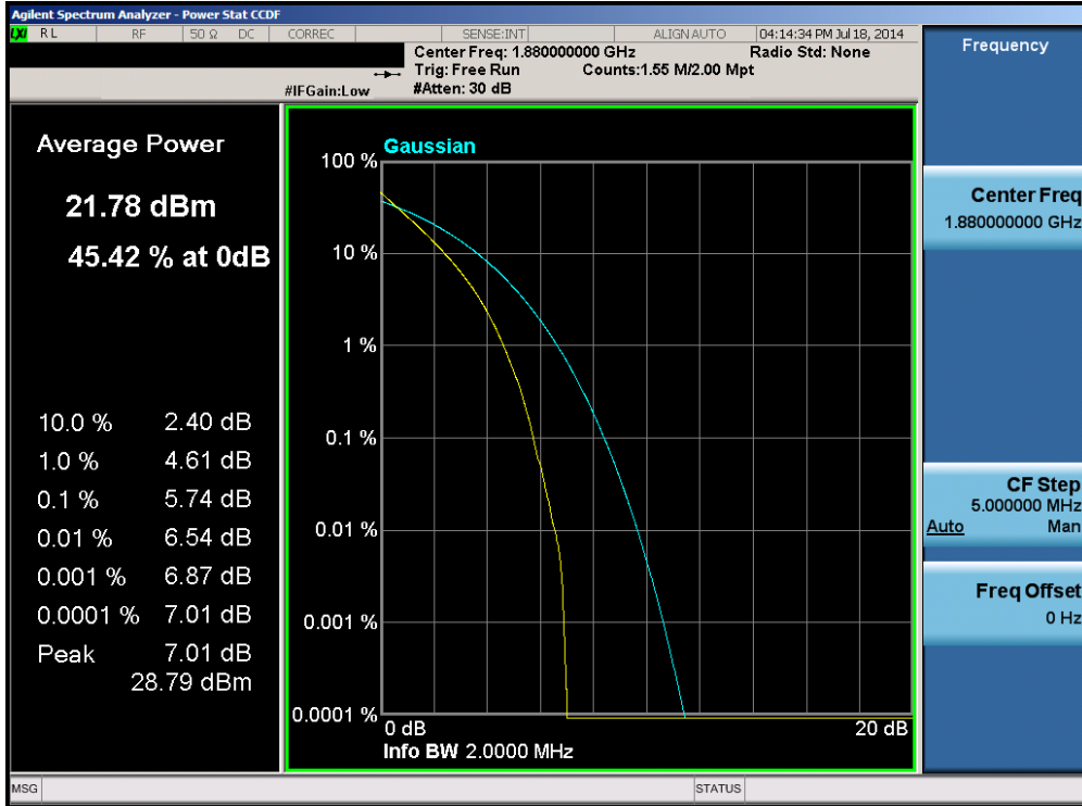
Plot 6-73. PAR Plot (Band 2 – 1.4MHz QPSK – RB Size 6)
