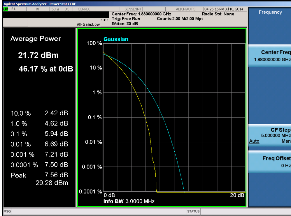
Plot 6-75. PAR Plot (Band 2 – 3.0MHz QPSK – RB Size 15)
