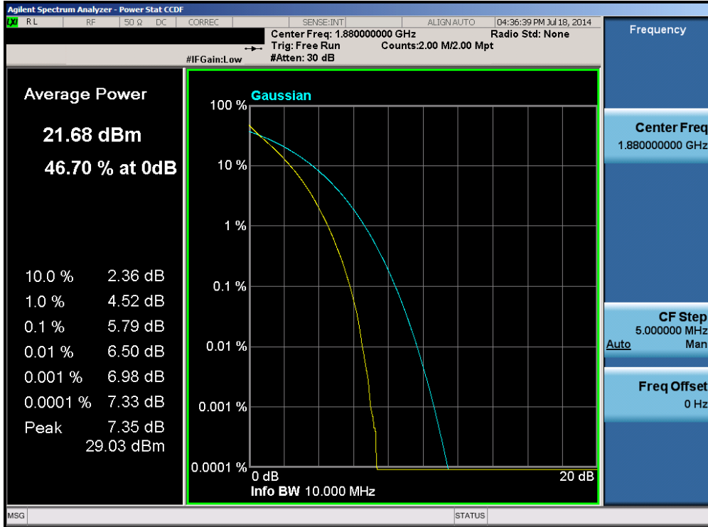
Plot 6-79. PAR Plot (Band 2 – 10.0MHz QPSK – RB Size 50)
