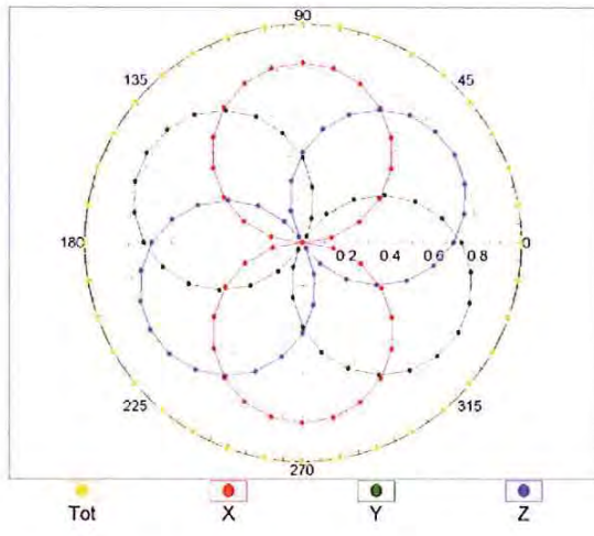
f=1800 MHz,R22
