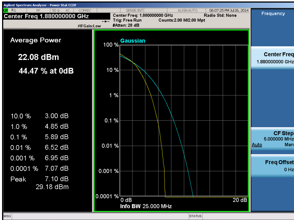
Plot 6-249. PAR Plot (Band 2 – 20.0MHz 16-QAM – RB Size 100)
