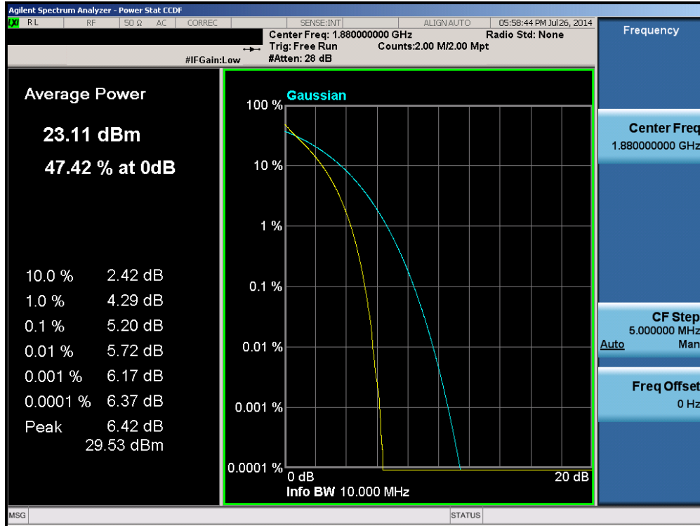
Plot 6-244. PAR Plot (Band 2 – 10.0MHz QPSK – RB Size 50)
