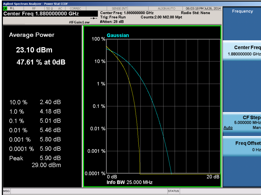
Plot 6-246. PAR Plot (Band 2 – 15.0MHz QPSK – RB Size 75)
