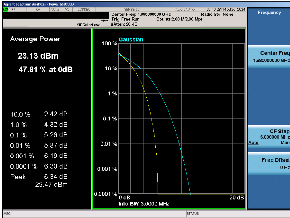
Plot 6-240. PAR Plot (Band 2 – 3.0MHz QPSK – RB Size 15)
