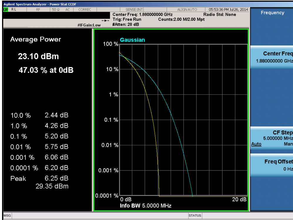
Plot 6-242. PAR Plot (Band 2 – 5.0MHz QPSK – RB Size 25)
