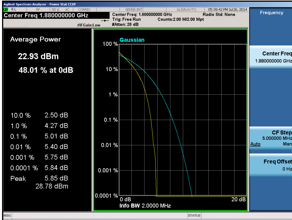
Plot 6-238. PAR Plot (Band 2 – 1.4MHz QPSK – RB Size 6)
