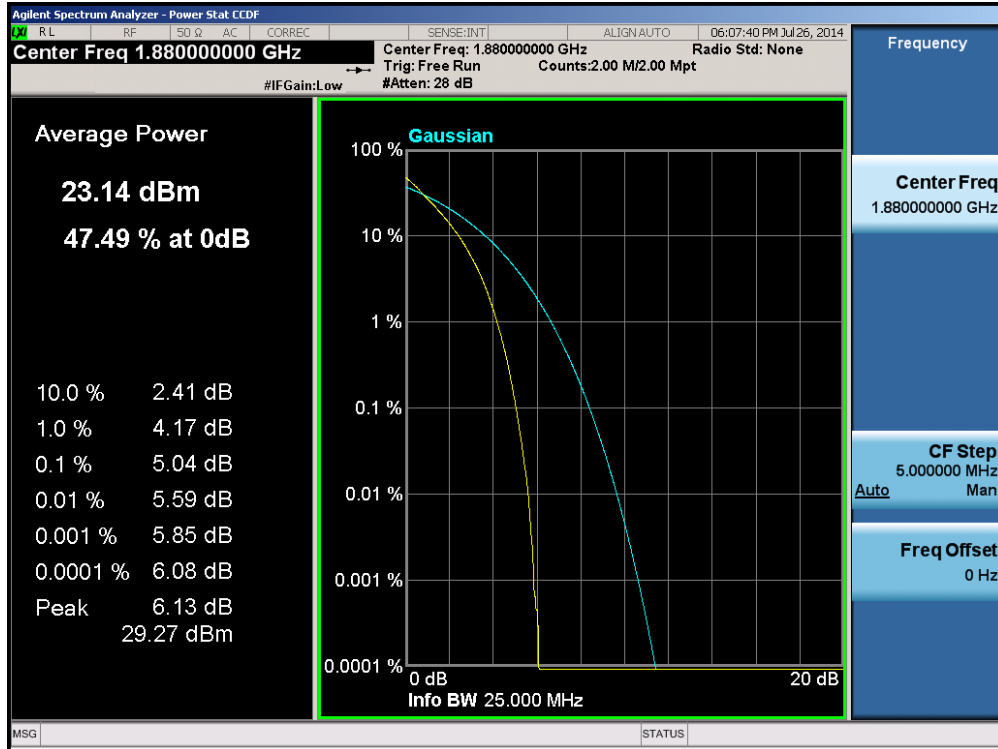
Plot 6-248. PAR Plot (Band 2 – 20.0MHz QPSK – RB Size 100)
