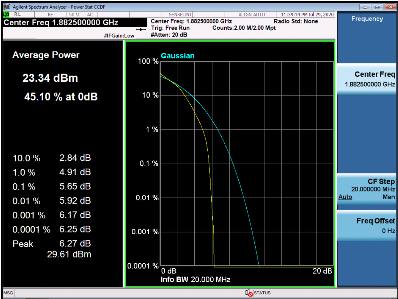
Sub6 n25(2). PAR Plot (20M BW Ch.376500 16QAM RB 100_0)
