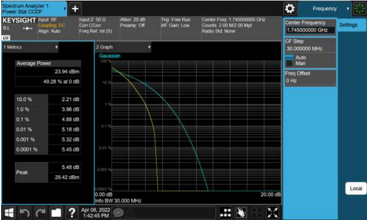
Sub6 n66. PAR Plot (30 M BW_Ch.349000_QPSK_Full RB)
