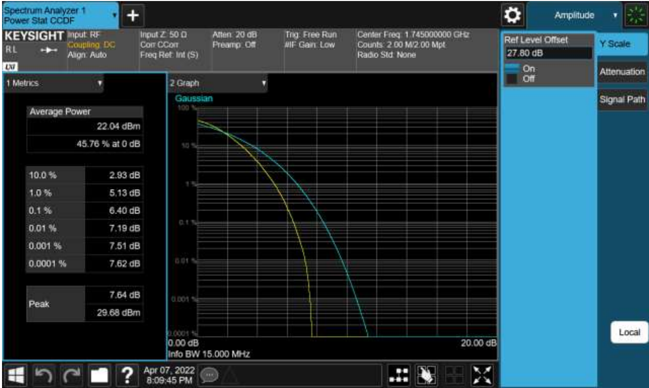
Sub6 n66. PAR Plot (15 M BW_Ch.349000_64QAM_Full RB)
