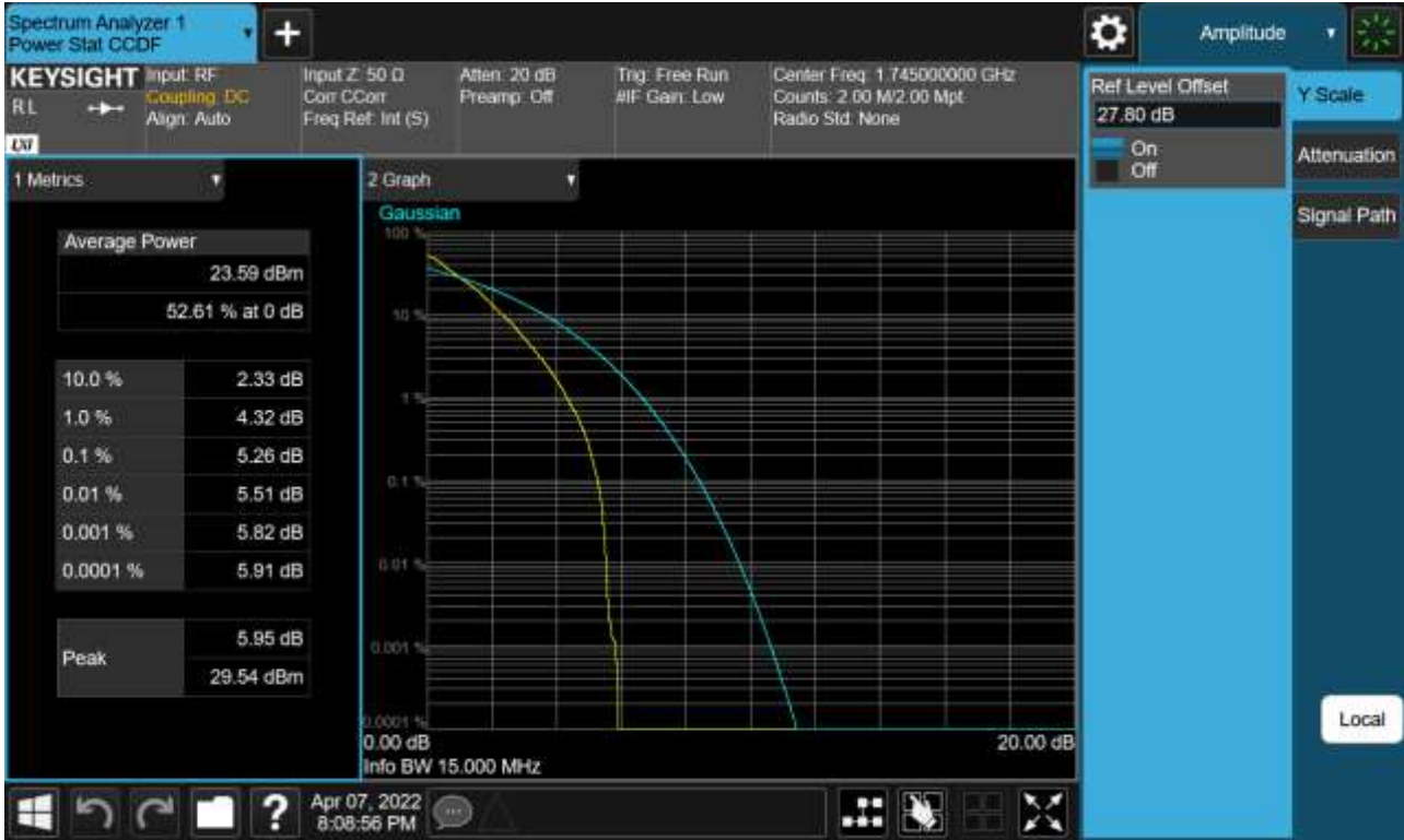
Sub6 n66. PAR Plot (15 M BW_Ch.349000_QPSK_Full RB)
