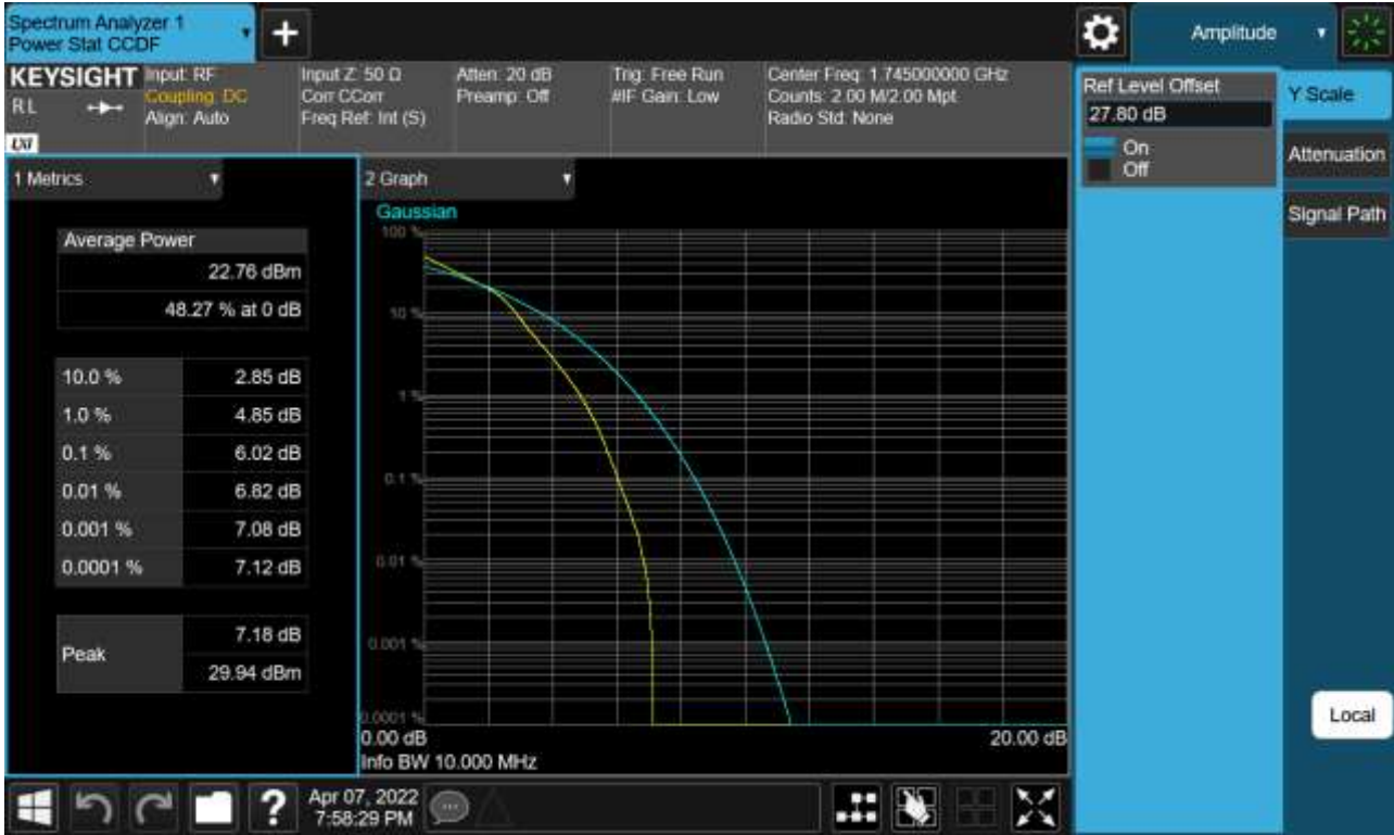
Sub6 n66. PAR Plot (10 M BW_Ch.349000_16QAM_Full RB)
