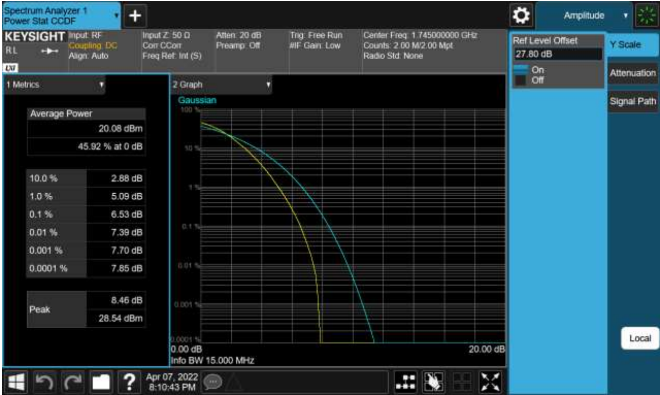
Sub6 n66. PAR Plot (15 M BW_Ch.349000_256QAM_Full RB)
