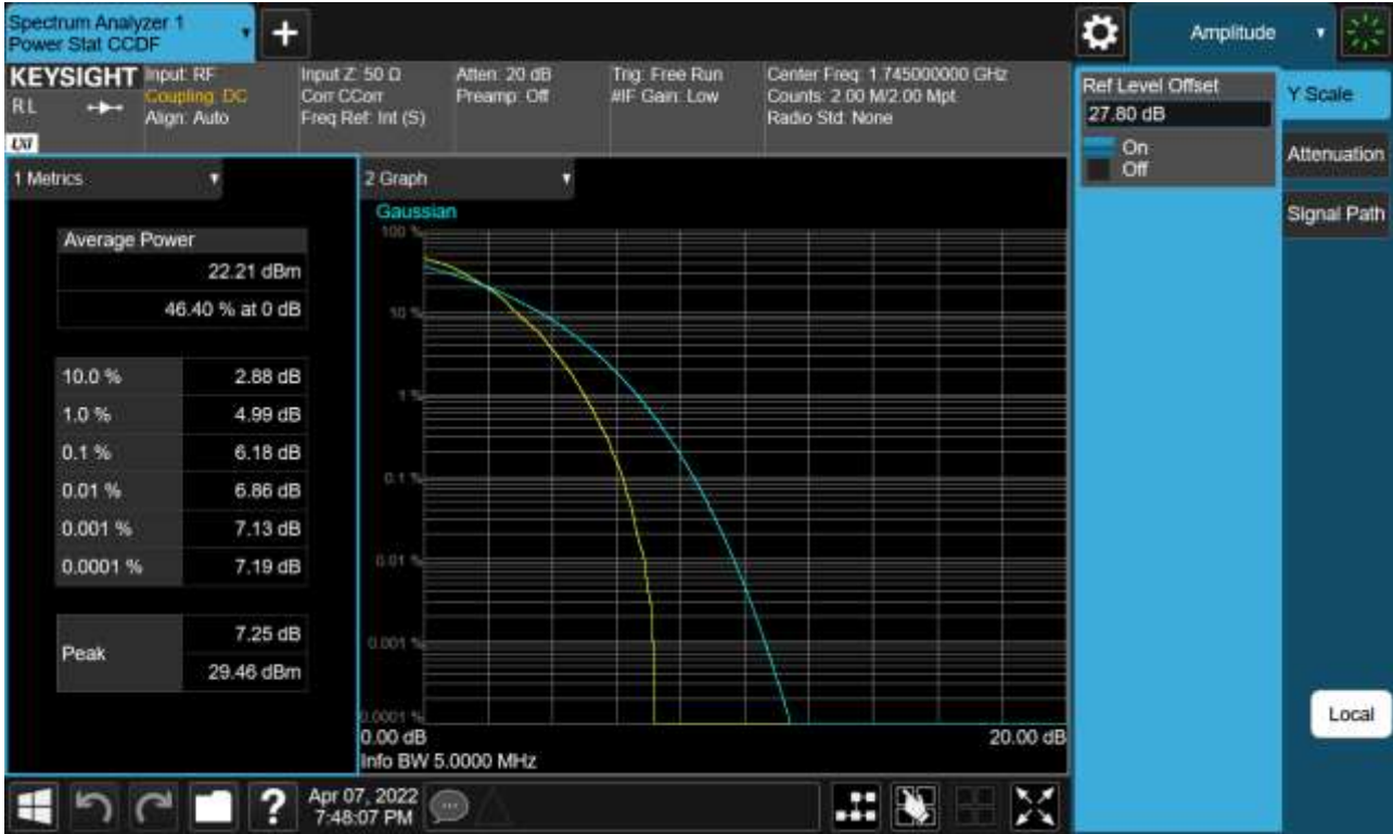
Sub6 n66. PAR Plot (5 M BW_Ch.349000_64QAM_Full RB)
