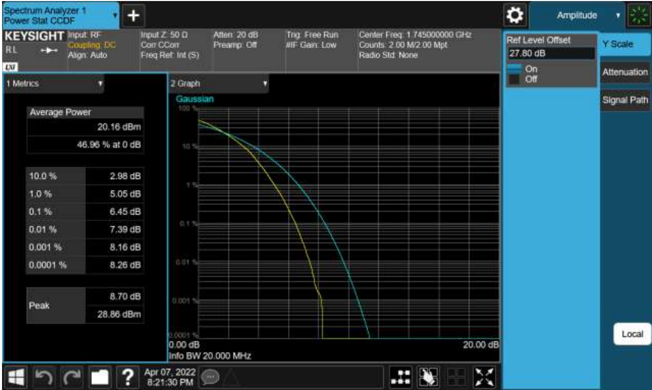
Sub6 n66. PAR Plot (20 M BW_Ch.349000_256QAM_Full RB)
