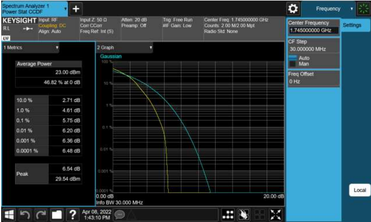
Sub6 n66. PAR Plot (30 M BW_Ch.349000_16QAM_Full RB)
