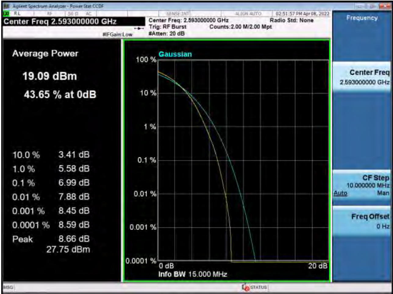
PAR Plot (15M BW_Ch.40620_256QAM_RB75_0) (POWER CLASS 3)
