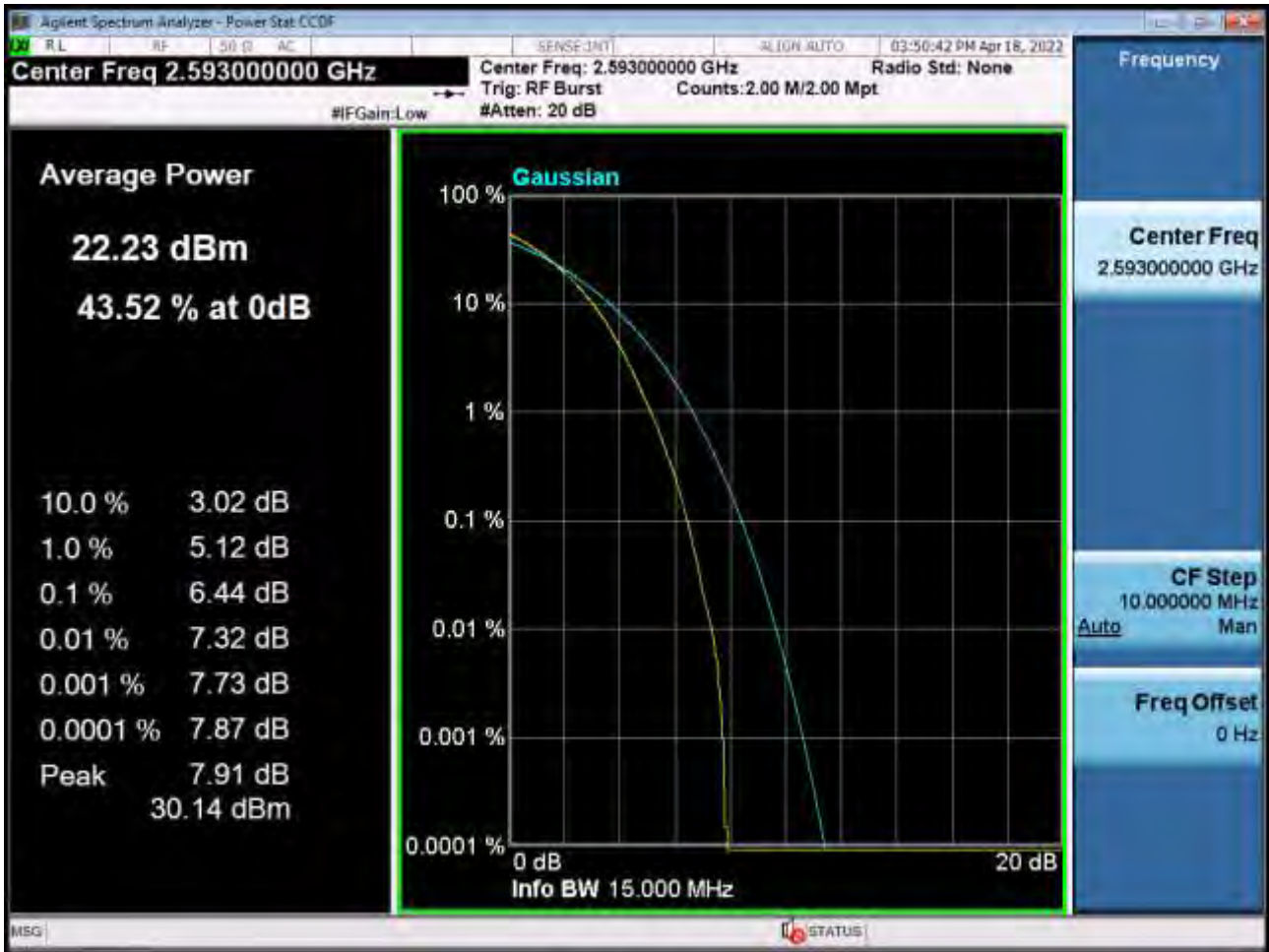
PAR Plot (15M BW_Ch.40620_256QAM_RB75_0) (POWER CLASS 2)
