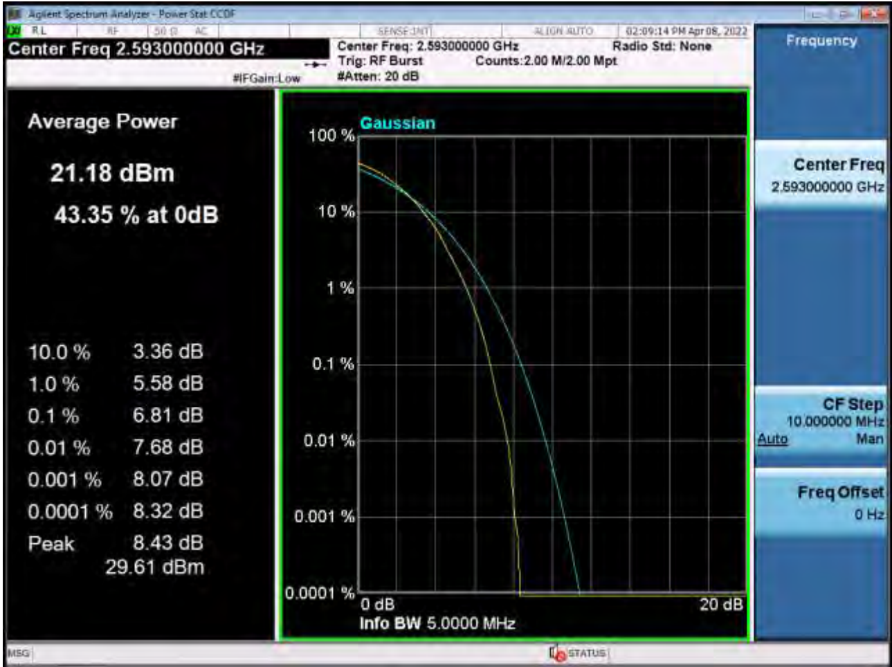
PAR Plot (5M BW_Ch.40620_64QAM_RB25_0) (POWER CLASS 3)
