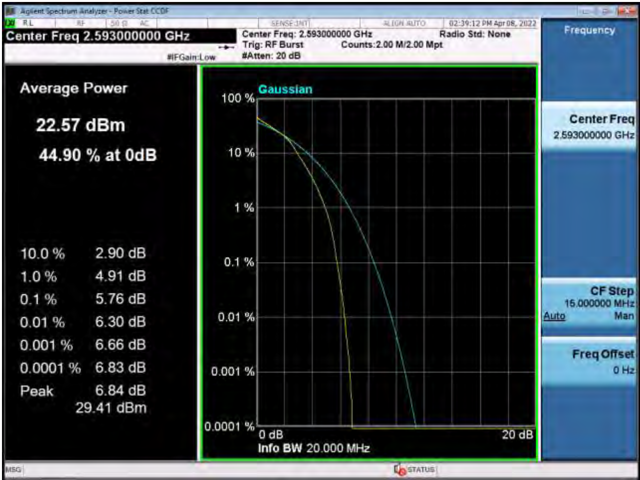
PAR Plot (20M BW_Ch.40620_16QAM_RB100_0) (POWER CLASS 3)
