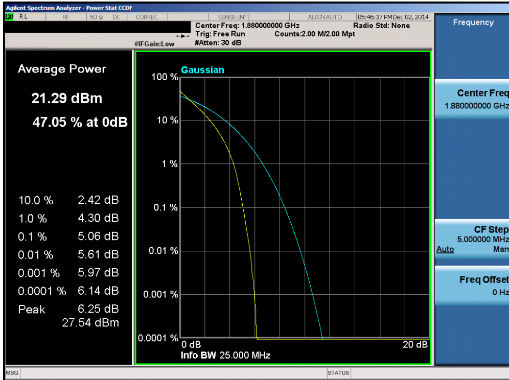
Plot 6-113. PAR Plot (Band 2 – 20.0MHz QPSK – RB Size 100)
