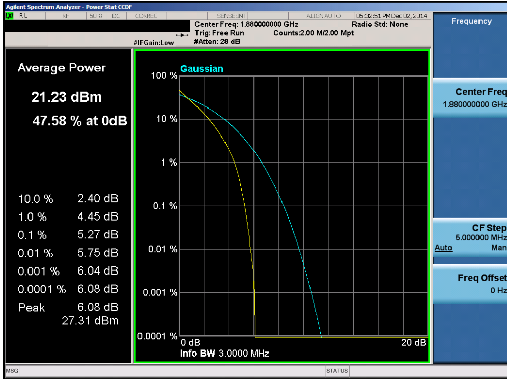
Plot 6-105. PAR Plot (Band 2 – 3.0MHz QPSK – RB Size 15)
