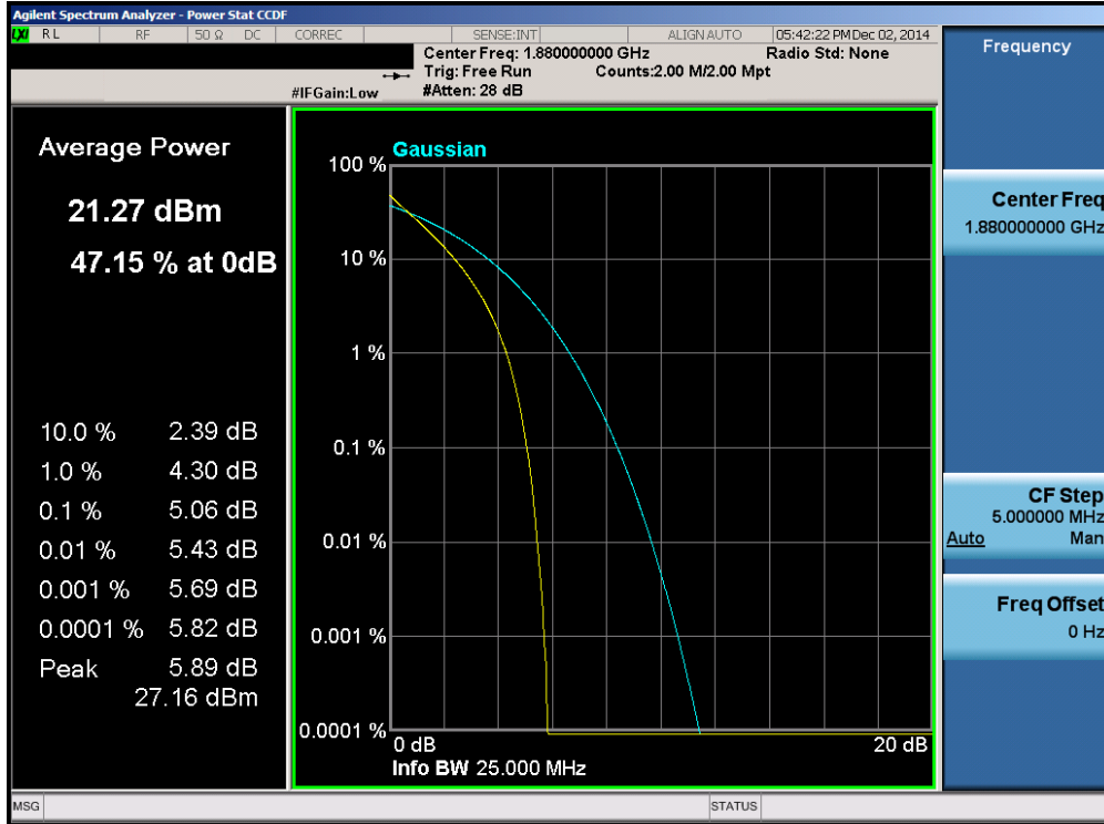
Plot 6-111. PAR Plot (Band 2 – 15.0MHz QPSK – RB Size 75)
