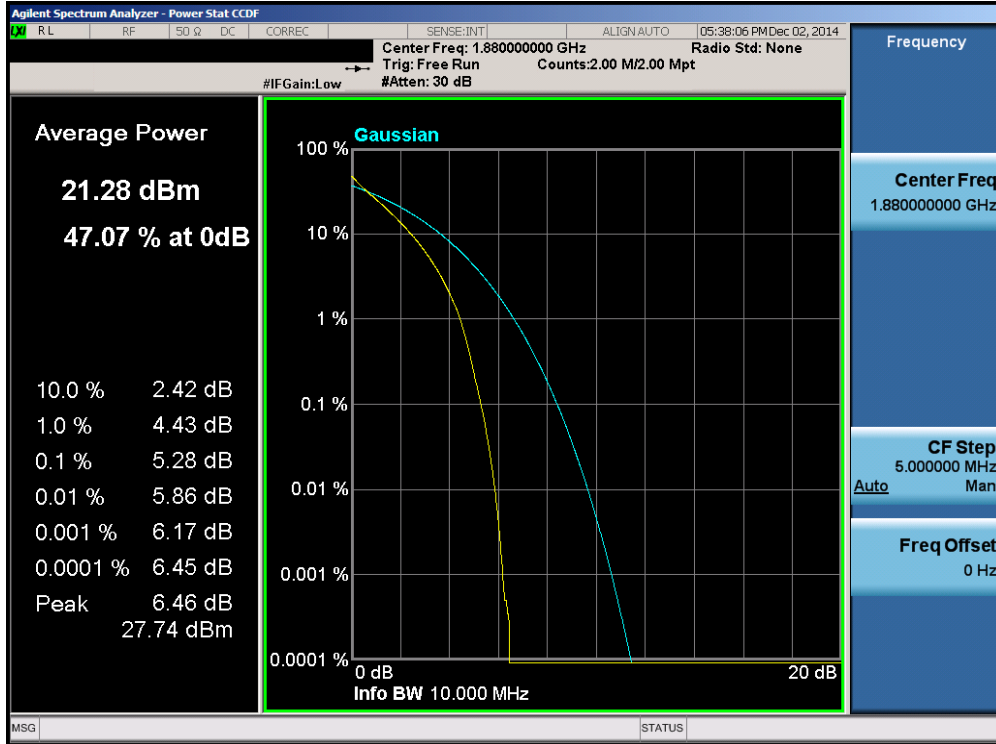
Plot 6-109. PAR Plot (Band 2 – 10.0MHz QPSK – RB Size 50)
