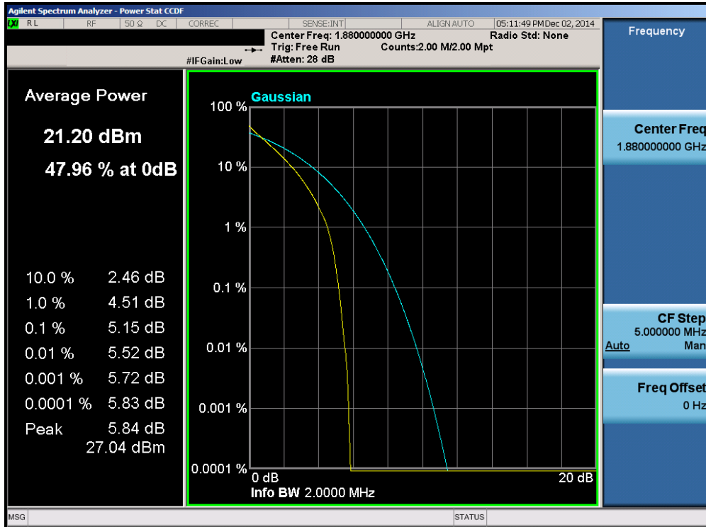
Plot 6-103. PAR Plot (Band 2 – 1.4MHz QPSK – RB Size 6)
