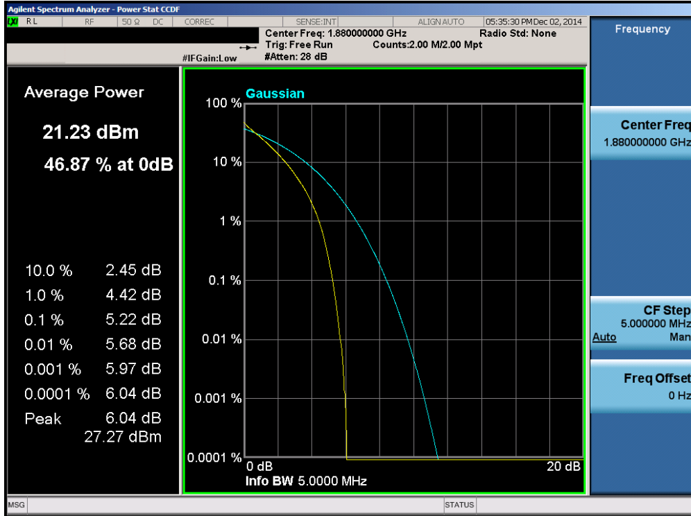
Plot 6-107. PAR Plot (Band 2 – 5.0MHz QPSK – RB Size 25)
