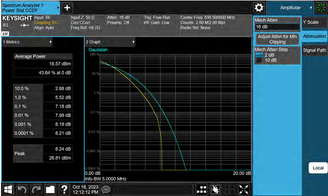
Sub6 n26. PAR Plot (5 M BW Ch.167300 256QAM_RB 25_0)
