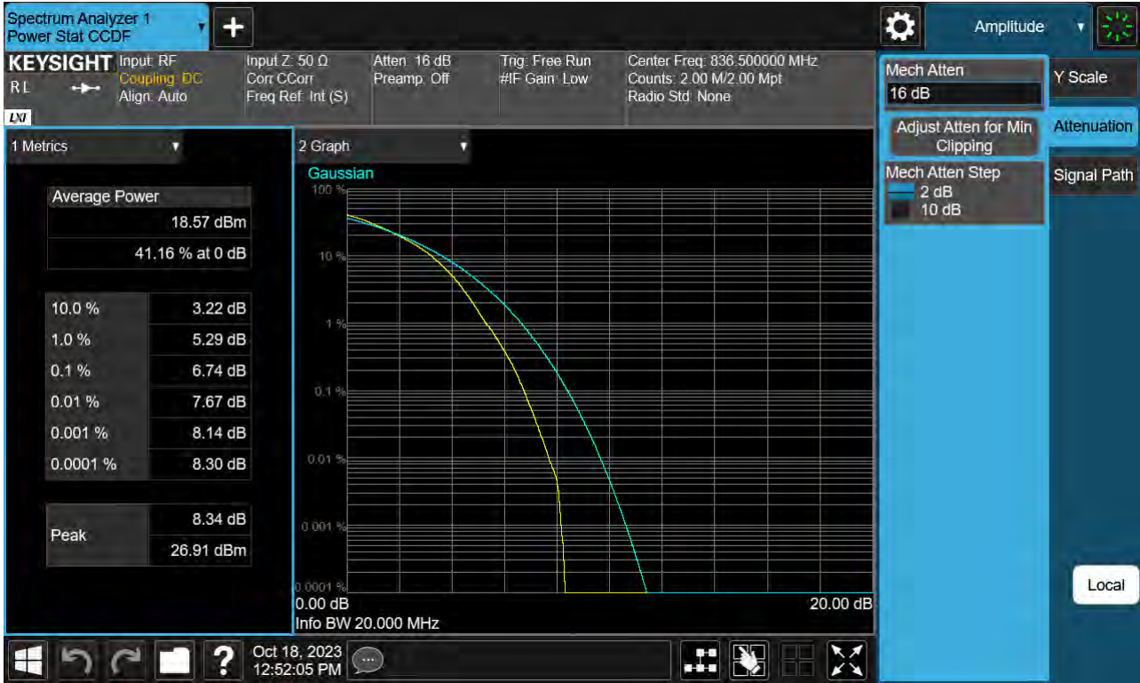
Sub6 n26. PAR Plot (20 M BW Ch.167300 256QAM RB 100_0)
