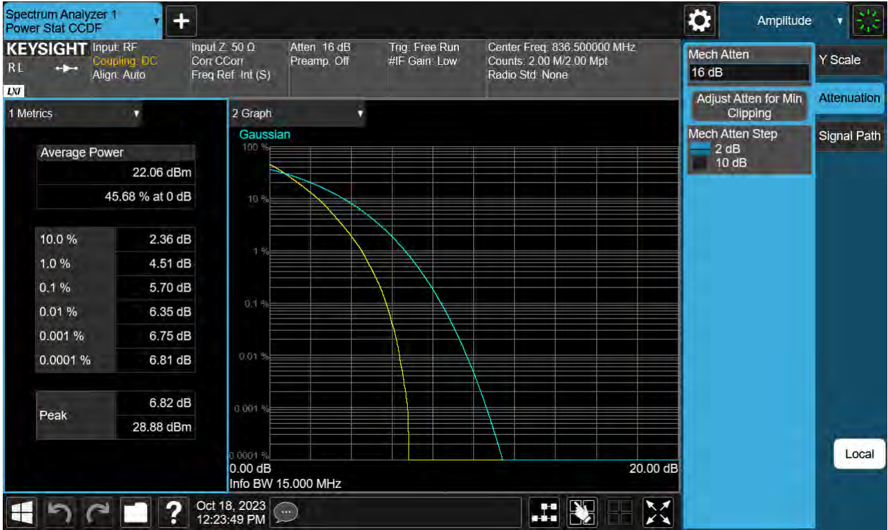
Sub6 n26. PAR Plot (15 M BW Ch.167300 QPSK RB 75_0)
