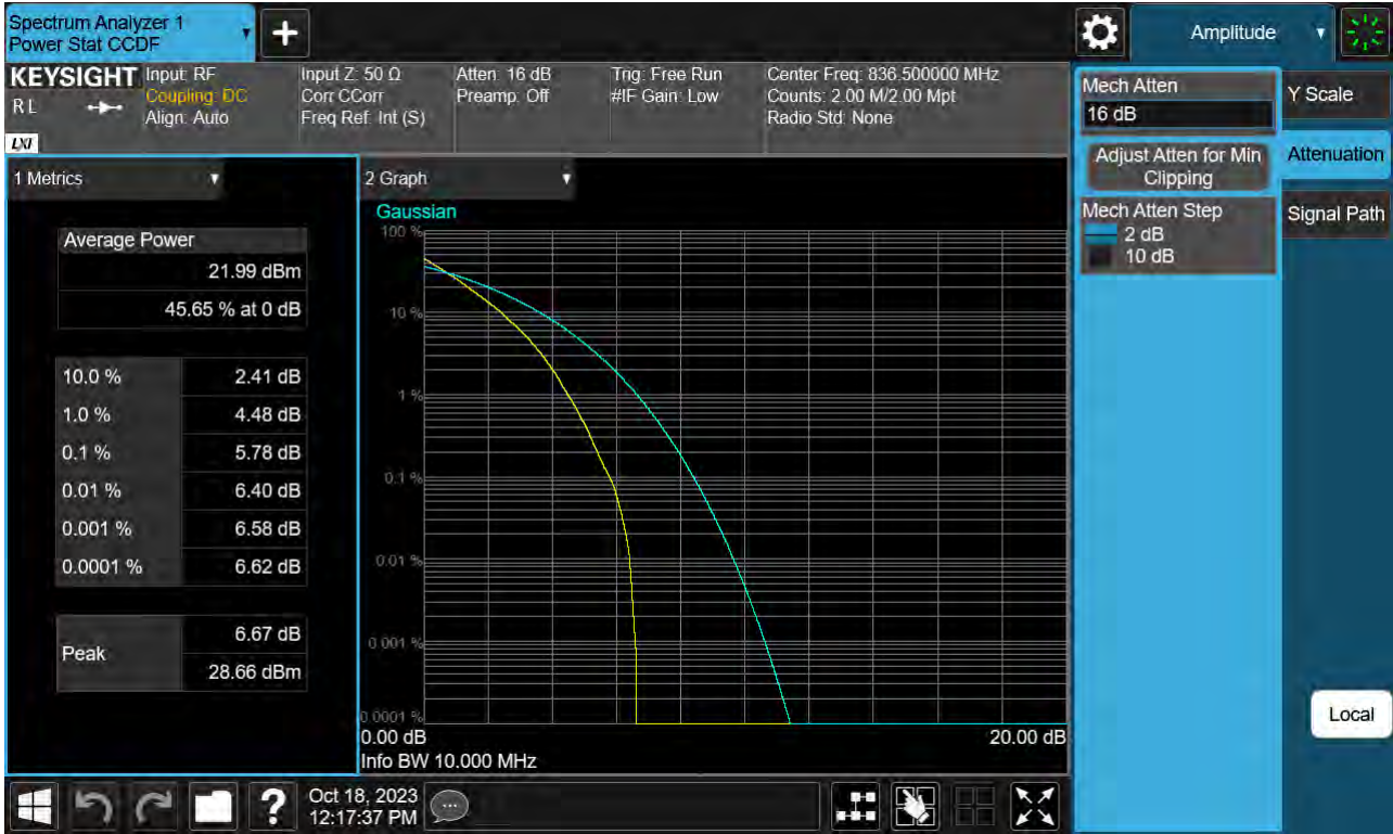
Sub6 n26. PAR Plot (10 M BW Ch.167300 QPSK_RB 50_0)
