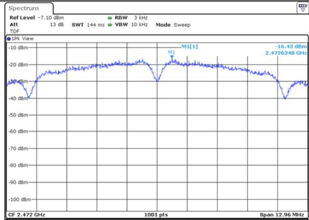
802.11b / 2 472 MHz
