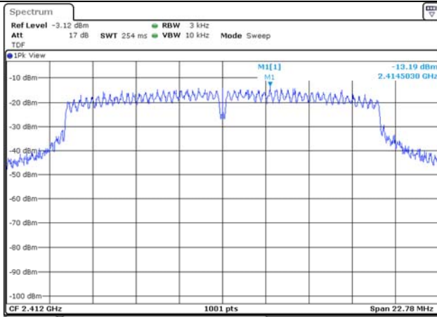
802.11g / 2 412 MHz
