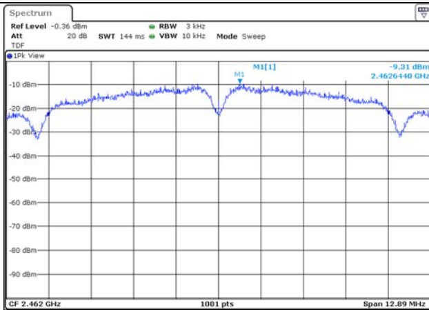
802.11b / 2 462 MHz
