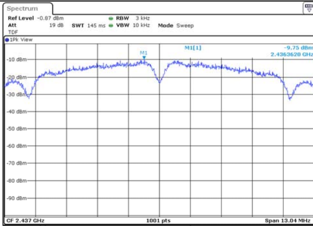
802.11b / 2 437 MHz
