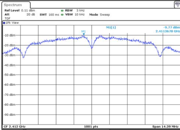
802.11b / 2 412 MHz
