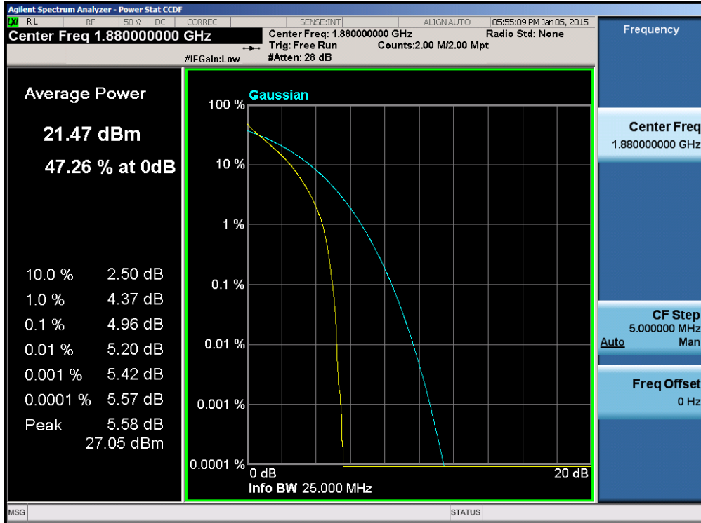
Plot 6-113. PAR Plot (Band 2 – 15.0MHz QPSK – RB Size 75)
