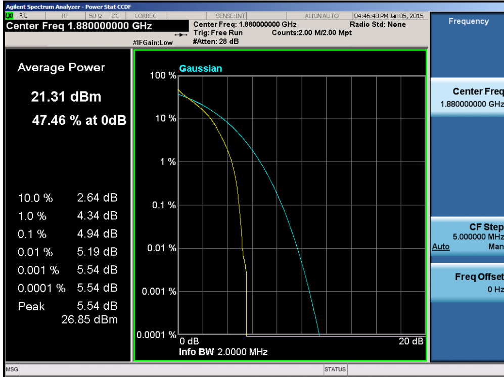
Plot 6-105. PAR Plot (Band 2 – 1.4MHz QPSK – RB Size 6)
