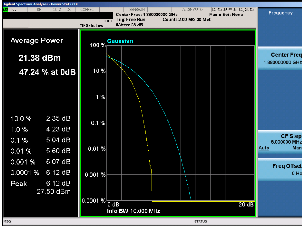
Plot 6-111. PAR Plot (Band 2 – 10.0MHz QPSK – RB Size 50)
