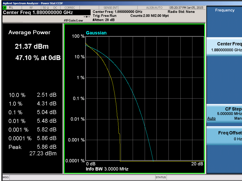
Plot 6-107. PAR Plot (Band 2 – 3.0MHz QPSK – RB Size 15)
