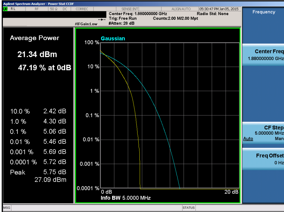
Plot 6-109. PAR Plot (Band 2 – 5.0MHz QPSK – RB Size 25)
