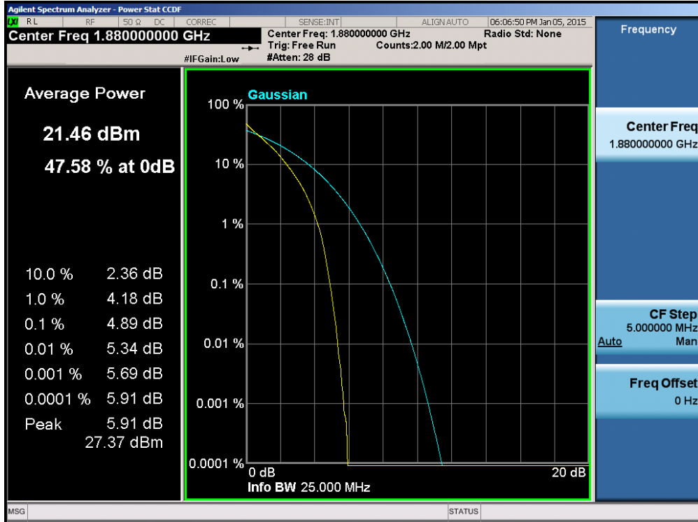
Plot 6-115. PAR Plot (Band 2 – 20.0MHz QPSK – RB Size 100)
