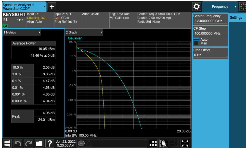
Plot 7-423. PAR Plot (NR Band n77 (C-Band) - 100MHz \pi/2 BPSK - Full RB - Antenna G)
