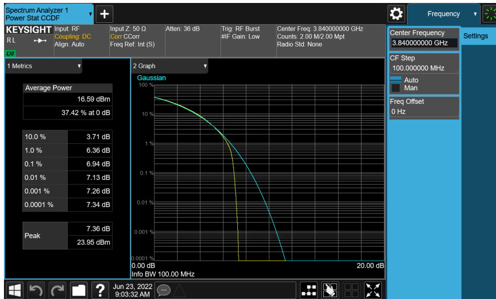
Plot 7-424. PAR Plot (NR Band n77 (C-Band) - 100MHz QPSK - Full RB - Antenna G)
