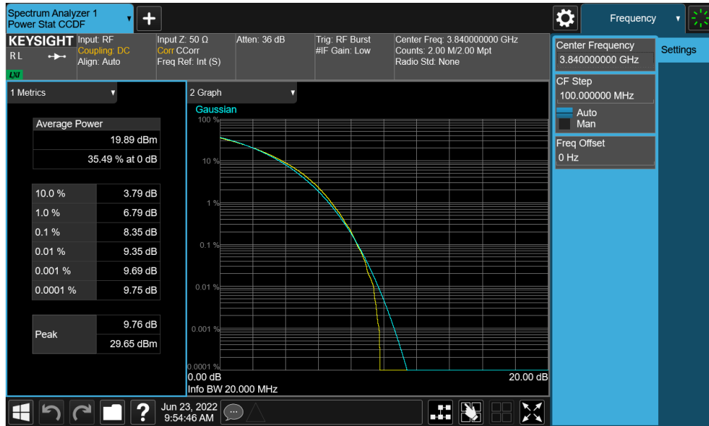
Plot 7-413. PAR Plot (NR Band n77 (C-Band) - 20MHz 256-QAM - Full RB - Antenna E)
