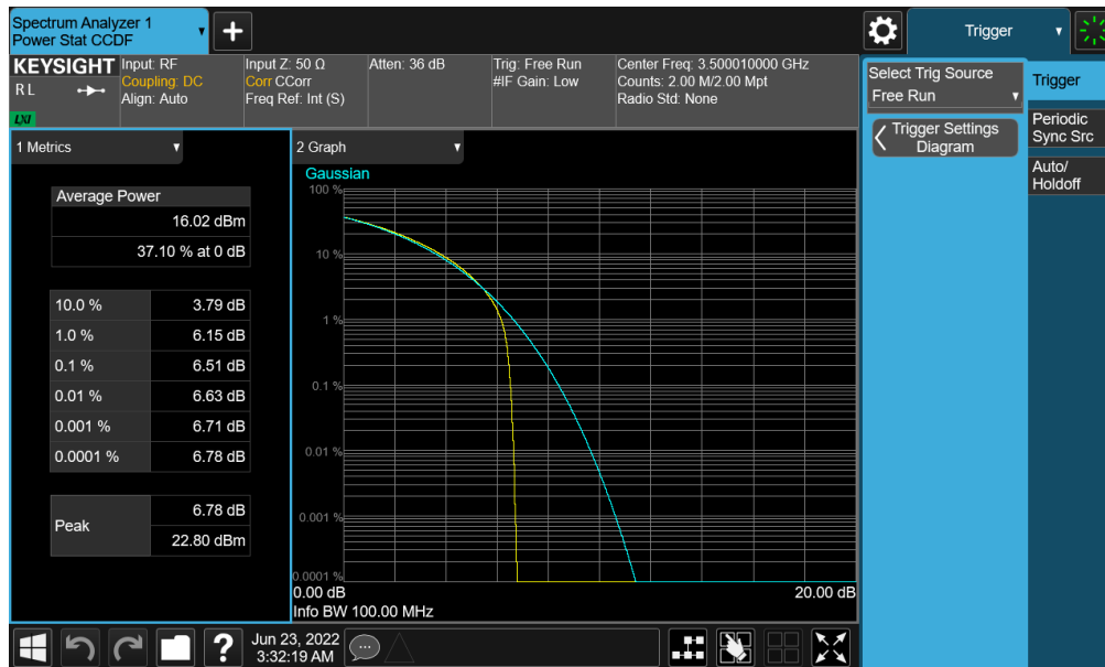
Plot 7-427. PAR Plot (NR Band n77 (DoD) - 100MHz QPSK - Full RB – Antenna D)
