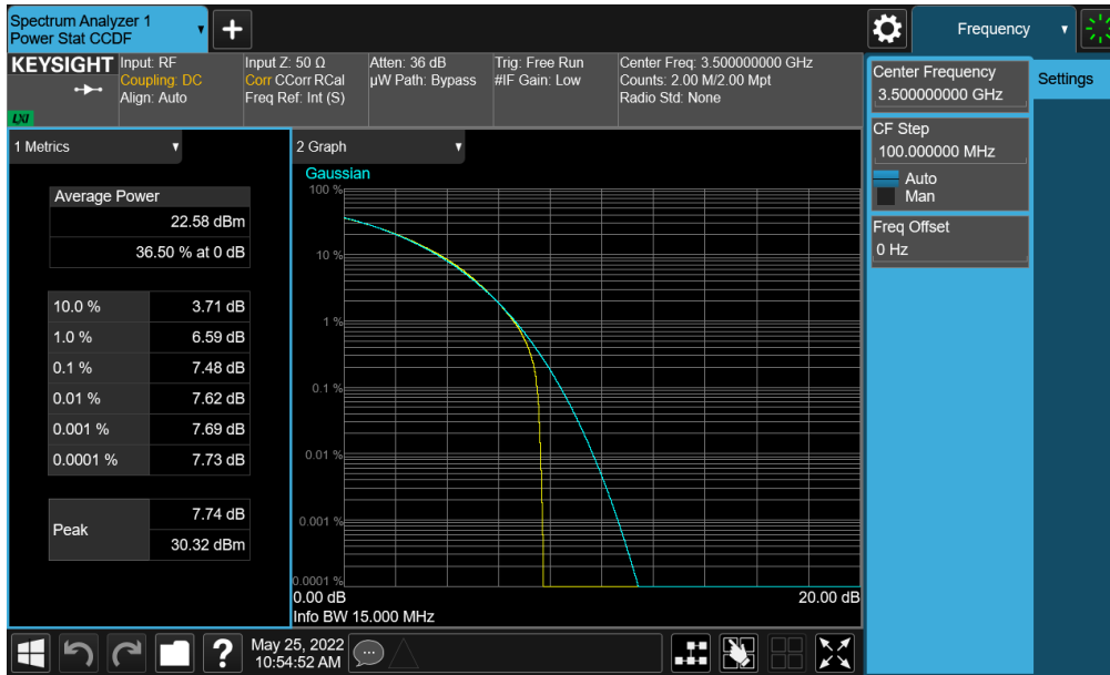
Plot 7-389. PAR Plot (NR Band n77 (DoD) - 15MHz CP-OFDM QPSK - Full RB - Ant F)
