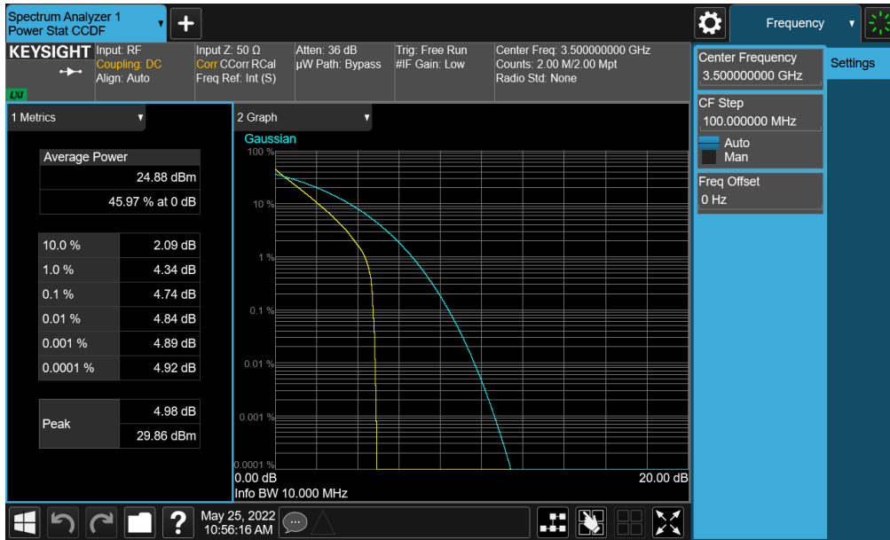
Plot 7-391. PAR Plot (NR Band n77 (DoD) - 10MHz DFT-s-OFDM BPSK - Full RB - Ant F)
