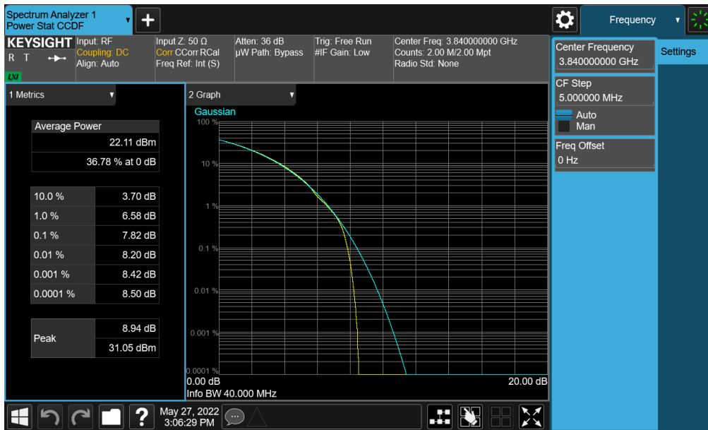
Plot 7-341. PAR Plot (NR Band n77 (C-Band) - 40MHz CP-OFDM QPSK - Full RB - Ant E)
