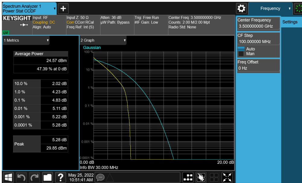
Plot 7-382. PAR Plot (NR Band n77 (DoD) - 30MHz DFT-s-OFDM BPSK - Full RB - Ant F)
