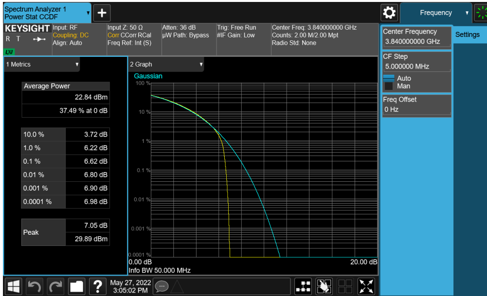
Plot 7-338. PAR Plot (NR Band n77 (C-Band) - 50MHz CP-OFDM QPSK - Full RB - Ant E)
