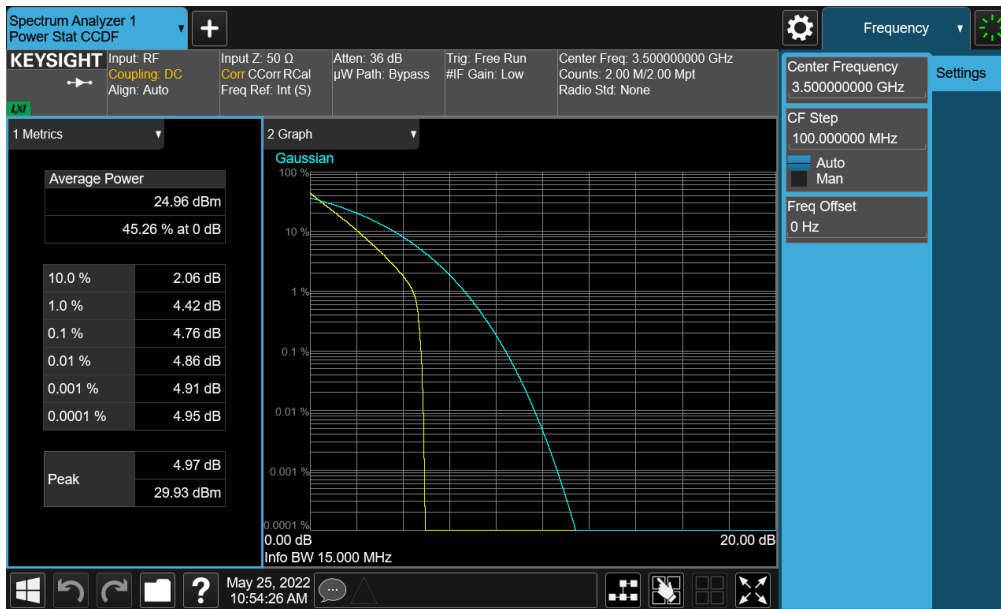
Plot 7-388. PAR Plot (NR Band n77 (DoD) - 15MHz DFT-s-OFDM BPSK - Full RB - Ant F)
