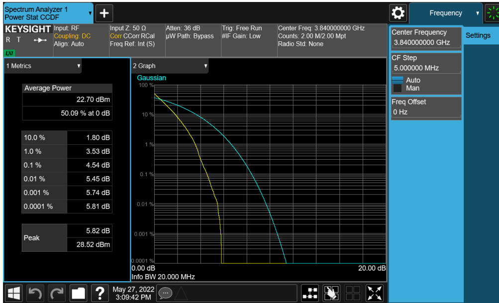
Plot 7-346. PAR Plot (NR Band n77 (C-Band) - 20MHz DFT-s-OFDM BPSK - Full RB - Ant E)
