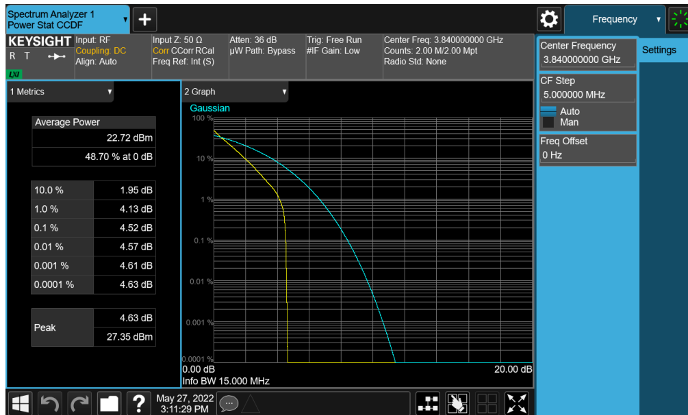
Plot 7-349. PAR Plot (NR Band n77 (C-Band) - 15MHz DFT-s-OFDM BPSK - Full RB - Ant E)
