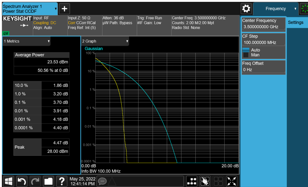
Plot 7-394. PAR Plot (NR Band n77 (DoD) - 100MHz DFT-s-OFDM BPSK - Full RB - Ant E)
