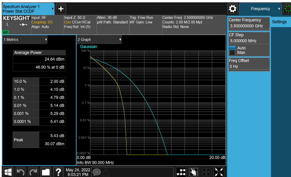
Plot 7-364. PAR Plot (NR Band n77 (DoD) - 90MHz DFT-s-OFDM BPSK - Full RB - Ant F)
