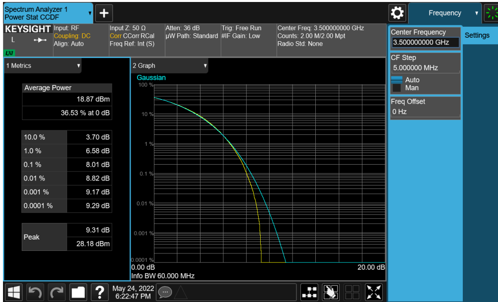
Plot 7-375. PAR Plot (NR Band n77 (DoD) - 60MHz CP-OFDM 256-QAM - Full RB - Ant F)
