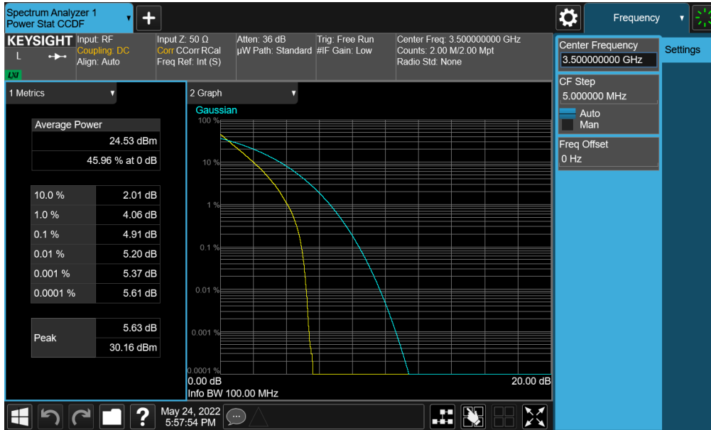
Plot 7-361. PAR Plot (NR Band n77 (DoD) - 100MHz DFT-s-OFDM BPSK - Full RB - Ant F)
