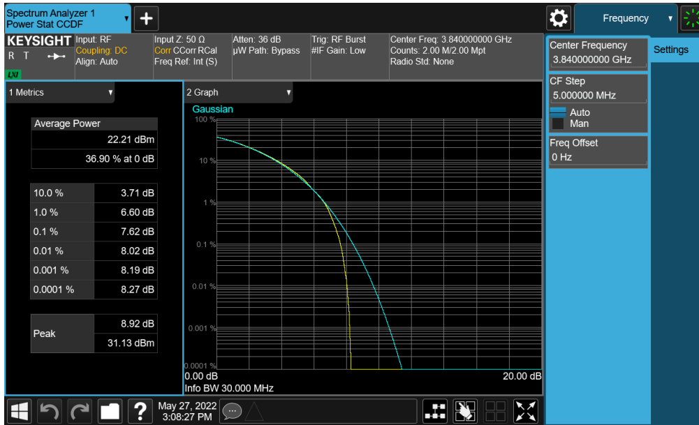
Plot 7-344. PAR Plot (NR Band n77 (C-Band) - 30MHz CP-OFDM QPSK - Full RB - Ant E)
