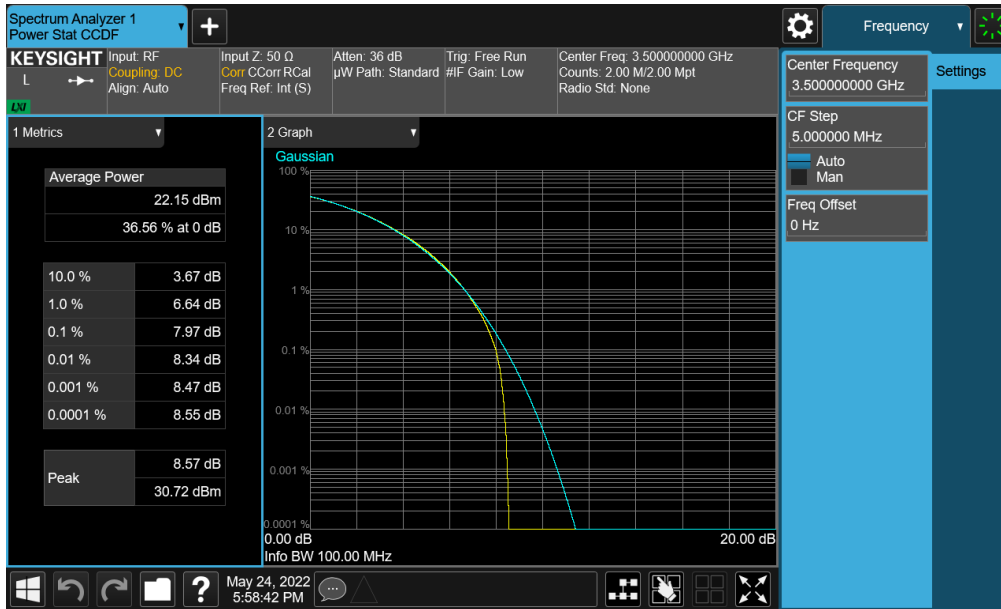
Plot 7-362. PAR Plot (NR Band n77 (DoD) - 100MHz CP-OFDM QPSK - Full RB - Ant F)
