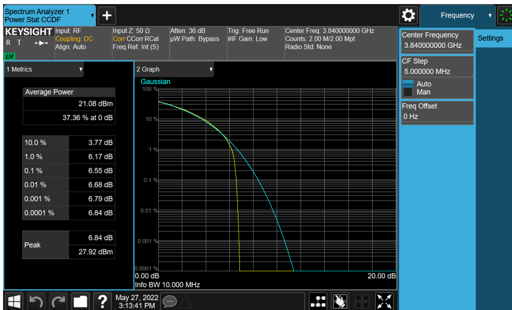
Plot 7-353. PAR Plot (NR Band n77 (C-Band) - 10MHz CP-OFDM QPSK - Full RB - Ant E)
