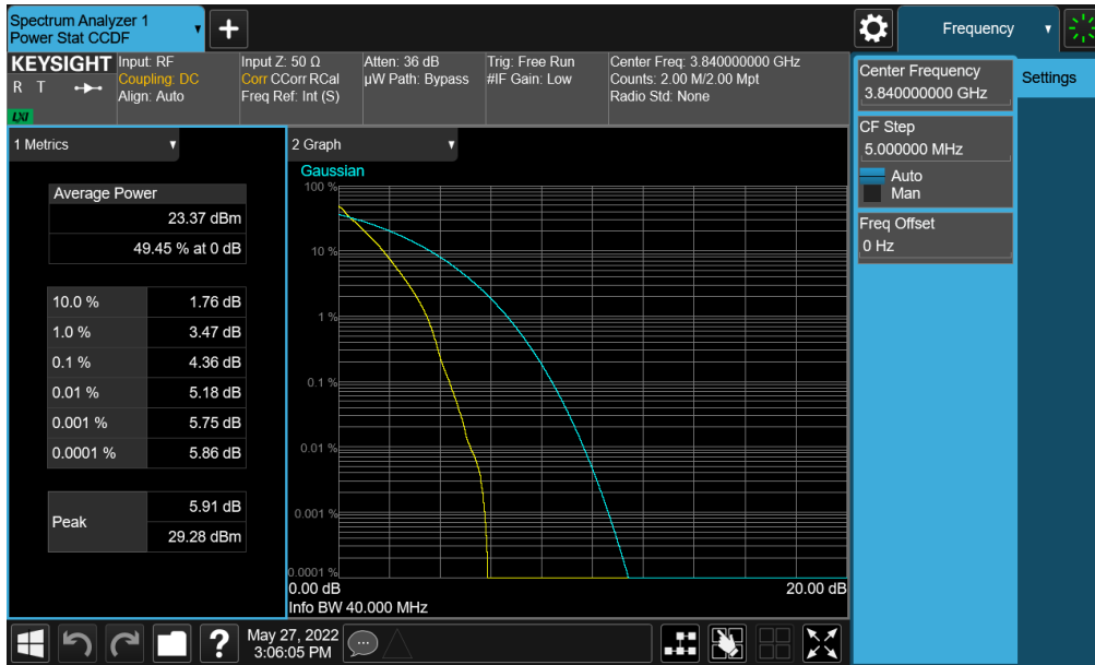
Plot 7-340. PAR Plot (NR Band n77 (C-Band) - 40MHz DFT-s-OFDM BPSK - Full RB - Ant E)
