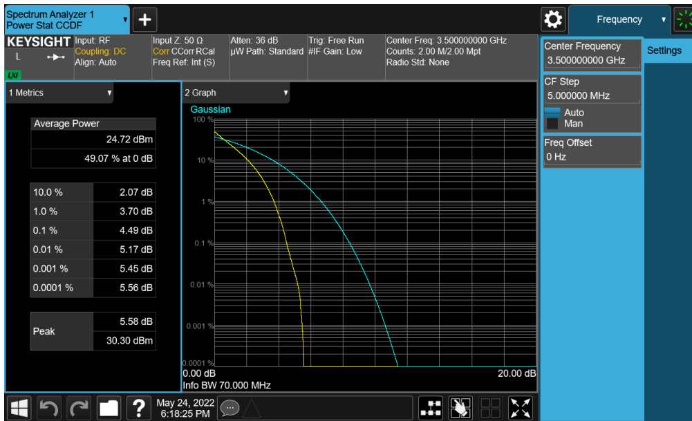
Plot 7-370. PAR Plot (NR Band n77 (DoD) - 70MHz DFT-s-OFDM BPSK - Full RB - Ant F)
