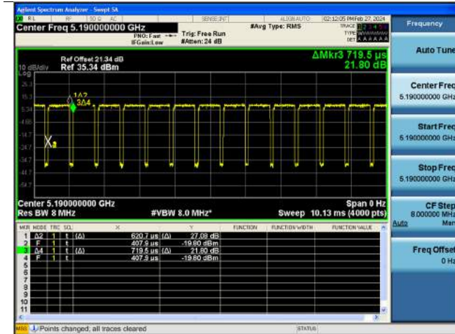
802.11n(HT40)
