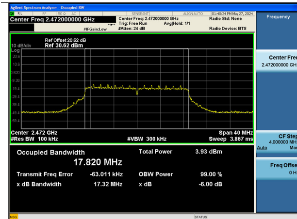
802.11n_HT20-CH 13
