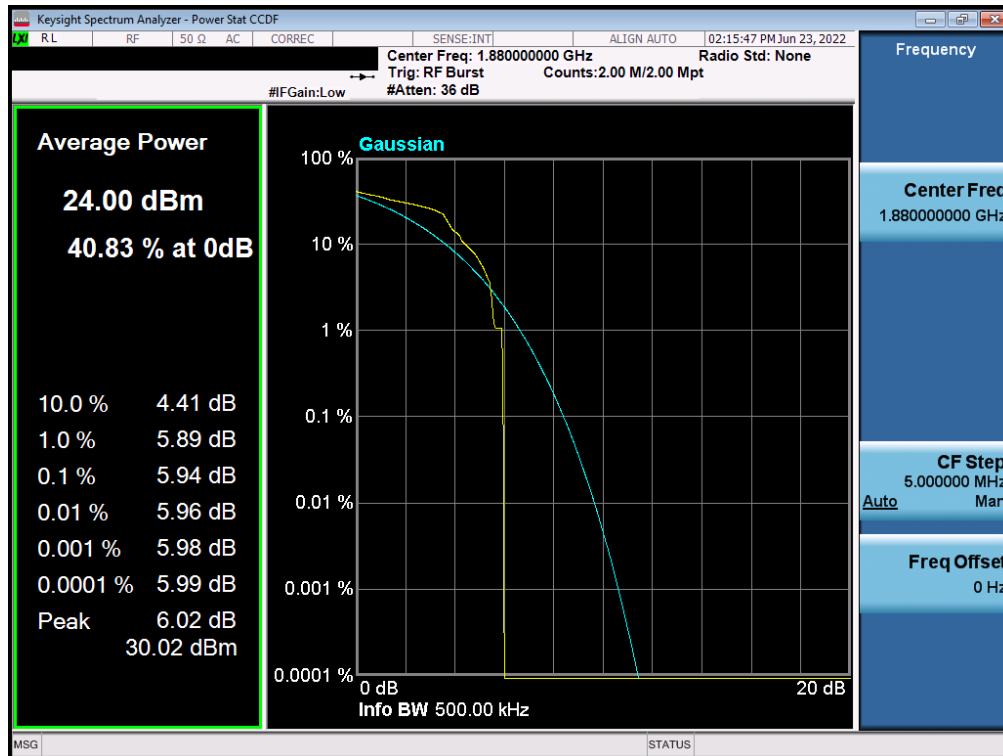
Plot 7-2. PAR Plot (EDGE, Ch. 661)
