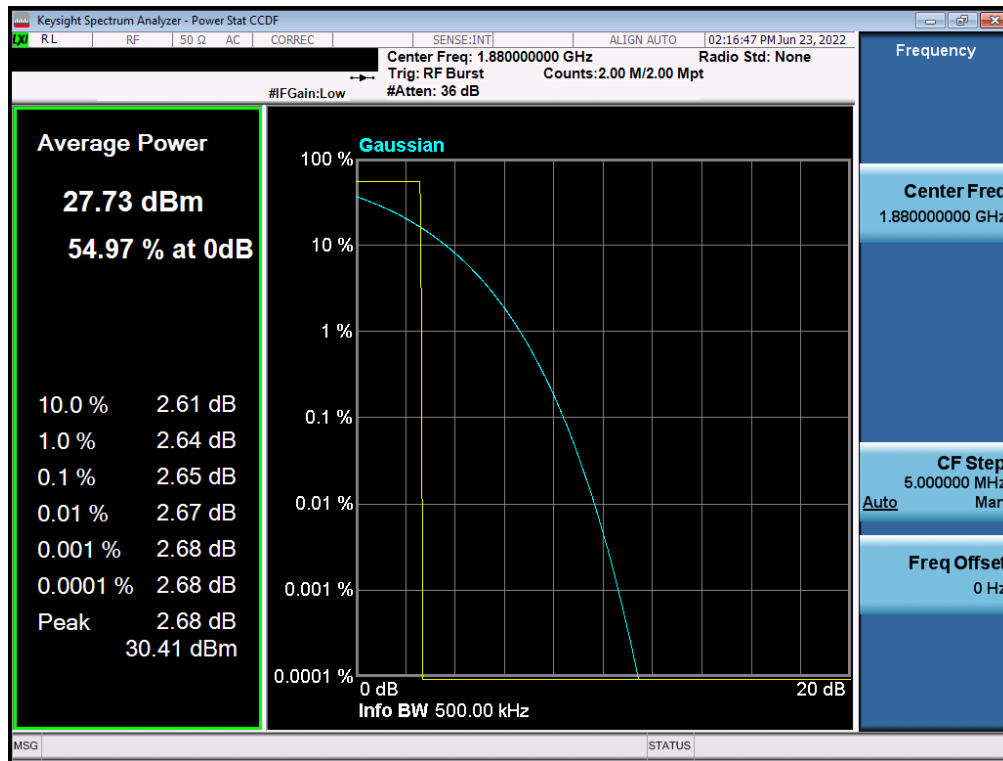
Plot 7-1. PAR Plot (GPRS, Ch. 661)
