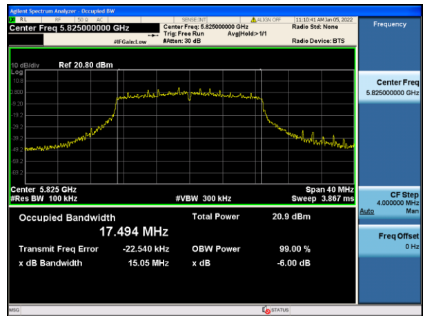
802.11ac(VHT20) (CH.165)
