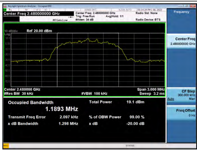
8DPSK : (CH.78)
