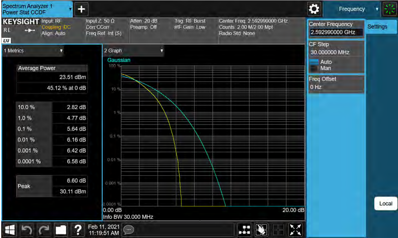
Sub6 n41. PAR Plot (30M BW_Ch.518598_64QAM)
