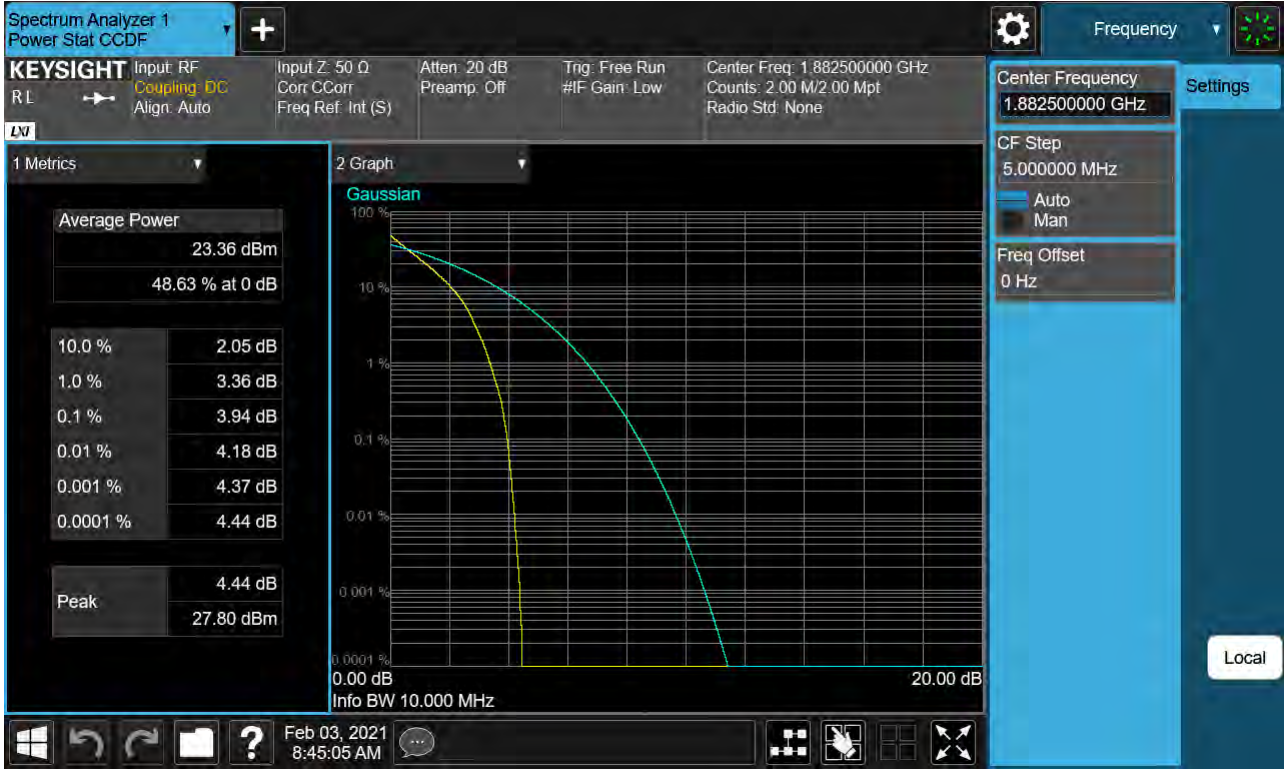
Sub6 n25. PAR Plot (10M BW Ch.376500 BPSK RB 50_0)
