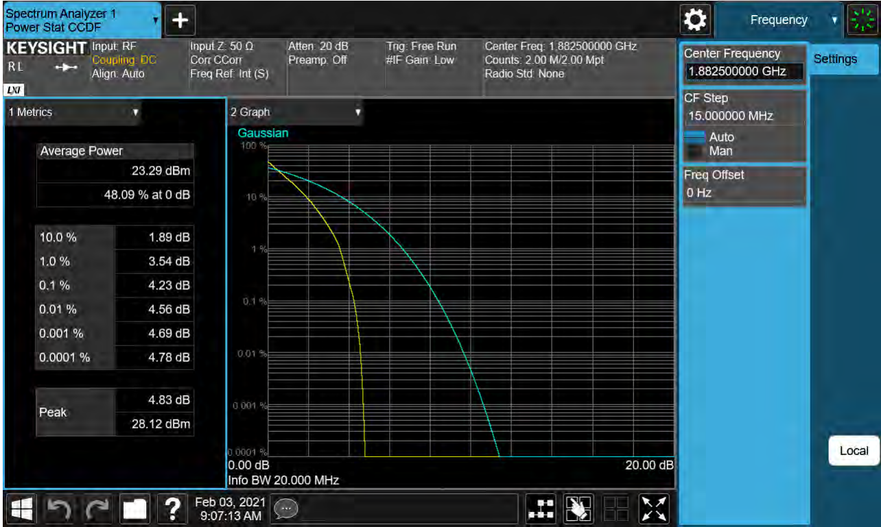
Sub6 n25. PAR Plot (20M BW Ch.376500 BPSK RB 100_0)
