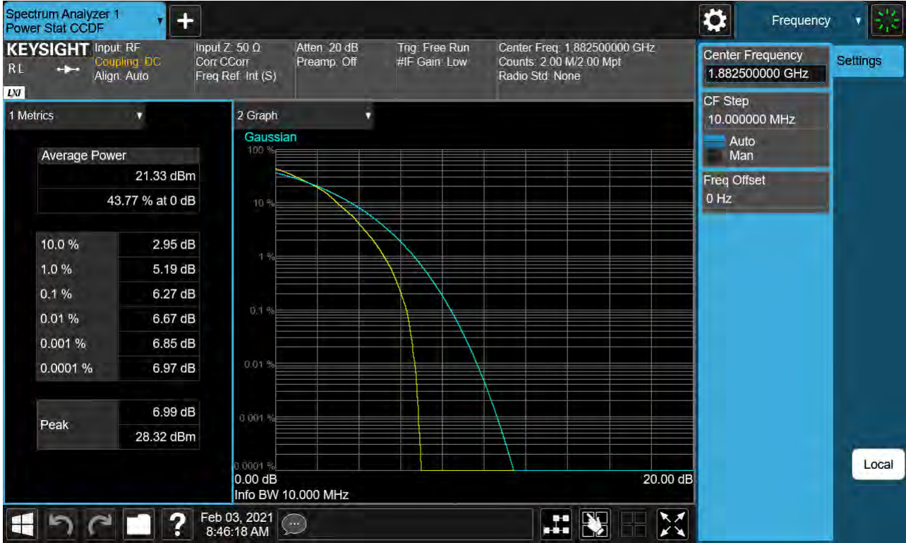
Sub6 n25. PAR Plot (10M BW Ch.376500 64QAM RB 50_0)
