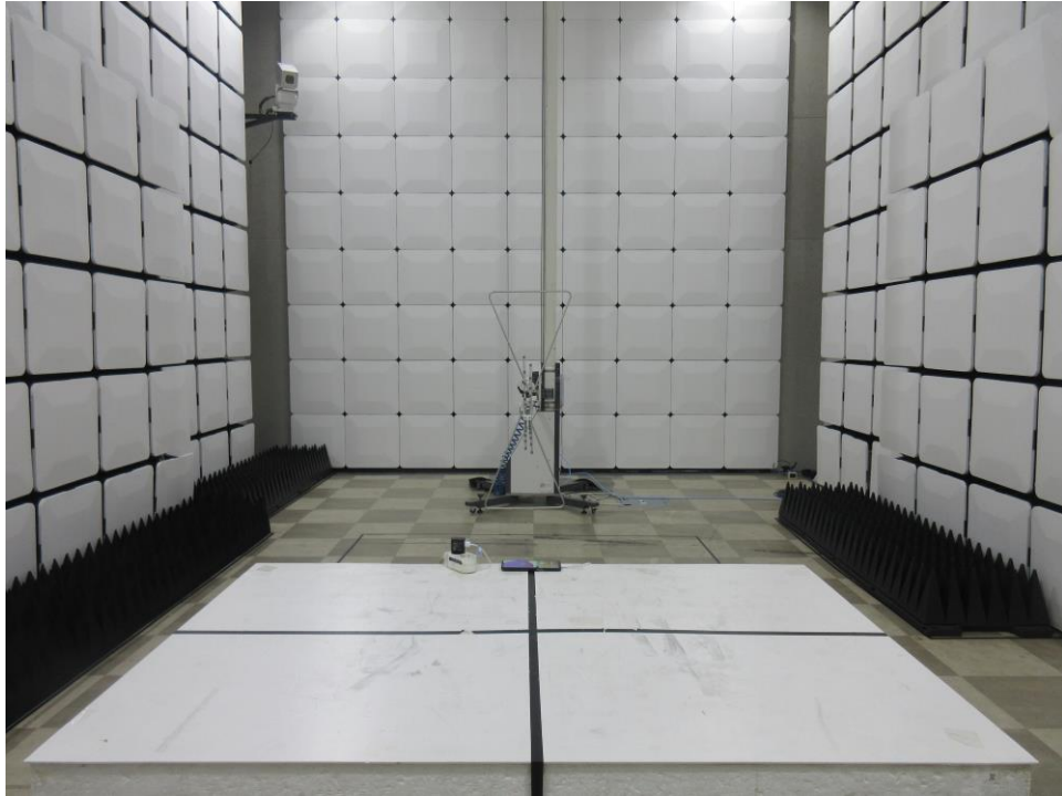
[EUT+TA (15 W)]
