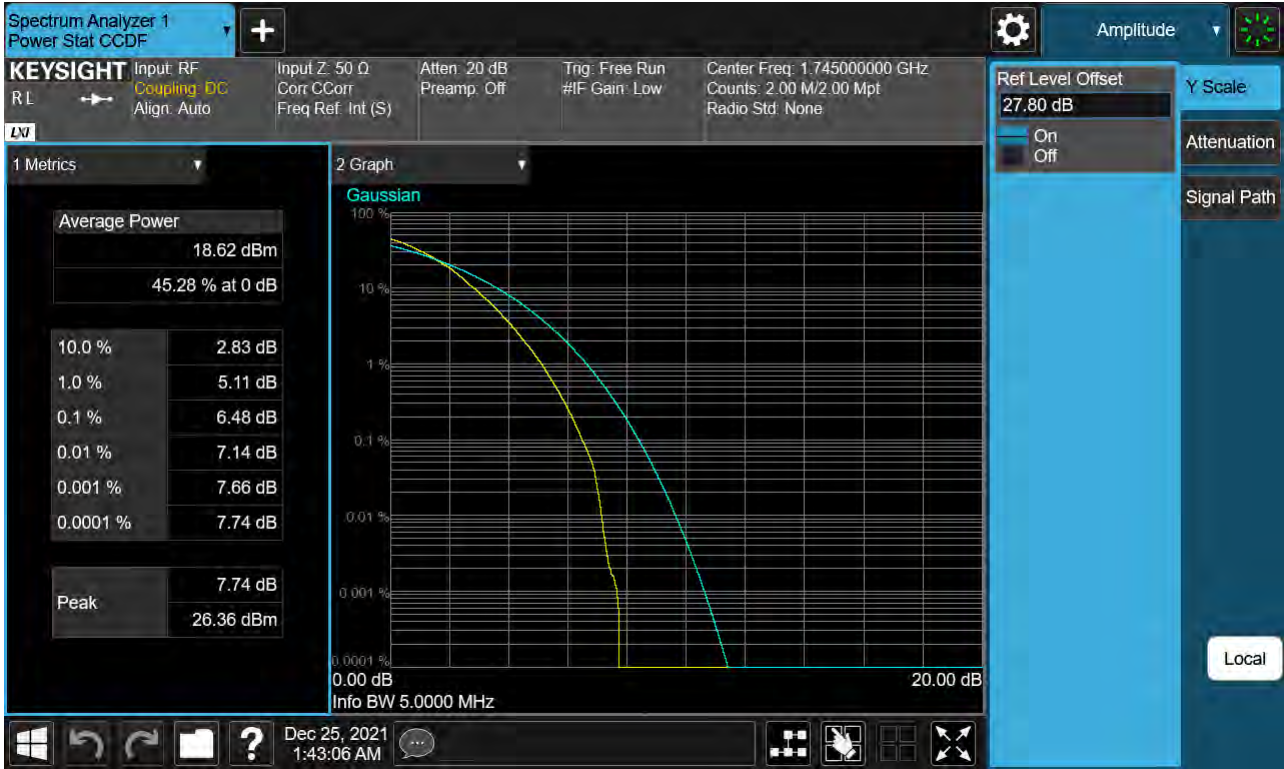
Sub6 n66. PAR Plot (5 M BW_Ch.349000_256QAM_Full RB)
