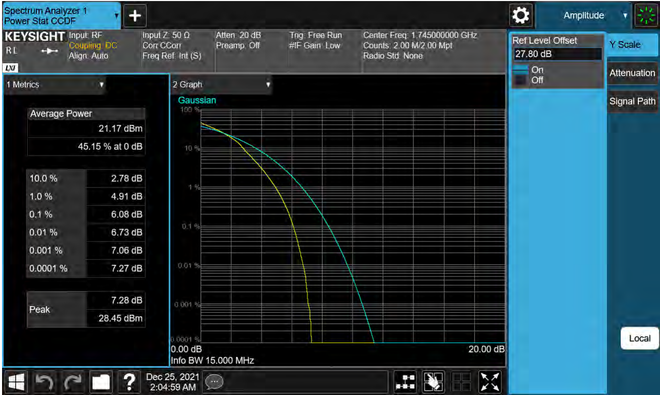
Sub6 n66. PAR Plot (15 M BW_Ch.349000_16QAM_Full RB)
