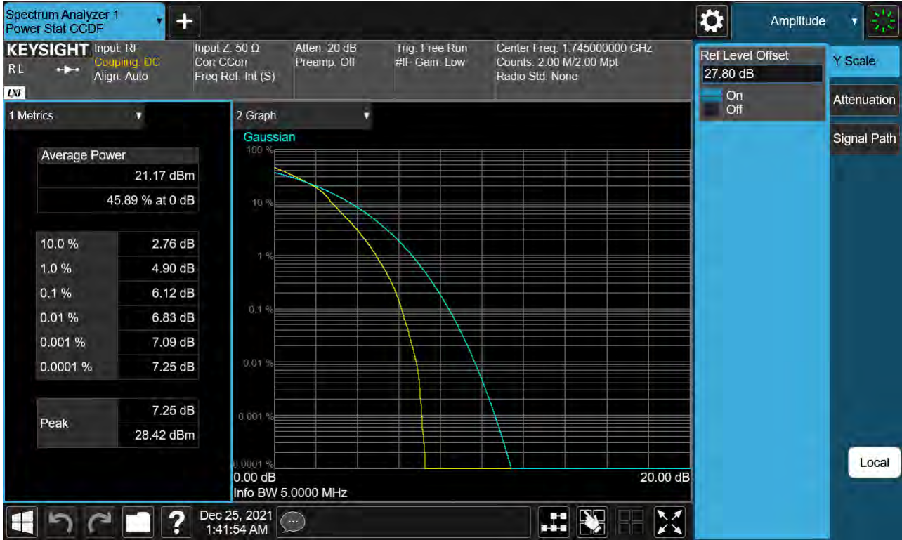
Sub6 n66. PAR Plot (5 M BW_Ch.349000_16QAM_Full RB)
