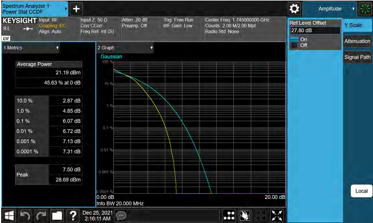
Sub6 n66. PAR Plot (20 M BW_Ch.349000_16QAM_Full RB)
