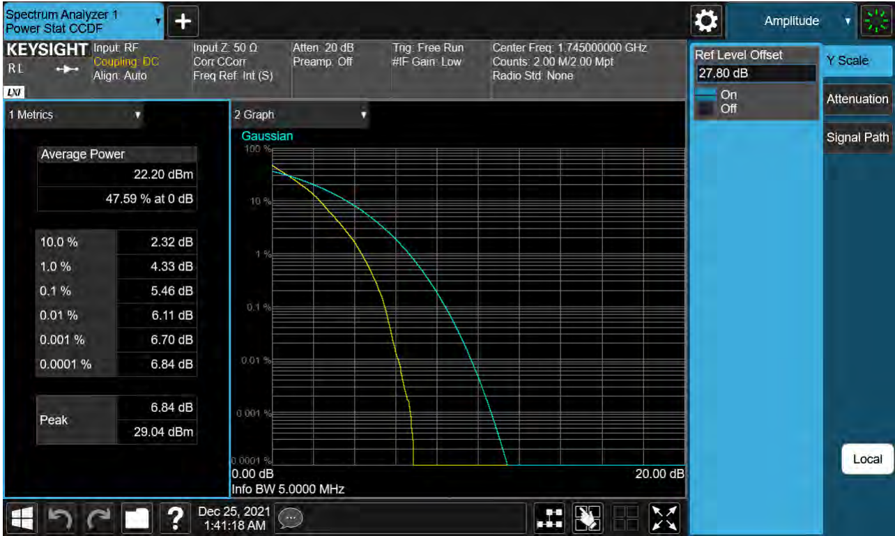
Sub6 n66. PAR Plot (5 M BW_Ch.349000_QPSK_Full RB)
