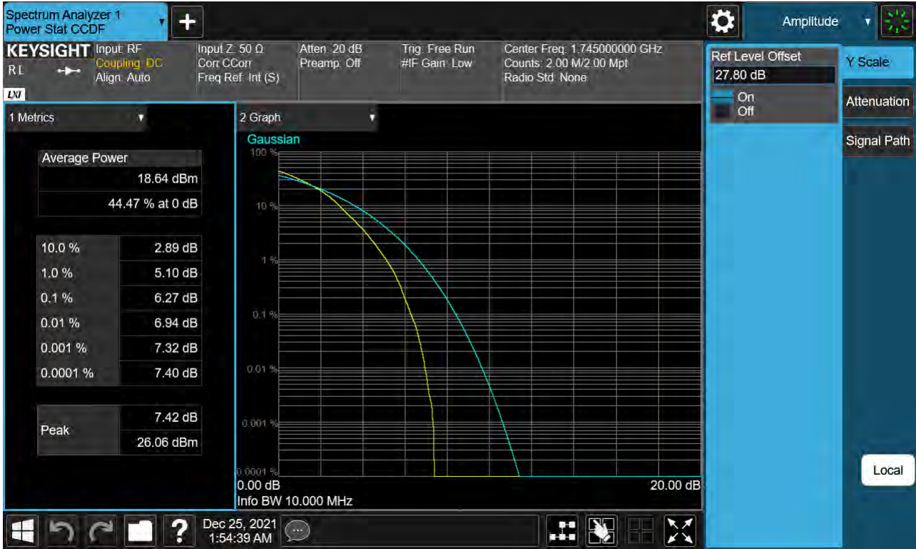
Sub6 n66. PAR Plot (10 M BW_Ch.349000_256QAM_Full RB)
