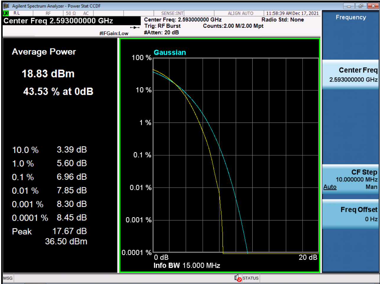
PAR Plot (15 M BW_Ch.40620_256QAM_RB75_0) (POWER CLASS 3)
