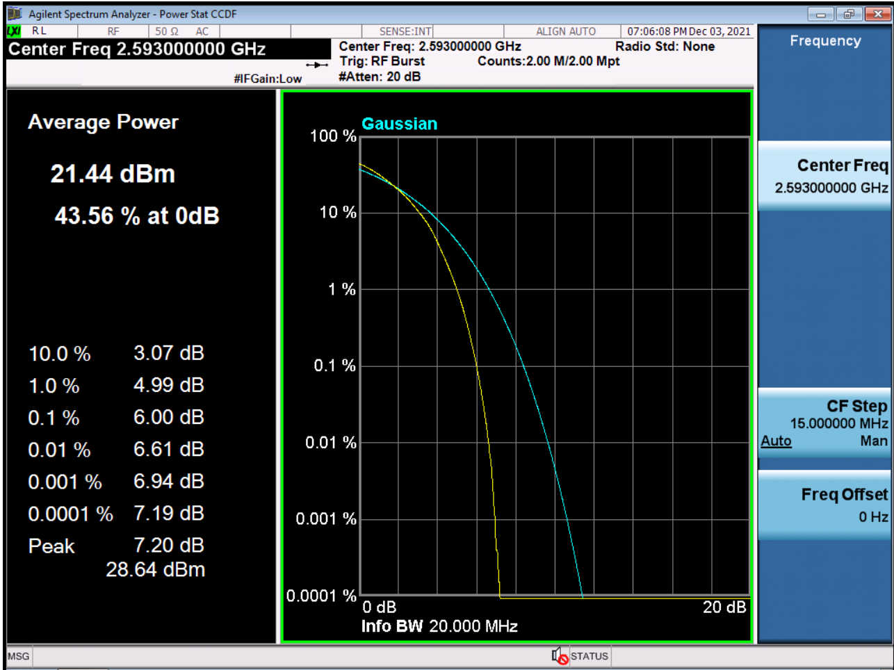
PAR Plot (20 M BW_Ch.40620_64QAM_RB100_0) (POWER CLASS 3)
