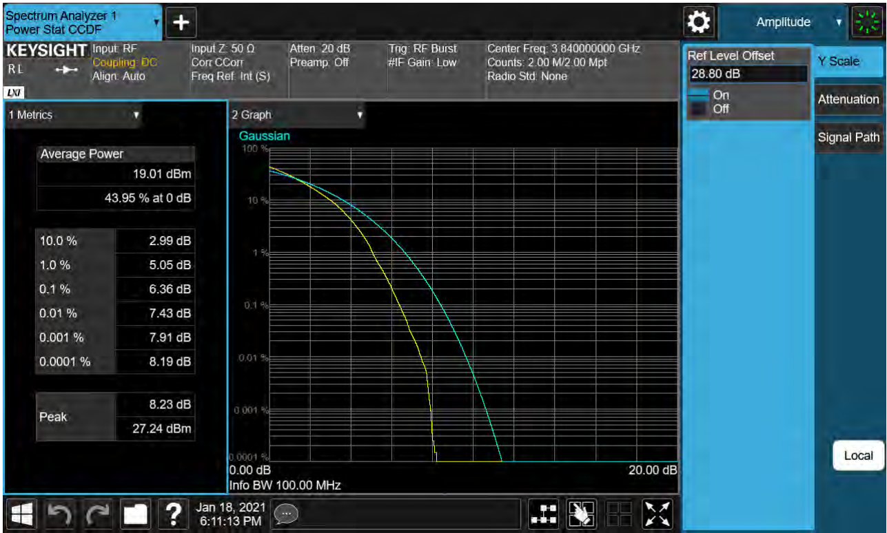
Sub6 n77. PAR Plot (100M BW_Ch.656000_256QAM)
